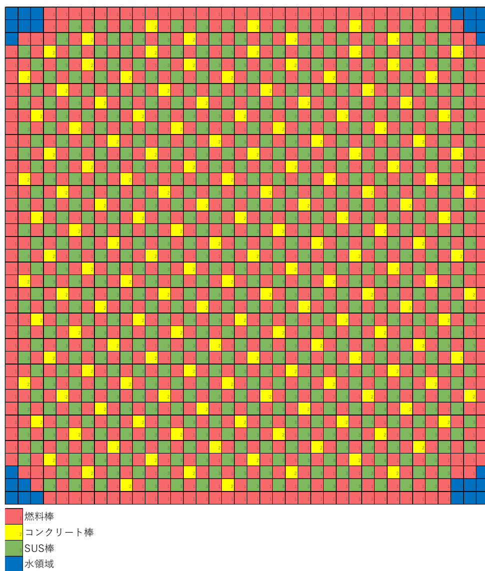
図 2 燃料棒 : コンクリート棒 : SUS 棒 : 水領域比率 800:160:496:26(39×38)の炉心構成例
