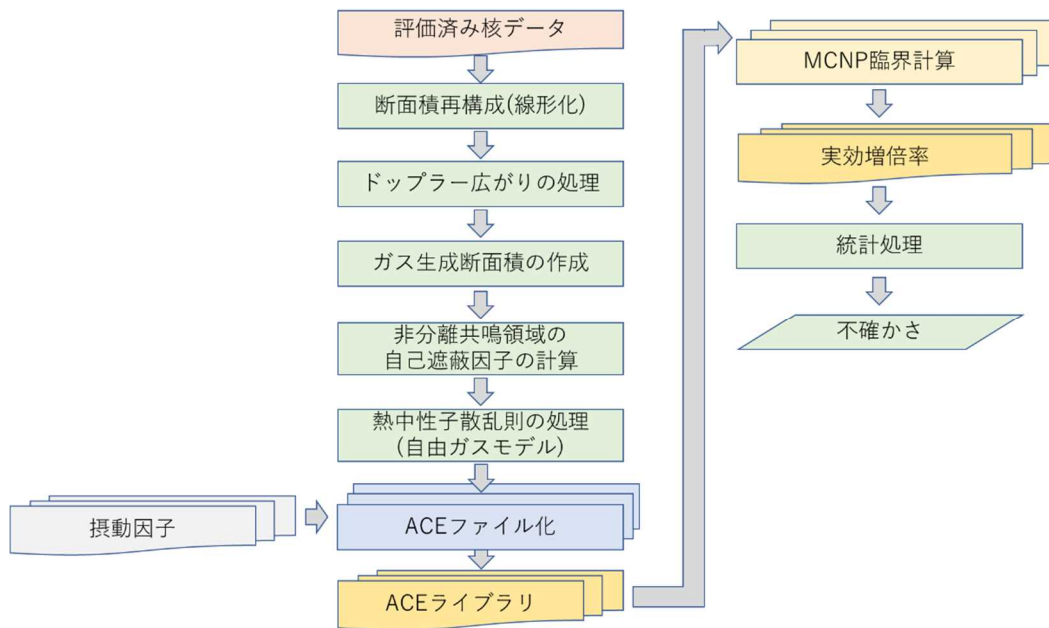
図4 FRENDDYコードを用いた断面積処理の流れ
