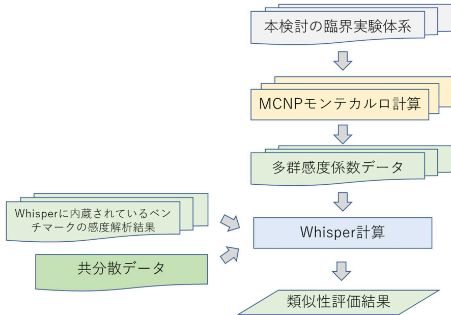
図3 Whisper1.1 を用いた類似性評価の流れ
