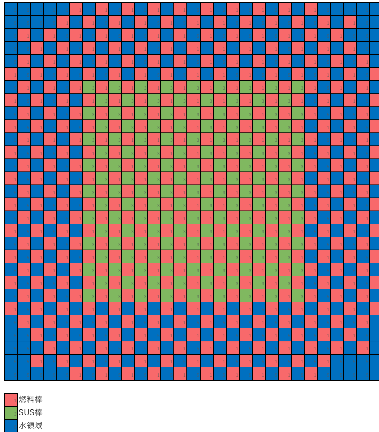
図1 燃料棒：コンクリート棒：SUS棒：水領域比率 400:0:145:296(29×29)の炉心構成例
