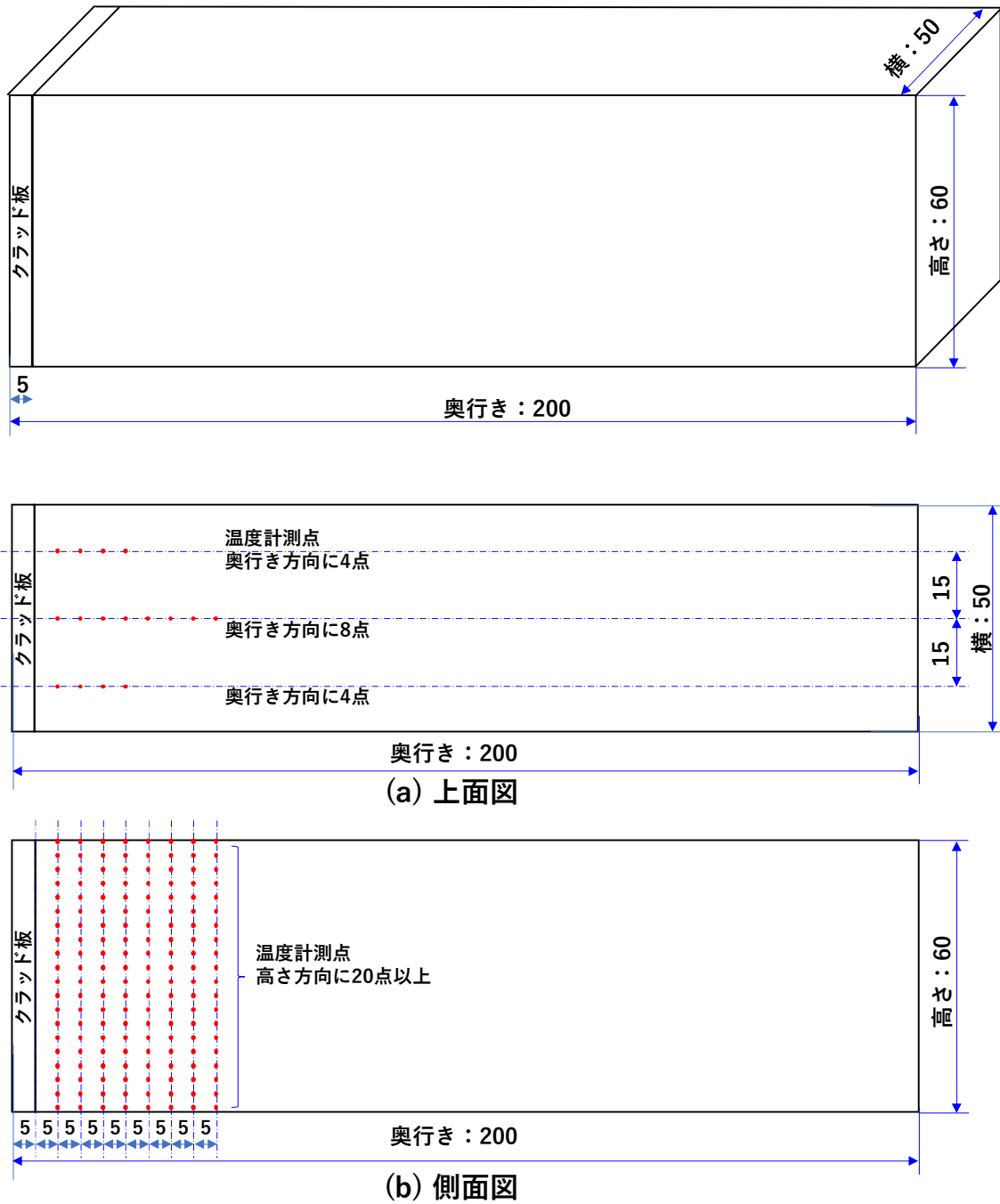
図1 クラッド鋼材の概念図
