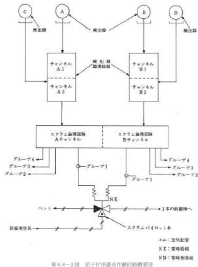
第6.6-3図 原子炉保護系作動回路概図
