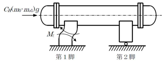
図5 長手方向荷重により 胴が受ける局部モーメント
