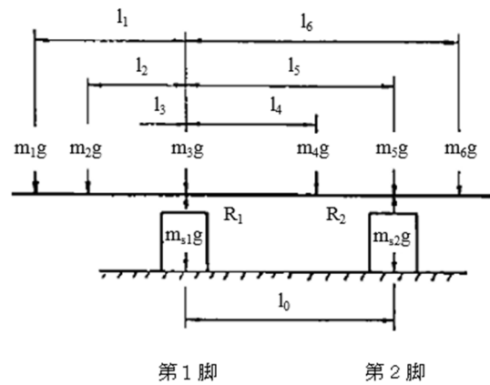
図3 荷重状態
