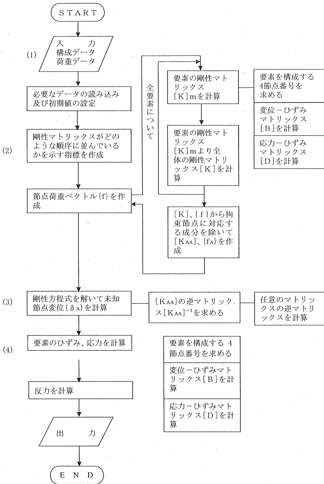
(ロ) - 第 A. 127 図 解析フロー
