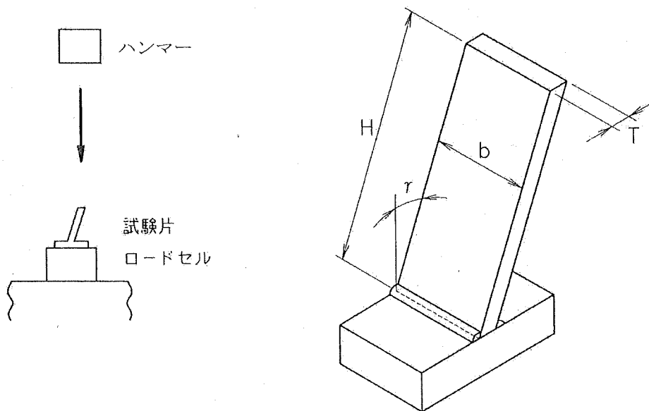
(ロ) - 第 A. 139 図 フィンの解析モデル
