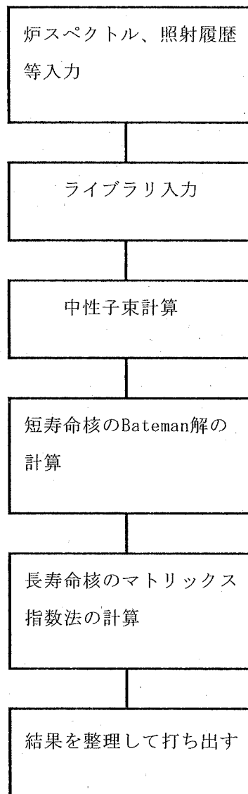
(ロ) - 第 D. 19 図 ORIGEN コード概略計算フロー
