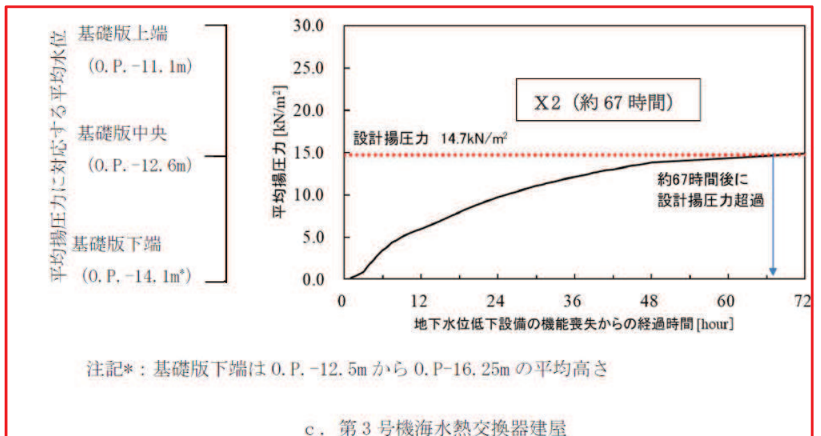
図6-2 地下水位低下設備機能喪失後の到達時間 (X1 及び X2)
