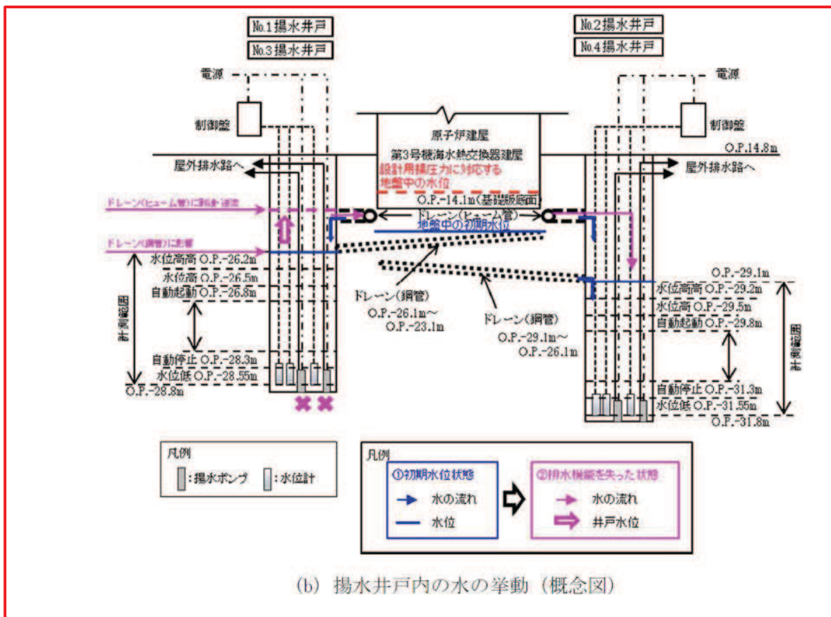
図 7-1 揚水ポンプが 1 系列動作不能となった場合の地下水位の挙動について
