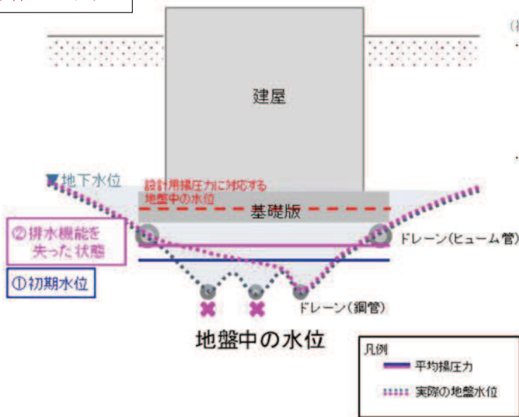
(a) 地盤中の地下水の挙動 (概念図)
