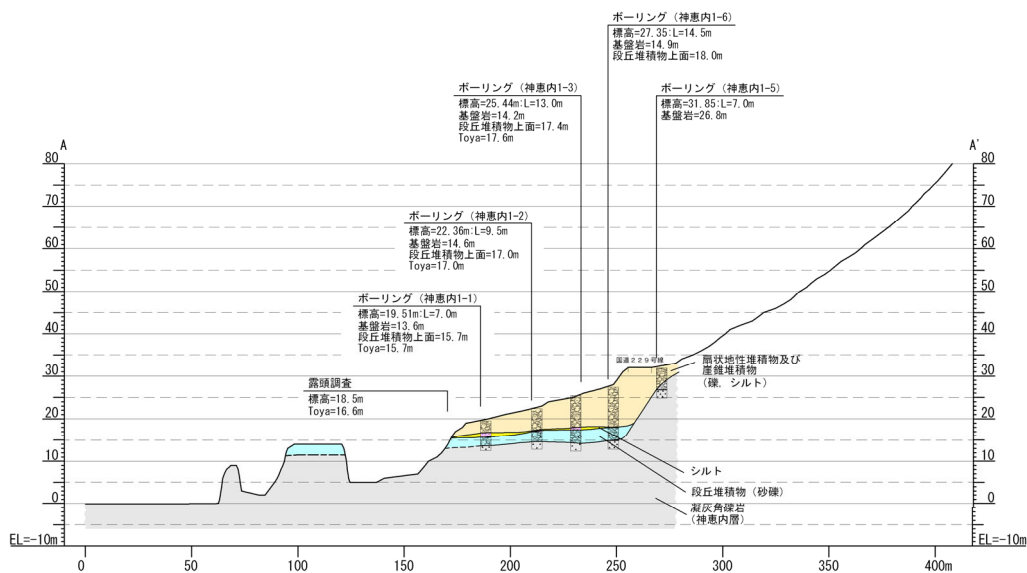
A-A'断面
