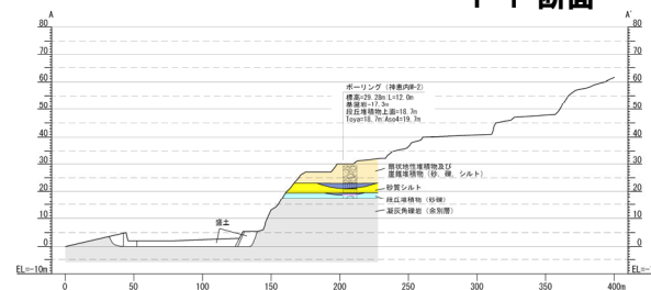
A-A' 断面
