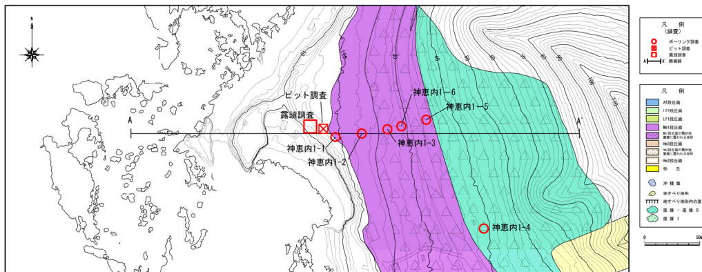
地形分類図
