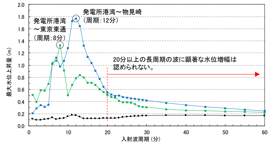
各評価位置における正弦波の入射波周期と最大水位上昇量の関係(水位増幅)
