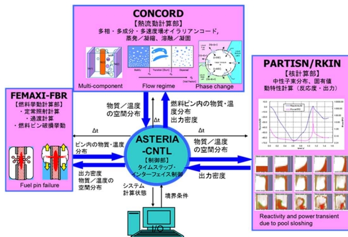
図 1 ASTERIA-SFR のコード構造
