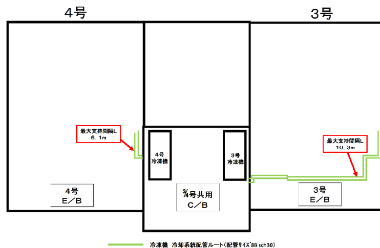
図 18-3-1 大飯3号との配管ルート（配管サイズ 8B sch30 EL26.0m の例）
