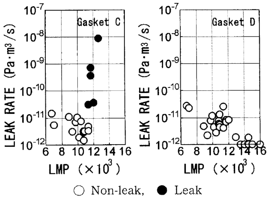
第 1-16 図 漏えい率と LMP の関係 (定数 C=20) (17)
