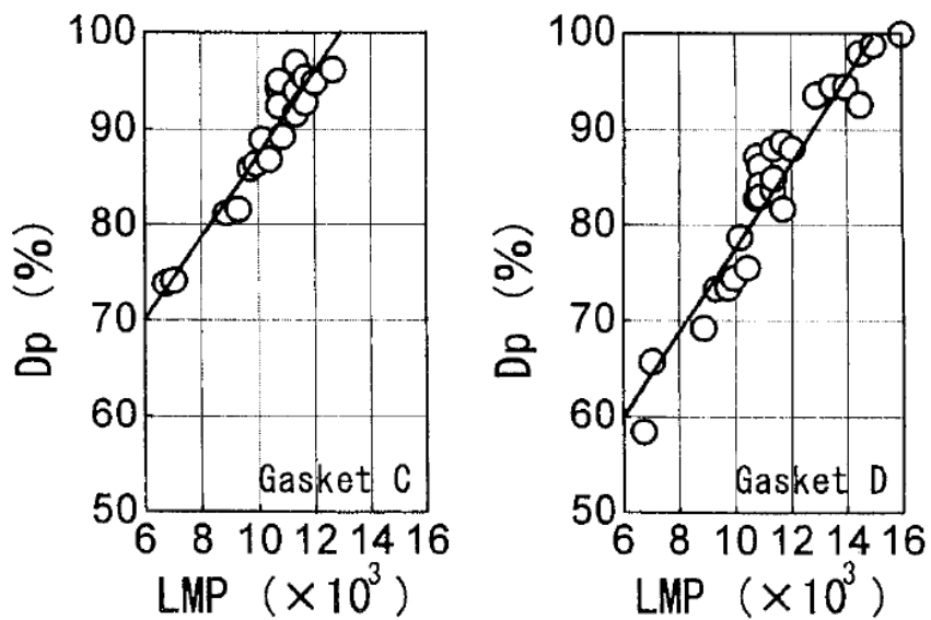
第 1-14 図 塑性変形率 D_p と LMP の関係 (17)
