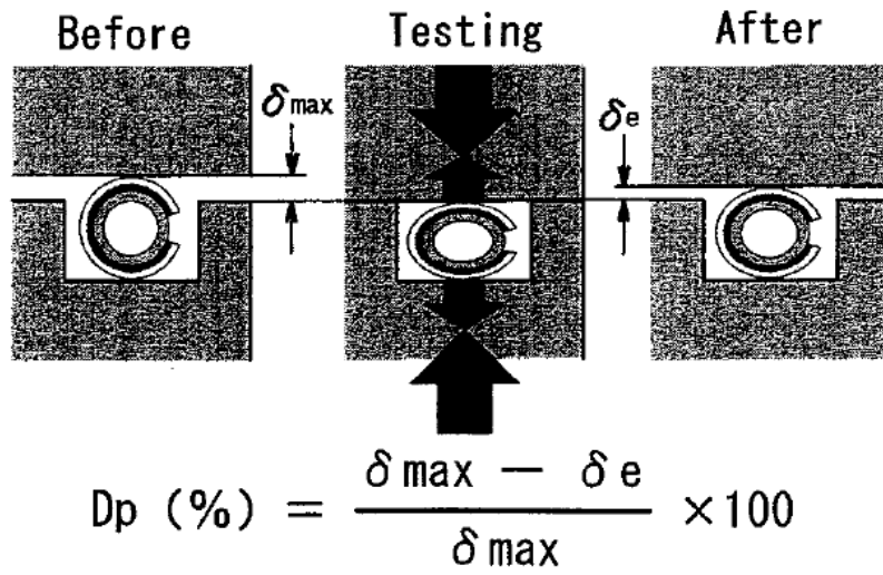
第 1-15 図 塑性変形率の定義 (17)
