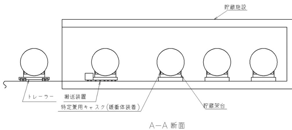
第 5 図 貯蔵施設概要図 (例)
