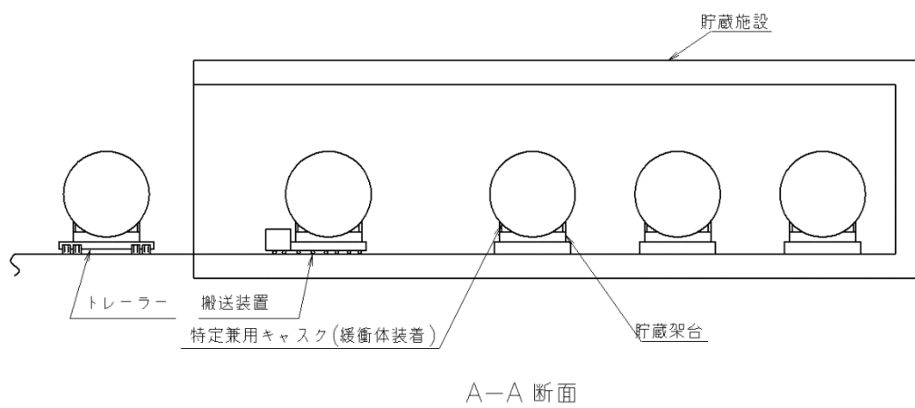
第 1-3 図 貯蔵施設概要図 (例)
