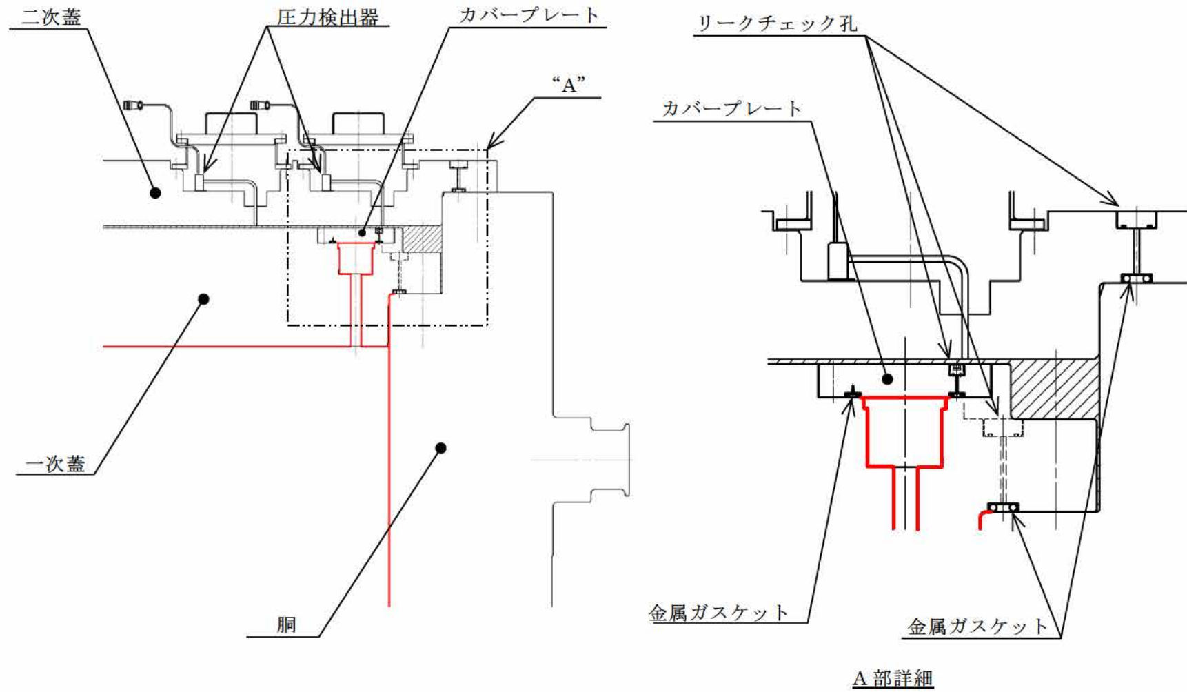
第 1-10 図 Hitz-B69 型のシール部詳細
