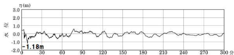
第1.3.2.15図 基準津波の時刻歴波形
