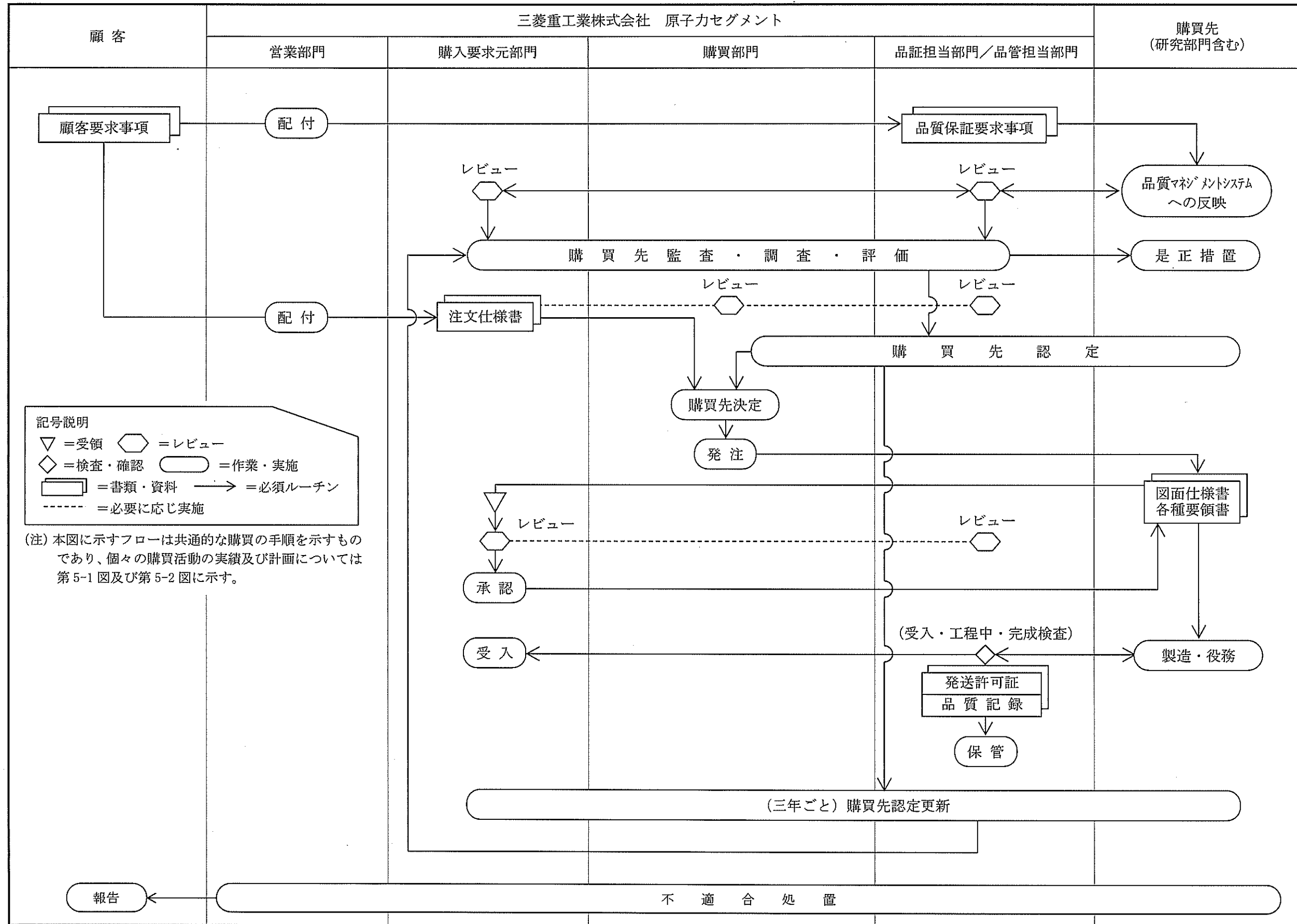
第5-3図 型式設計特定機器の設計及び製作に係る設計フロー図
