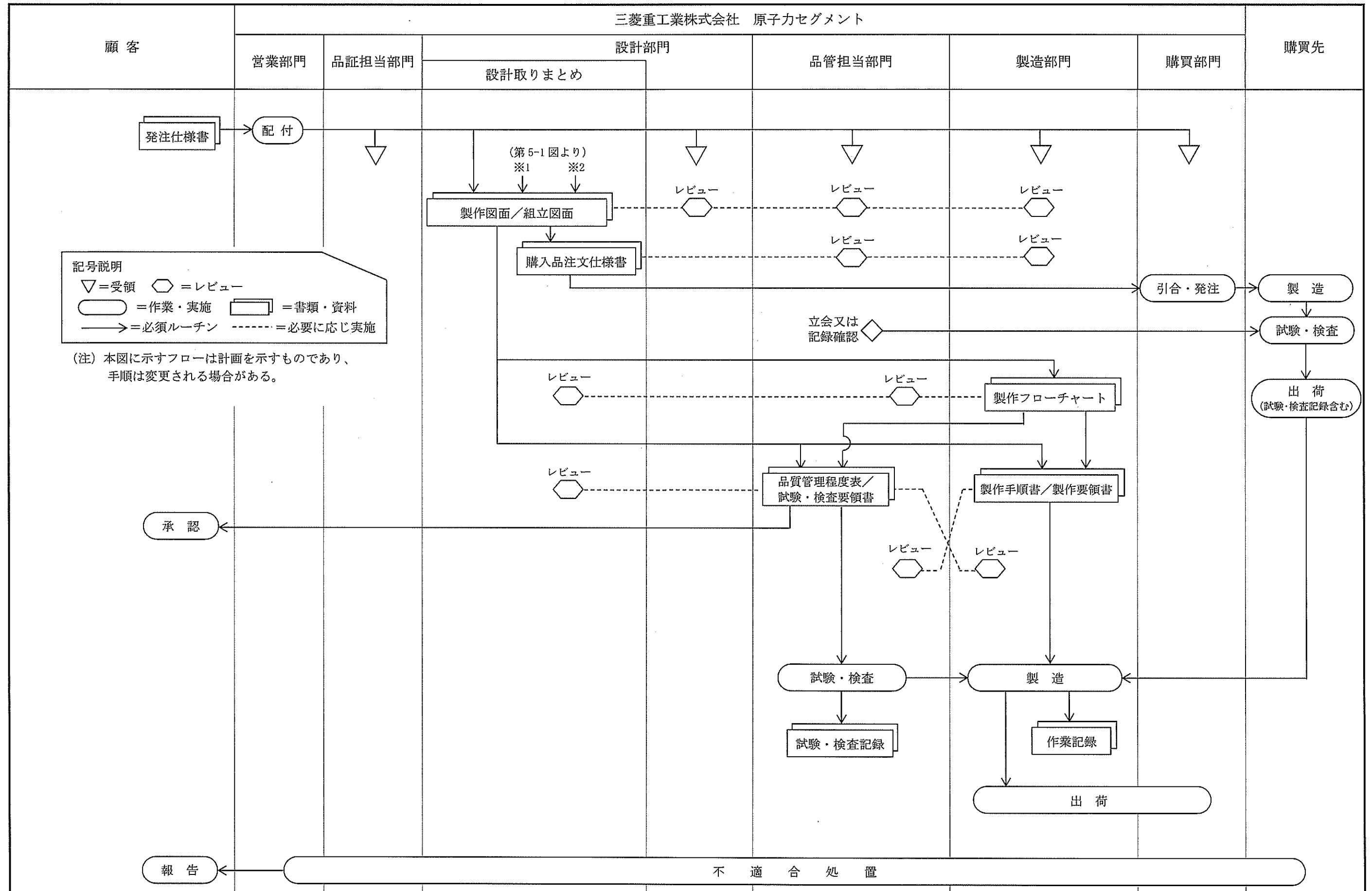
第5-2図 型式設計特定機器の設計及び製作に係る設計フロー図
