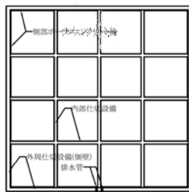
図 1-イ (ハ)-15 埋設設備群の配置図(平面)
