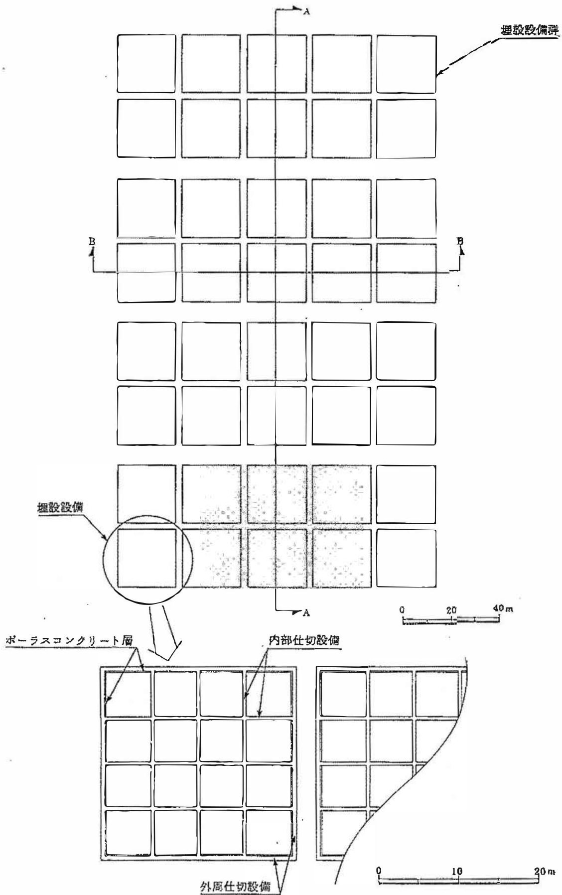
図1-イ(ハ)-1 埋設設備群の配置図 (平面)
