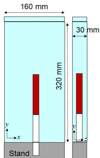
図 1 二次元温度成層化装置の概略図
