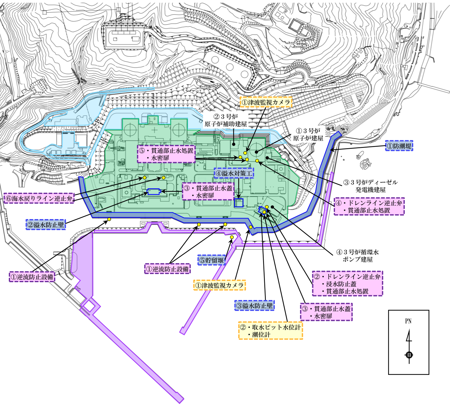
泊発電所3号炉 津波防護対策の概要図
