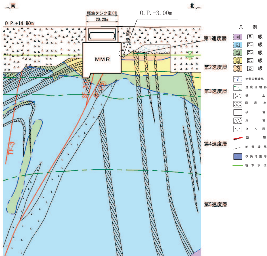
図 3-35 設計用地下水位 (南北方向)
