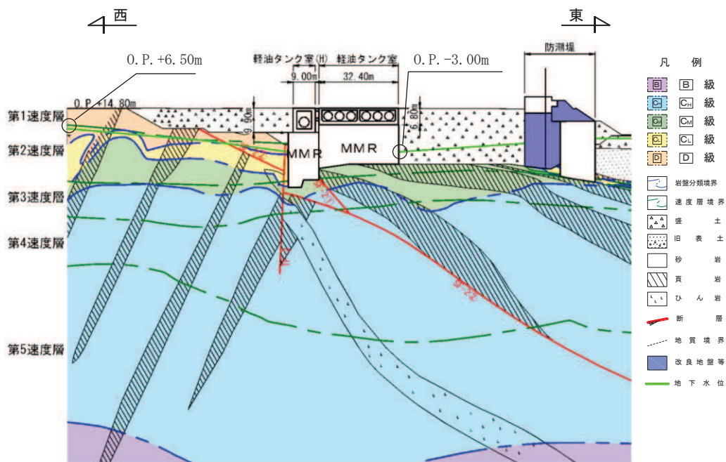
図 3-36 設計用地下水位 (東西方向)
