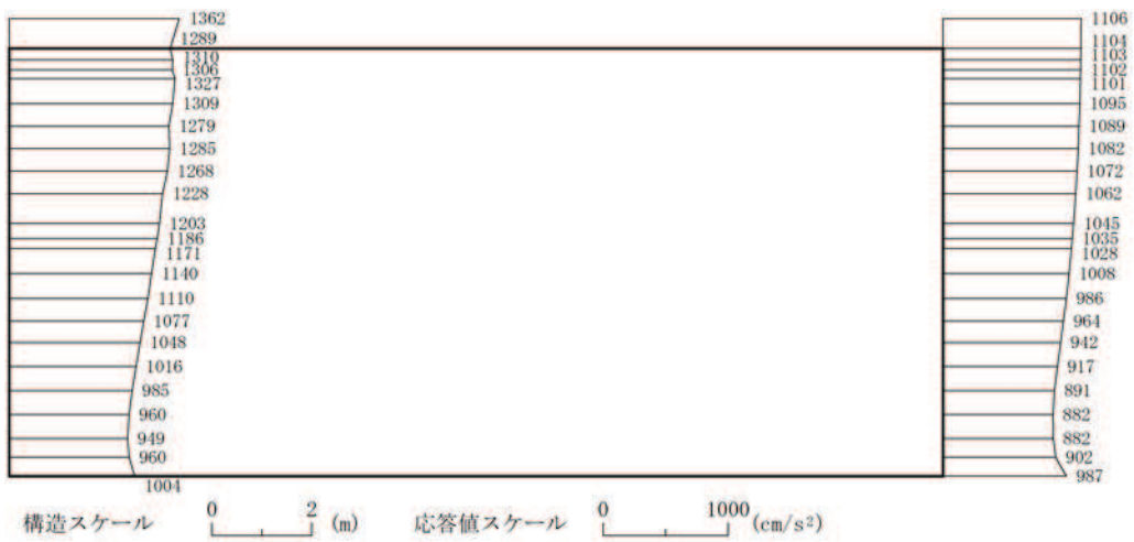
(b) S s - D 2 ( - + ) 鉛直
