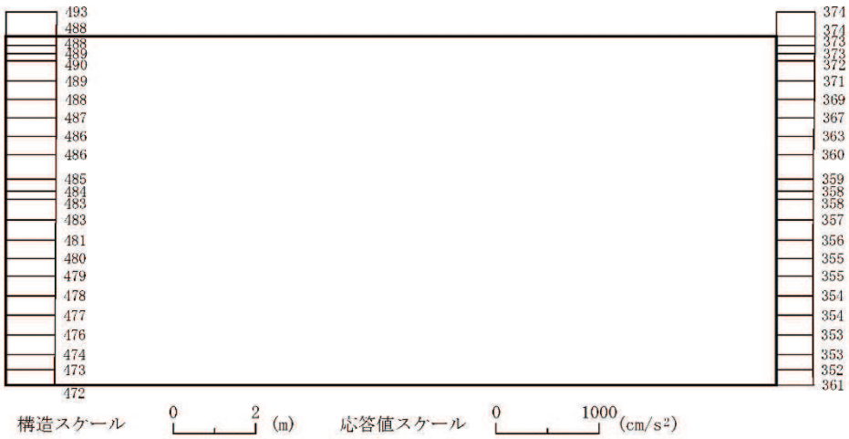
(b) S d - D 1 ( - + ) 鉛直
