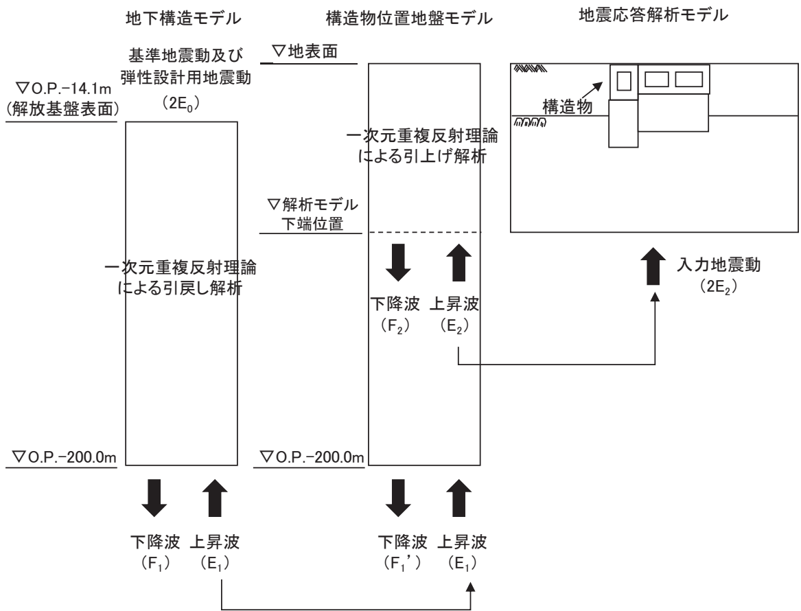
図3-4 入力地震動算定の概念図（基準地震動 S_s 及び弾性設計用地震動 S_d ）
