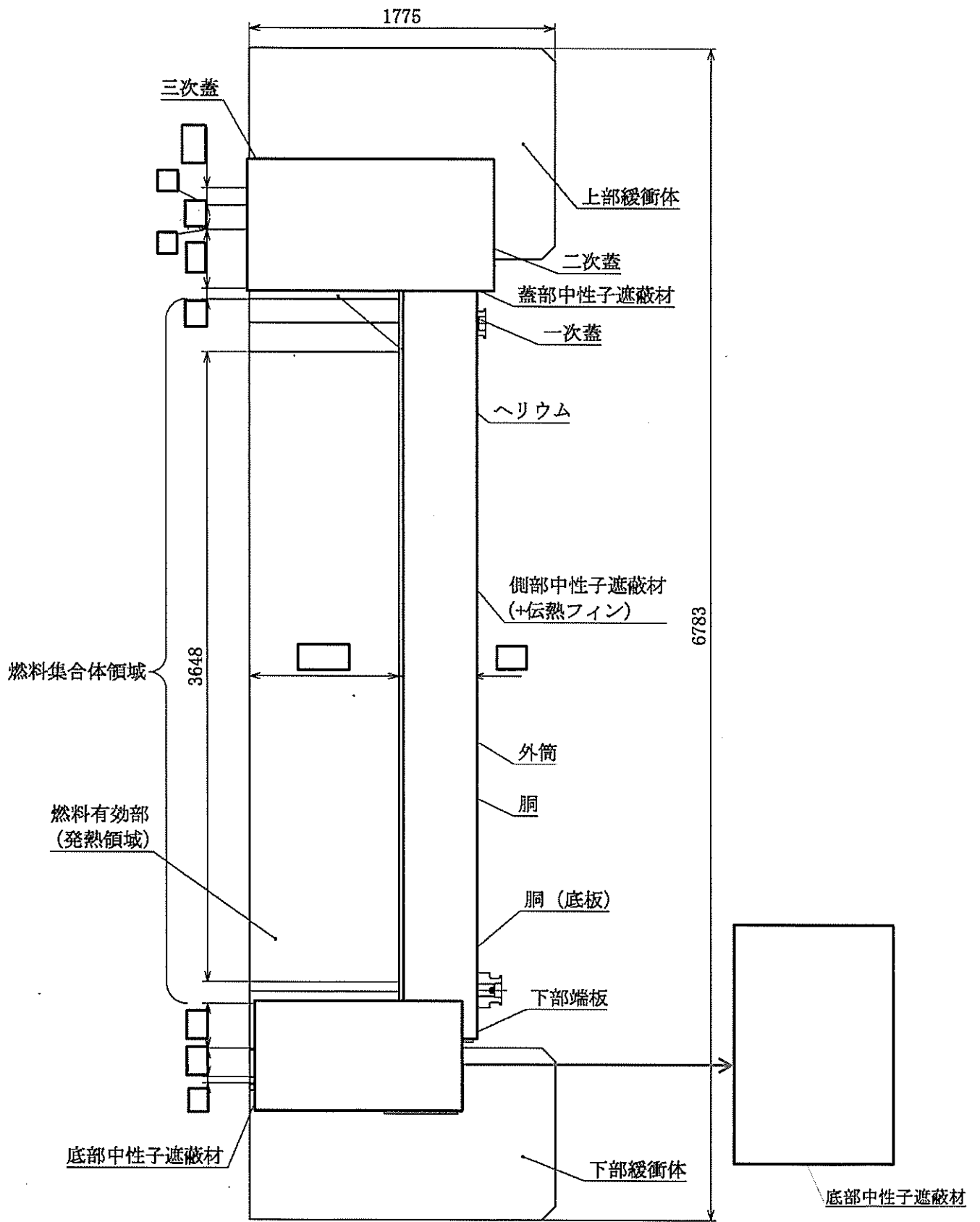
(D)-第B.1図 一般の試験条件の全体モデル形状図 (1/2) (縦断面図)
