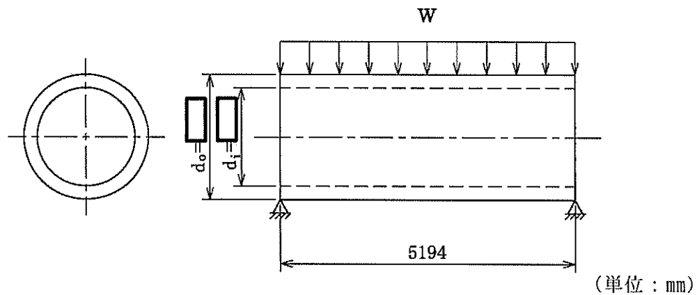
(D)-第 A. 37 図 両端単純支持された容器本体の解析モデル図
