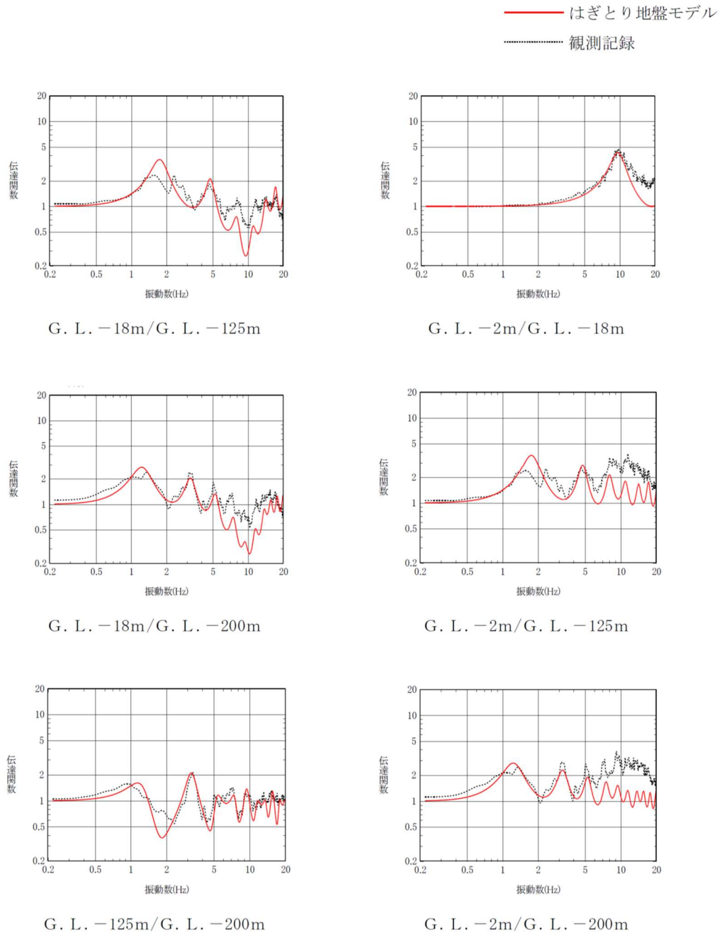
第 5-4 図(1) 観測記録に基づく伝達関数とはぎとり地盤モデルによる伝達関数の比較 (中央地盤)
