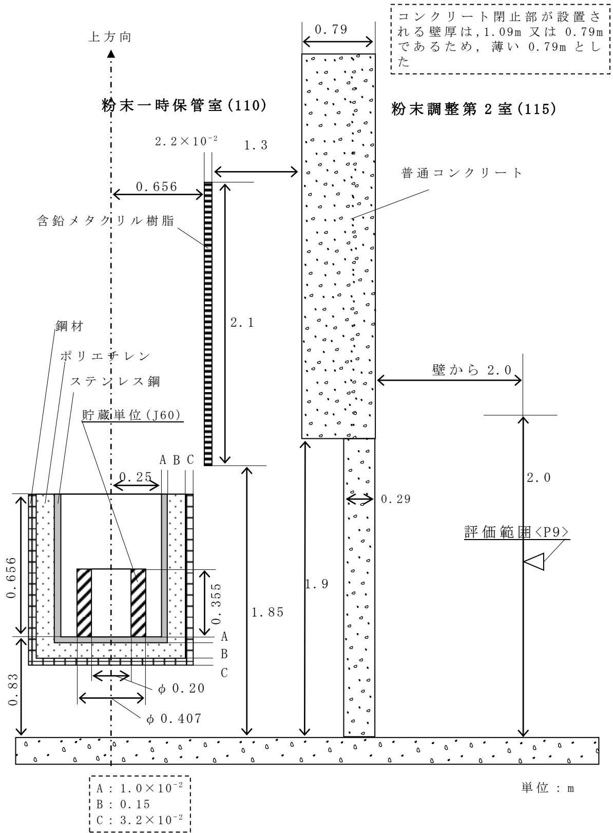
第 2.2-1 図 (14) 粉末一時保管装置：西方向線量率計算モデル図 (線源形状：有限円筒)
