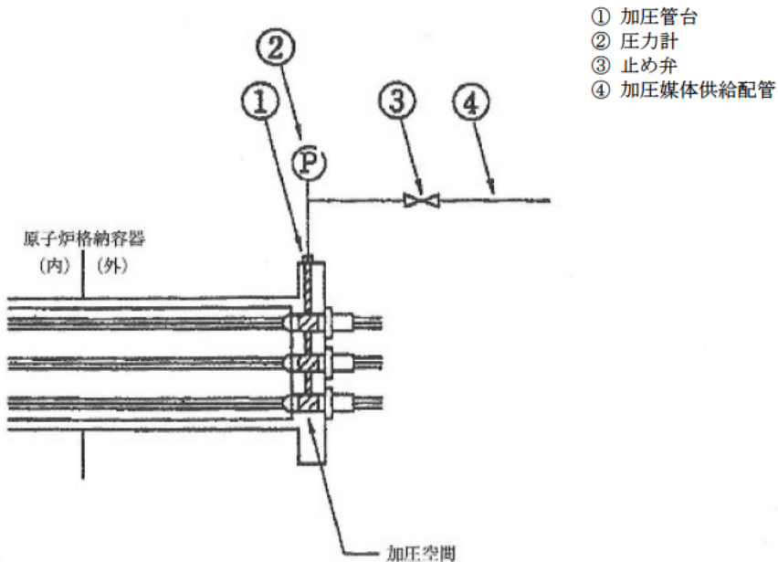
図 B 種試験 (電気配線用貫通部) 概念図 [1]
