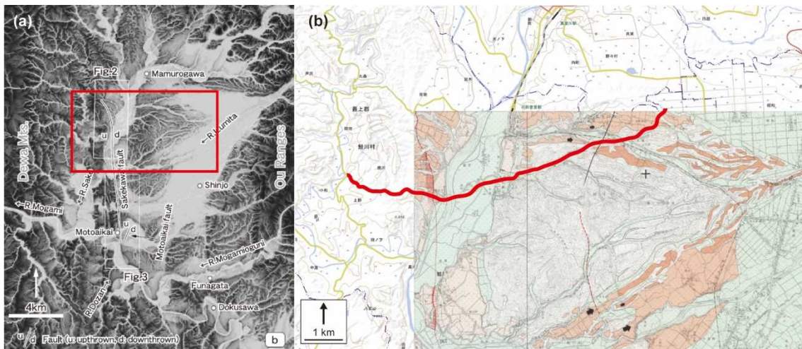
図1 新庄盆地西縁断層帯及び調査測線。(a) 新庄盆地とその周辺の地形及び新庄盆地西縁断層帯（松浦、2003）(b) 探査測線（赤線）。原図は都市圏活断層図（新庄）及び地理院タイルを使用。
