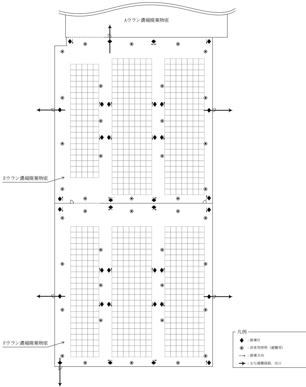
図1 安全避難通路等設備 配置概略図
