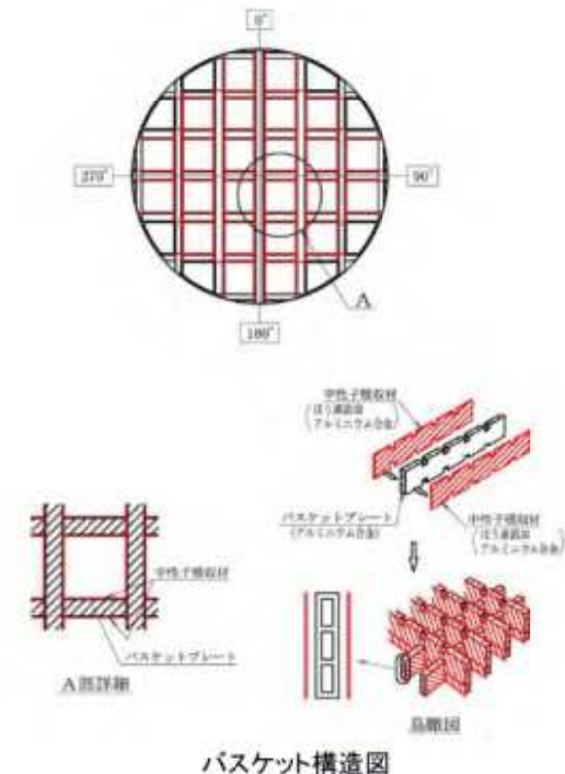
バスケット構造図
