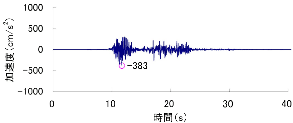
Ss-3 (UD 方向)
