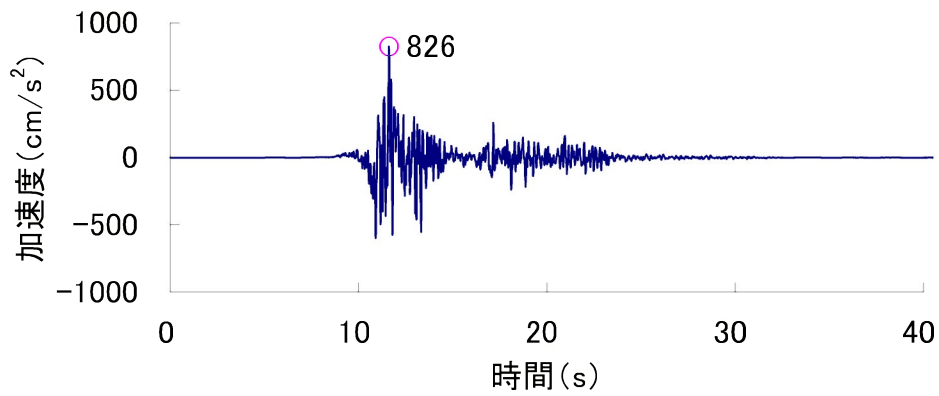
Ss-3 (EW 方向)
