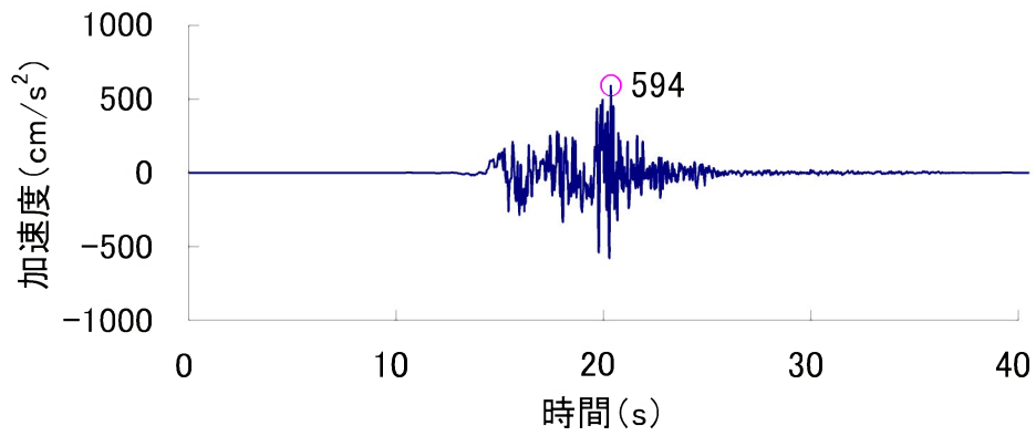
Ss-17 (NS 方向)
