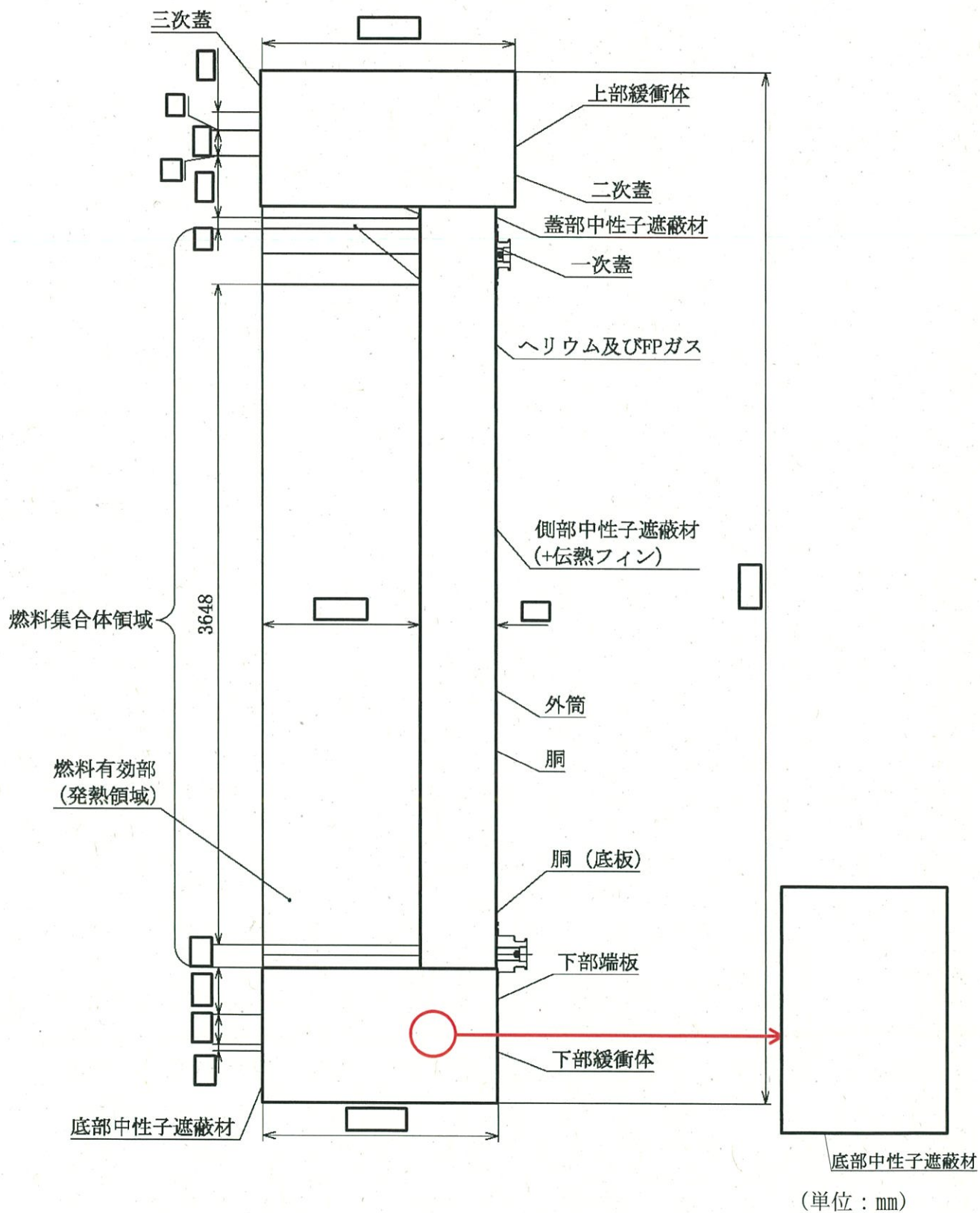
(口)-第 B. 10 図 特別の試験条件の全体モデル形状図 (1/2) (縦断面図)
