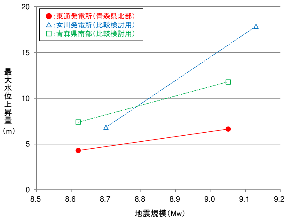
■地震規模と津波高さ(最大水位上昇量)の関係
