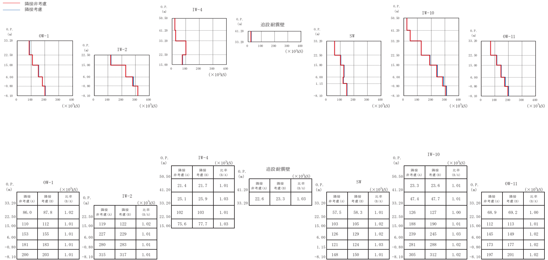
図 3.2-16 最大応答せん断力の比較 (02R/B, EW 方向)
