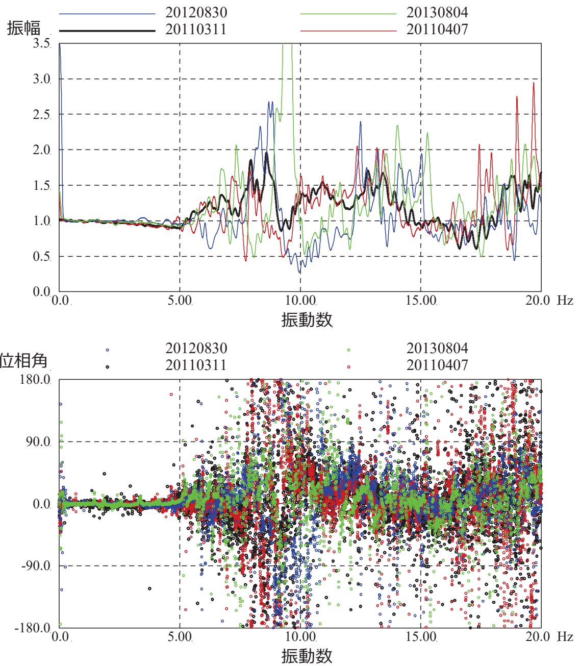
図 3-19 検討対象地震の平均波に対する端部の観測波形の伝達関数の比較 (3.11 地震後の地震との比較) (EW 方向北側)
