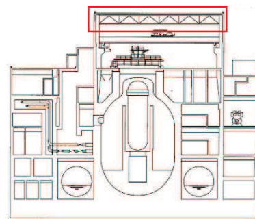
断面図(NS方向)
