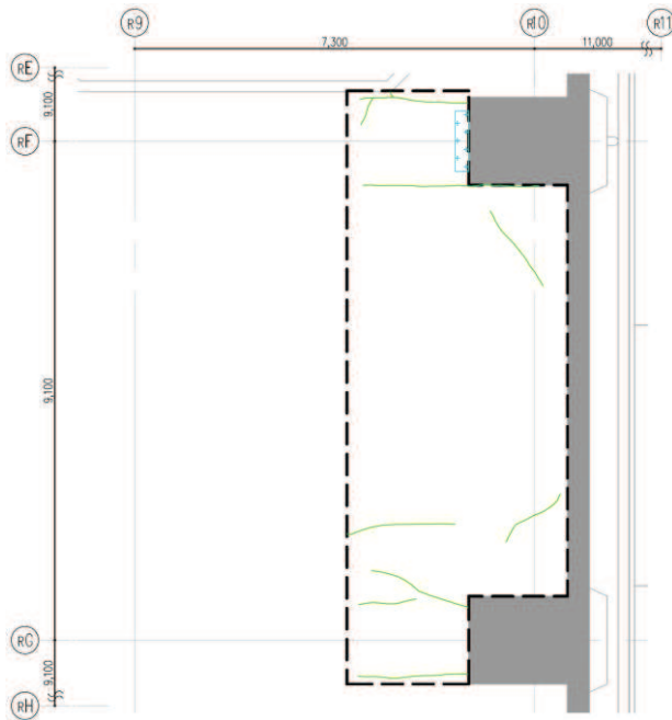
図 4-2(2) 原子炉建屋 地上 3 階床ひび割れ調査結果 (発生応力の小さい部位を選定)
