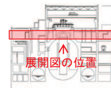
断面図
