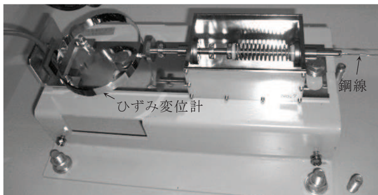
図 1-5 変位計及び変位計取付治具の設置状況
