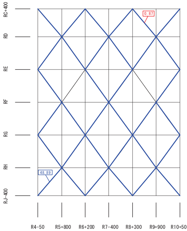
屋根トラス下弦面 (0. P. 47.125)
