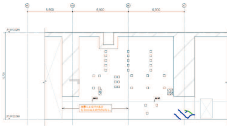
(東面 立面図)
