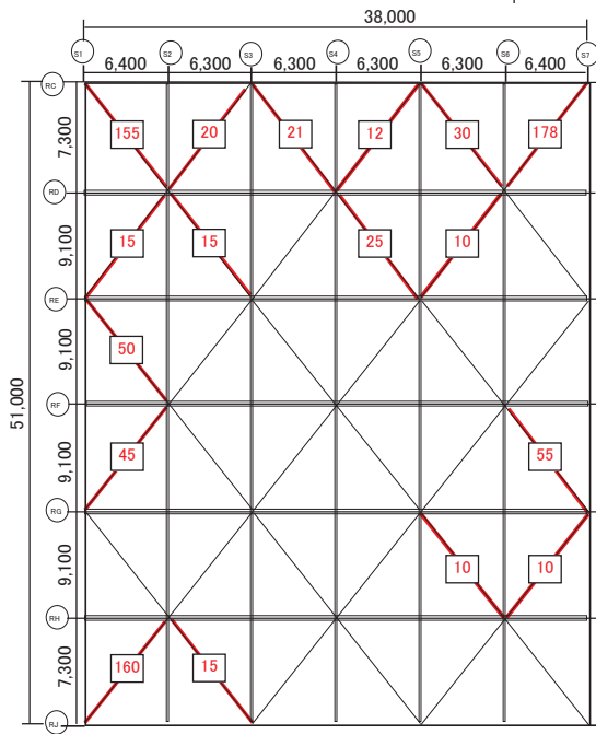
下弦水平ブレース
