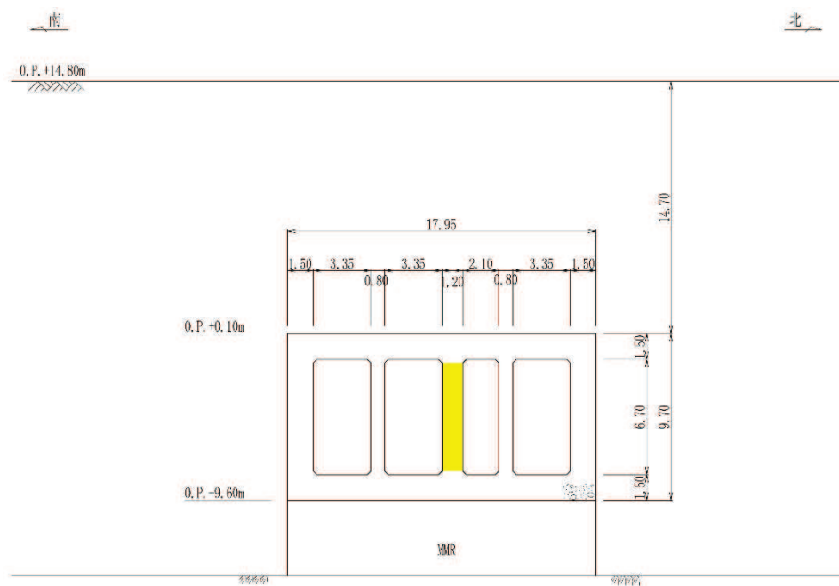
A-A 断面
