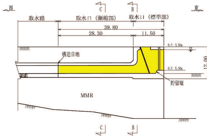
A-A 断面
