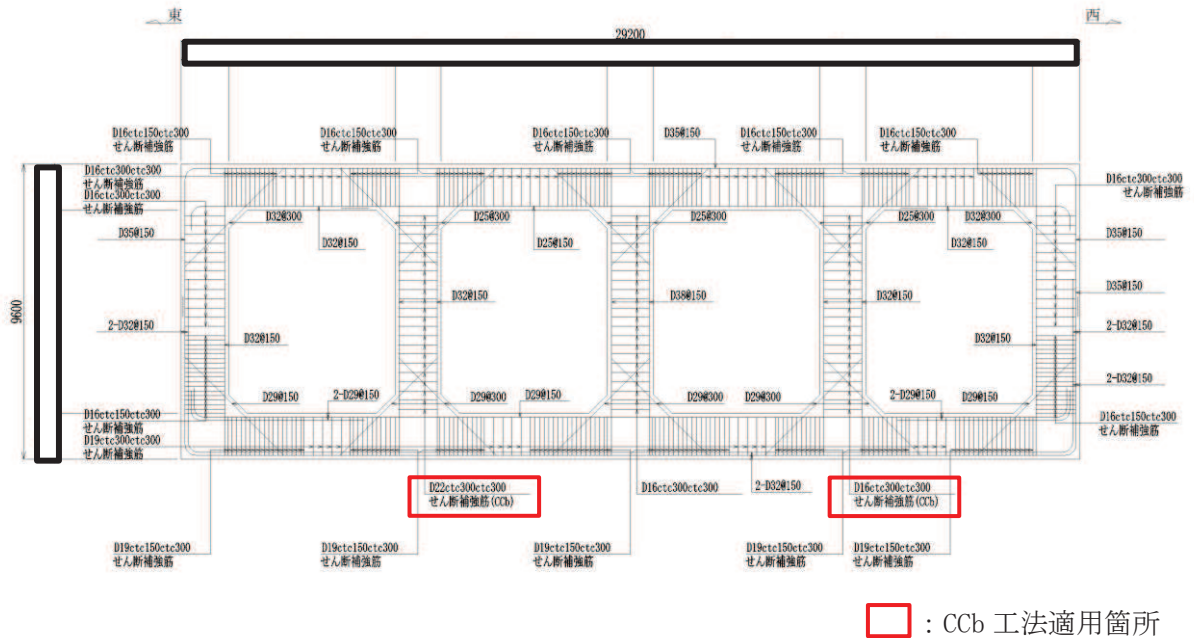
図4-2 取水路（漸拡部）の補強仕様
