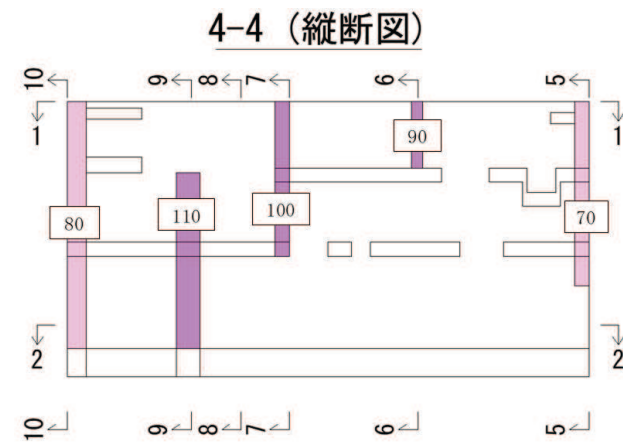
図 3-14 評価部材位置 (第 3 号機海水ポンプ室)
