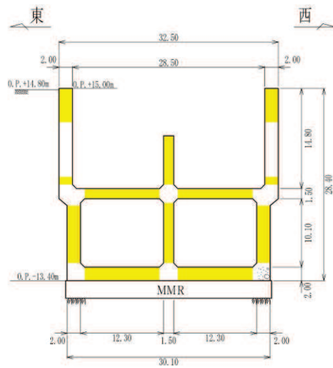
C-C 断面
