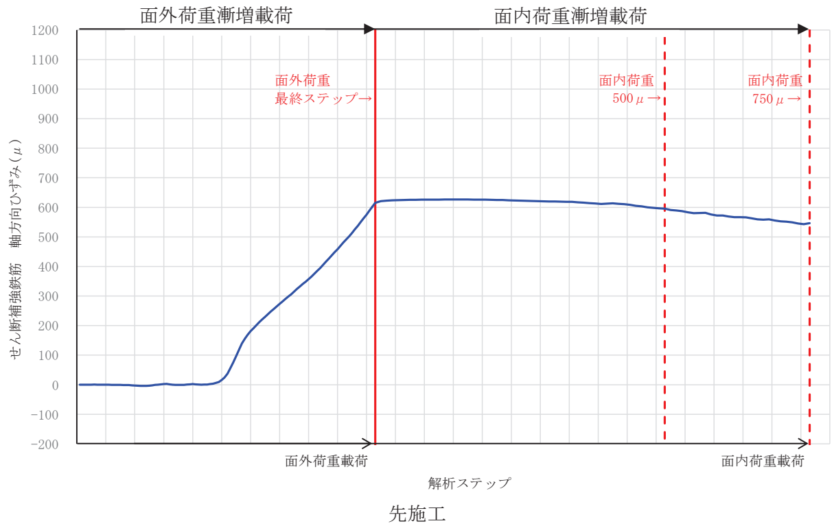
図 6-9 せん断補強鉄筋の軸方向ひずみ
