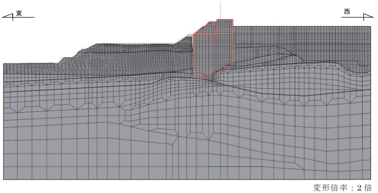
図 2-9 有効応力解析（断面②）の残留変形図
