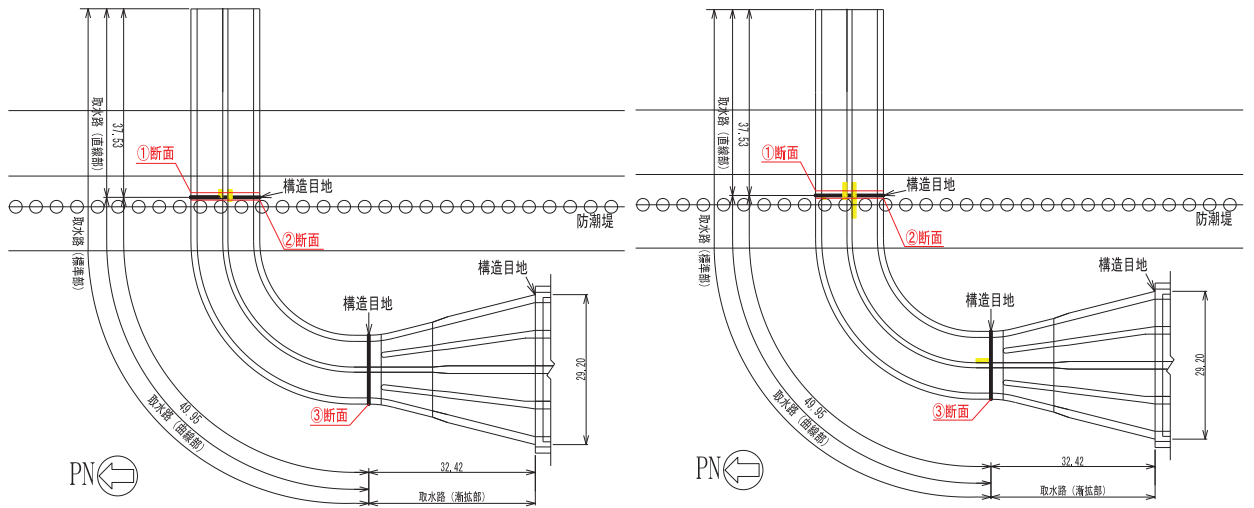
平面図 (頂版)
