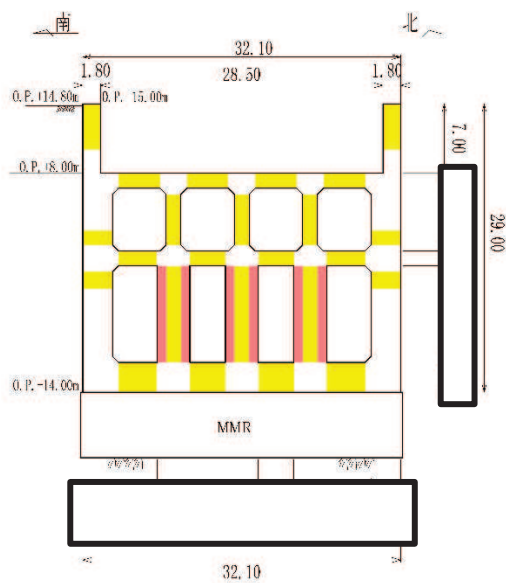
A-A 断面
