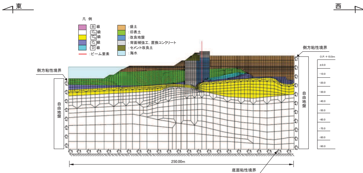
図 2-6 断面②の解析モデル
