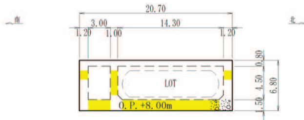
B-B 断面
