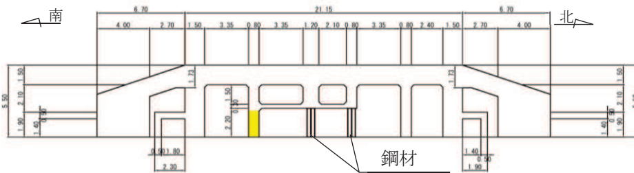
断面図 (C-C 断面)
