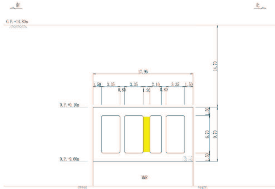
A-A 断面
