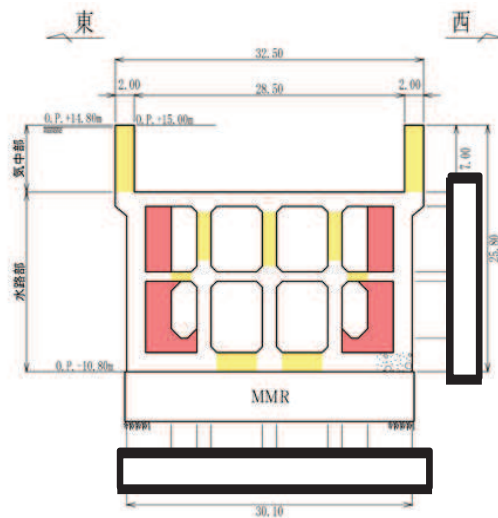
A-A 断面
