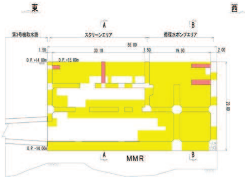
C-C 断面
