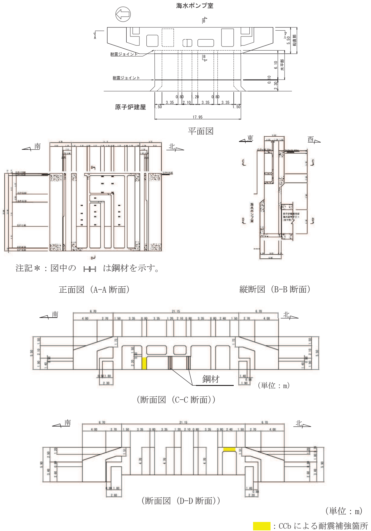
図 2-8 CCb による耐震補強対象の構造物 （原子炉機器冷却海水配管ダクト（鉛直部））
