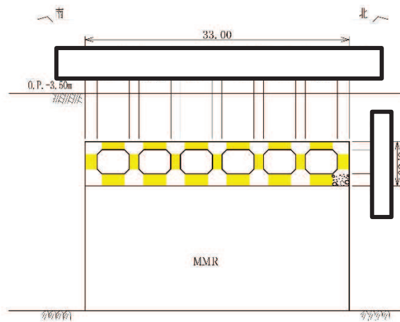
C-C 断面
