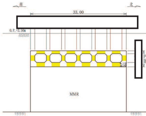
C-C 断面
