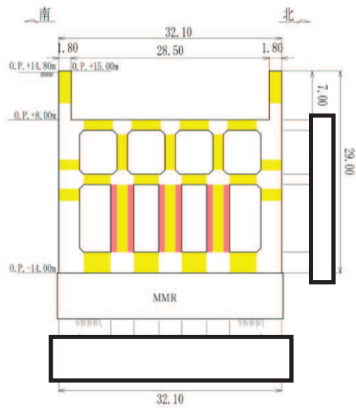
A-A 断面
