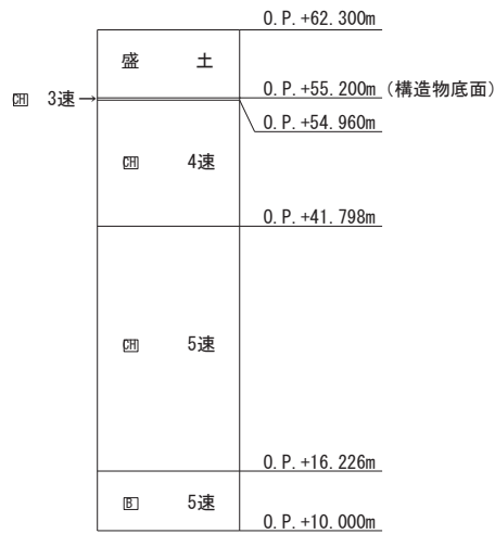
図 5-3 ガスタービン発電設備軽油タンク室 一次元解析モデル
