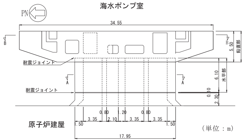
図 4.6-2 原子炉機器冷却海水配管ダクト平面図 南 北
