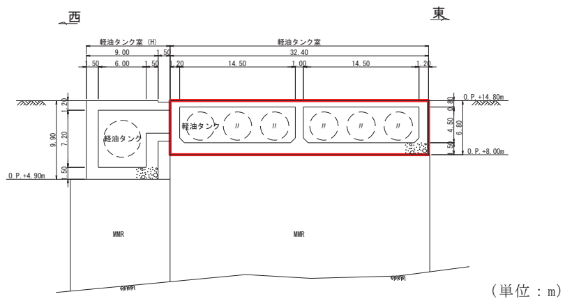
図 4.8-4 軽油タンク室断面図 (B-B 断面, 東西 (タンク室))
