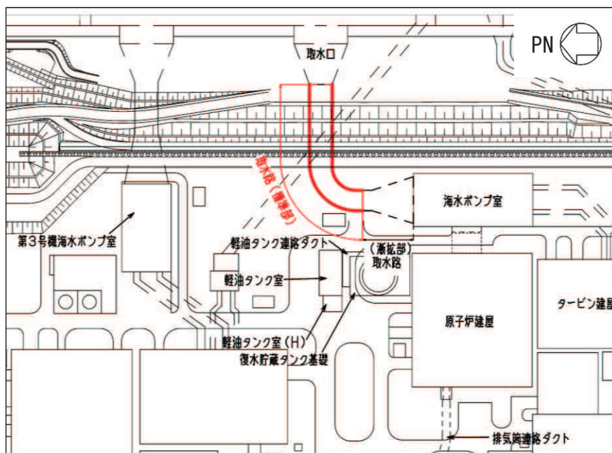
図 4.12-1 取水路（標準部）配置図
