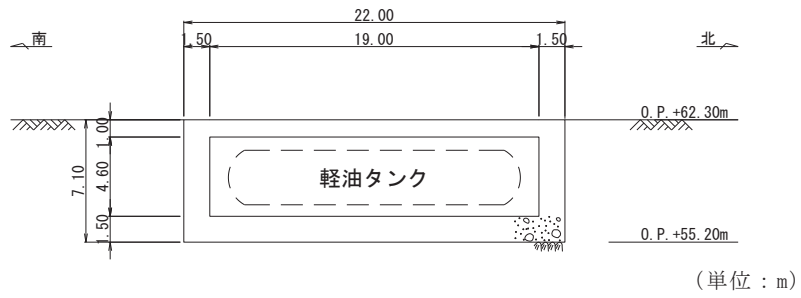
図 4.14-3 ガスタービン発電設備軽油タンク室断面図 (A-A 断面, 南北)
