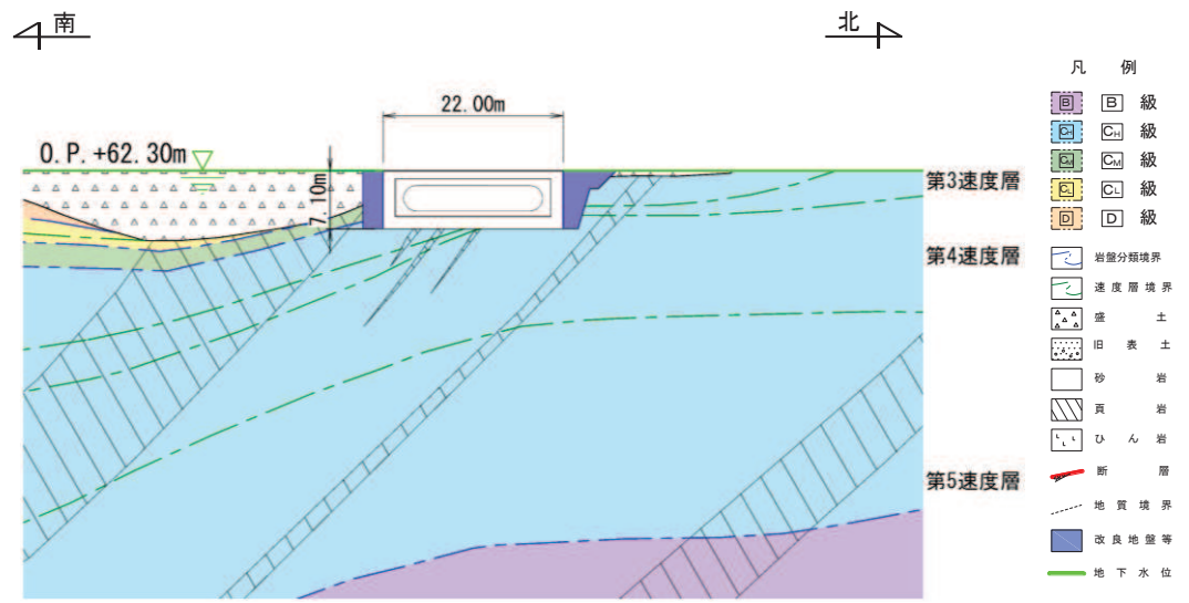
図 4.14-8 ガスタービン発電設備軽油タンク室地質断面図 (B-B 断面)
