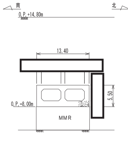
図 4.12-3 取水路（標準部）断面図（A-A 断面）
