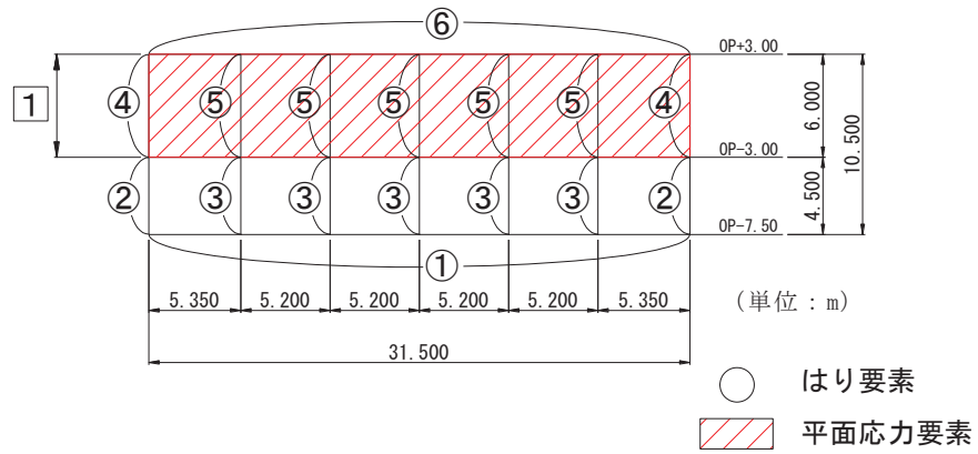
図11.2-10(1) 等価剛性設定用モデル (取水口 (標準部))
