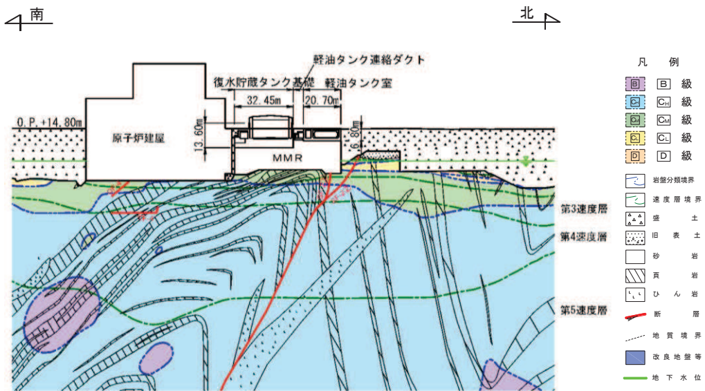
図 4.13-7 復水貯蔵タンク基礎地質断面図 (A-A 断面)
