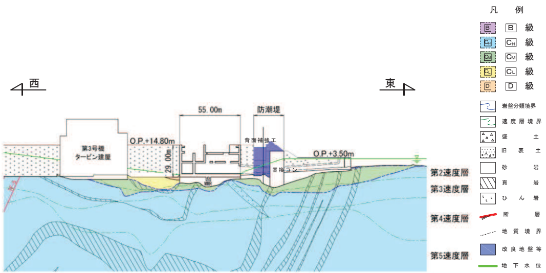
図 4.15-10(3) 第3号機海水ポンプ室 地震時荷重算出断面図 (東西方向)
