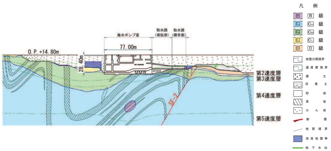
図 4.7-9 取水路（漸拡部）地質断面図（A-A 断面）
