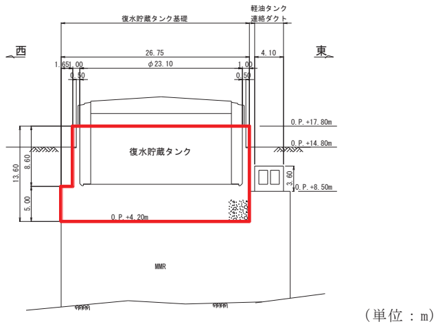
図 4.13-4 復水貯蔵タンク基礎断面図 (B-B 断面, 東西)
