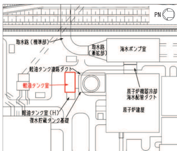
図 4.8-1 軽油タンク室配置図
