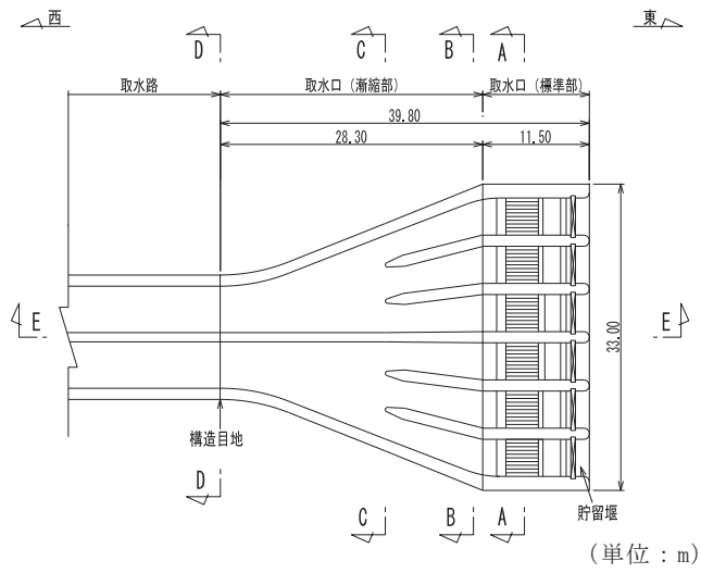
図 4.11-2 取水口，貯留堰平面図
