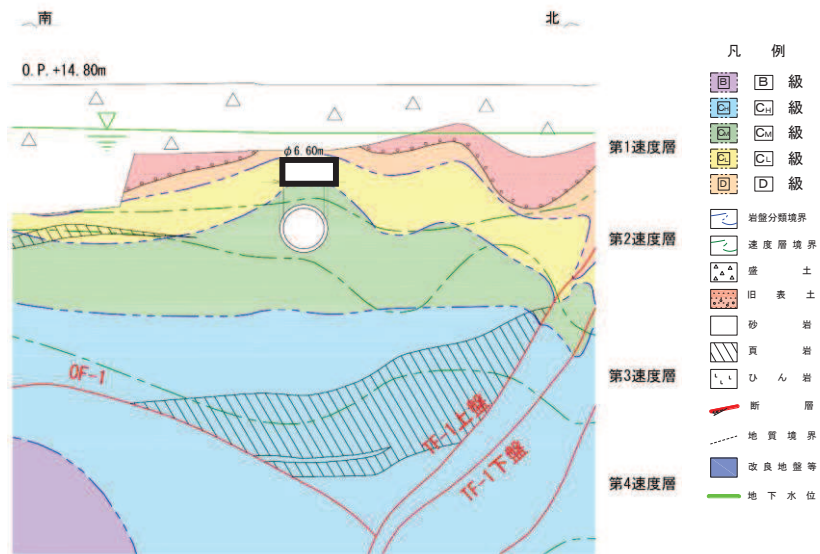
図 4.5-11 排気筒連絡ダクト（岩盤部） 評価対象断面図（断面⑤）
