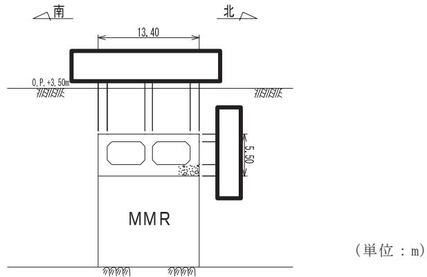
図 4.11-6 取水口断面図 (D-D 断面, 南北 (漸縮部))
