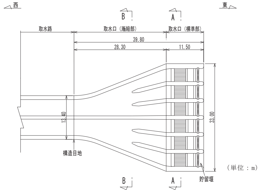
図11.2-6 取水口平面図
