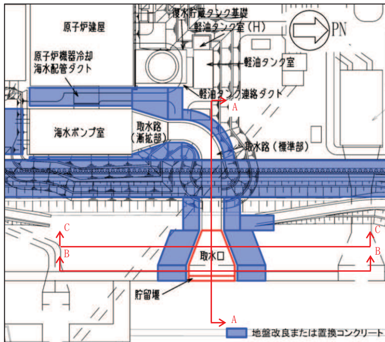
図 4.11-9 取水口，貯留堰掘削図
