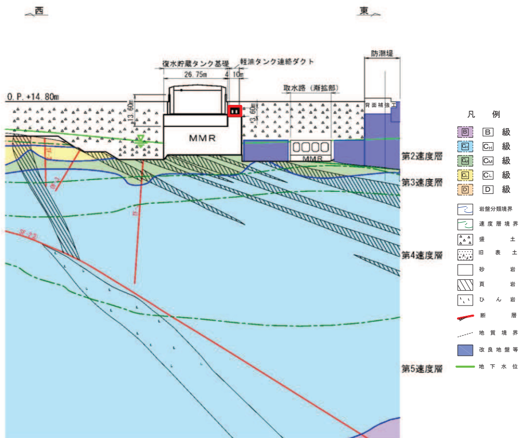
図 4.4-9 軽油タンク連絡ダクト地質断面図 (B-B 断面)
