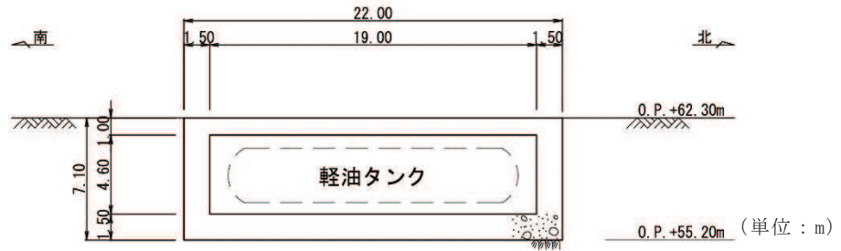
図11.2-2 ガスタービン発電設備軽油タンク室断面図 (A-A断面)
