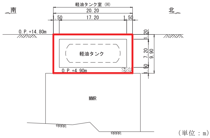
図 4.9-3 軽油タンク室 (H) 断面図 (A-A 断面, 南北)
