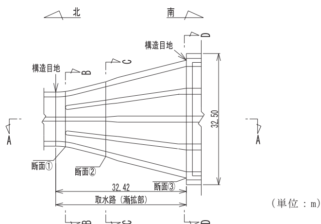
図 4.7-4 取水路（漸拡部）平面図及び候補断面位置
