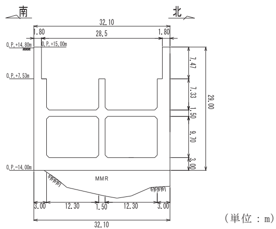
図 4.15-4 第 3 号機海水ポンプ室断面図 (B-B 断面)
