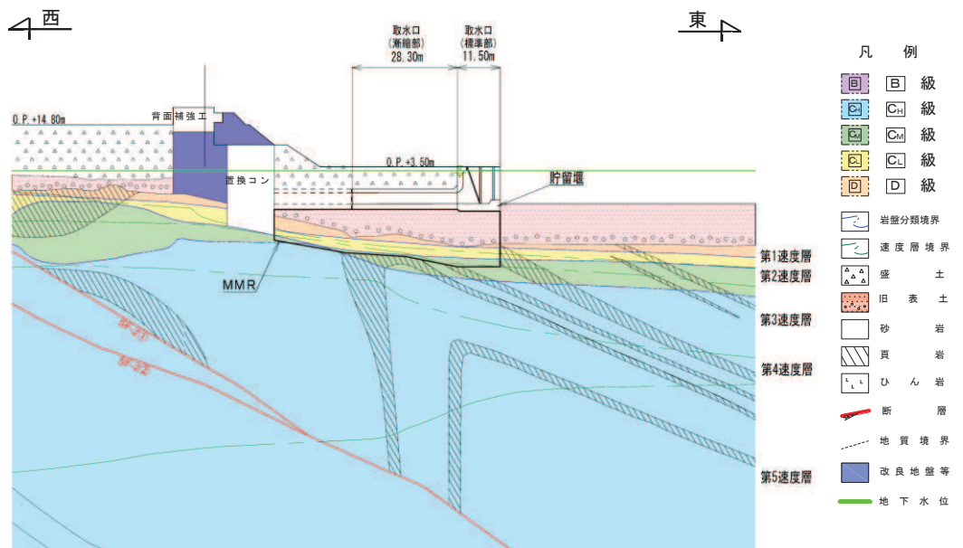
図 4.11-10 取水口，貯留堰地質断面図（縦断，A-A 断面）
