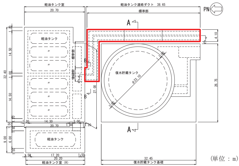
図 4.4-2 軽油タンク連絡ダクト平面図
