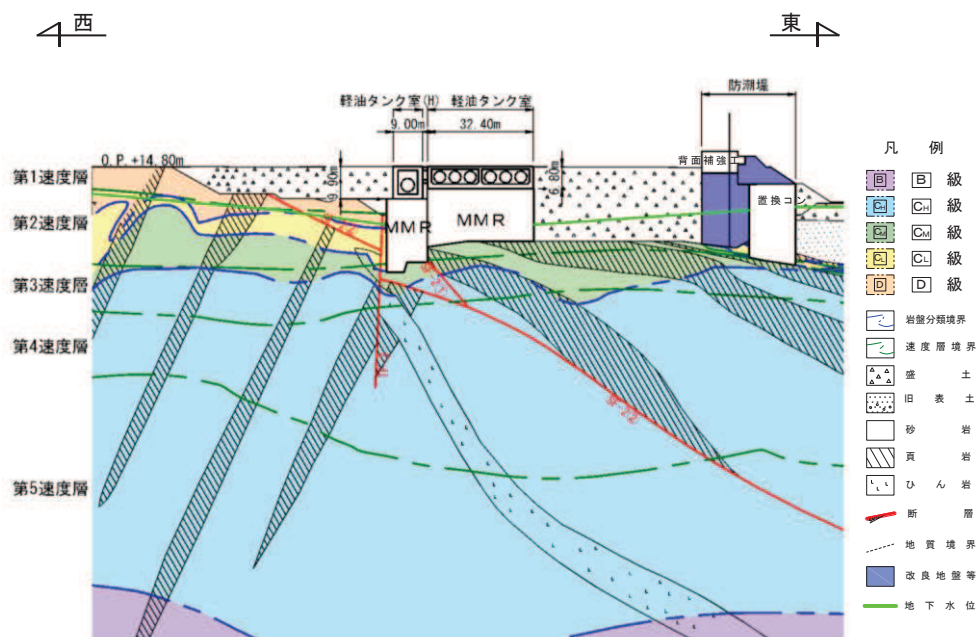
図 4.8-9 軽油タンク室地質断面図 (B-B 断面, 東西 (タンク室))
