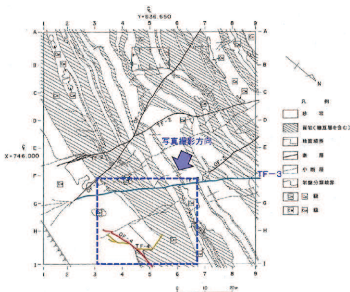
2号原子炉建屋掘削底盤スケッチ
