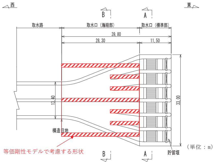
図11.2-9 等価剛性モデル範囲のイメージ図
