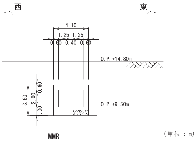
図 4.4-4 軽油タンク連絡ダクト断面図 (A-A 断面, 標準部)
