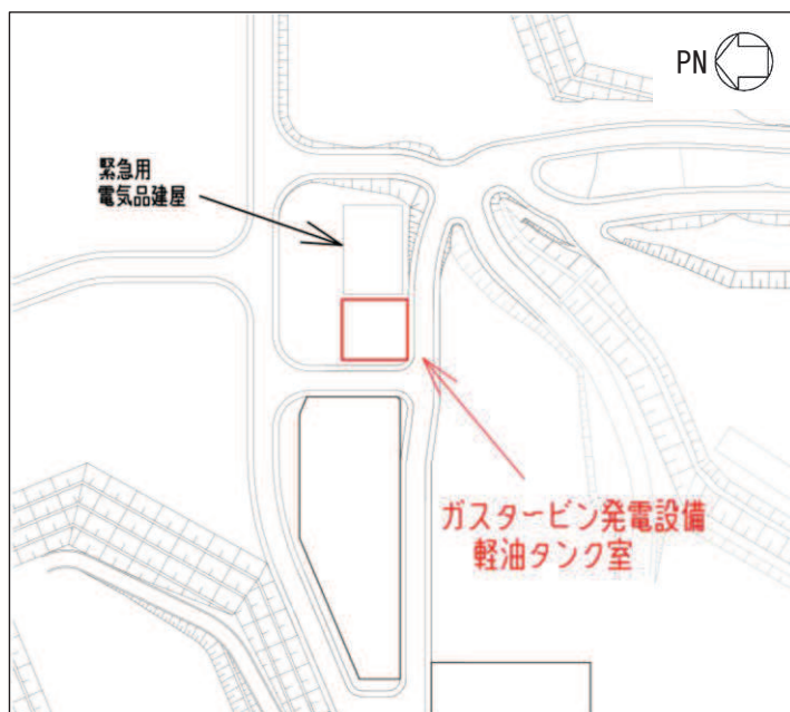
図 4.14-1 ガスタービン発電設備軽油タンク室配置図
