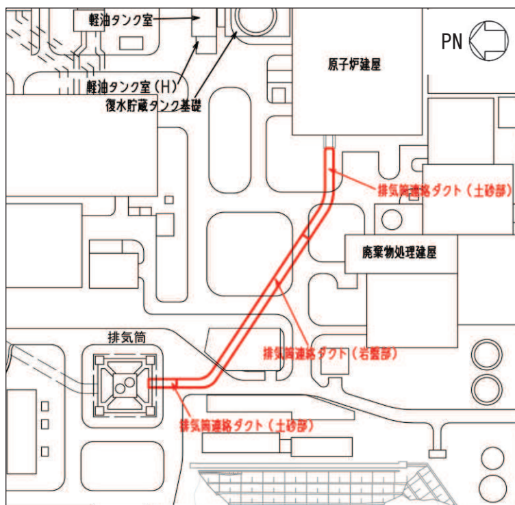
図 4.5-1 排気筒連絡ダクト配置図
