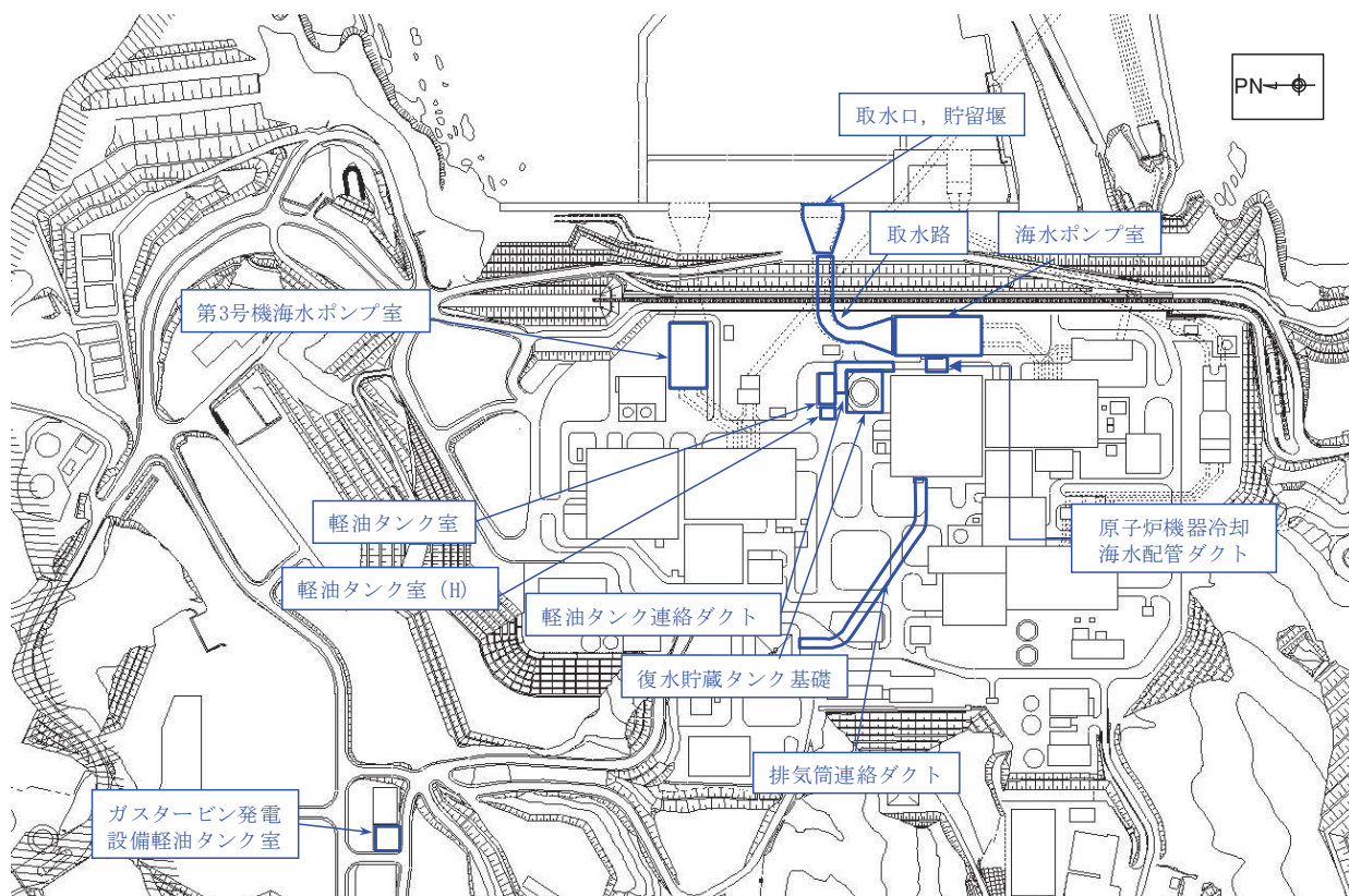
図1-1 屋外重要土木構造物等 位置図
