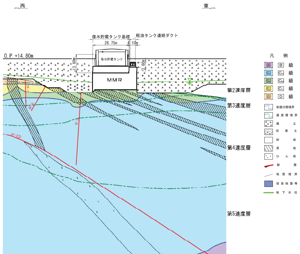
図 4.13-8 復水貯蔵タンク基礎地質断面図 (B-B 断面)
