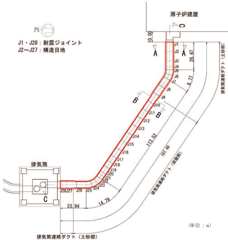
図 4.5-2 排気筒連絡ダクト平面図
