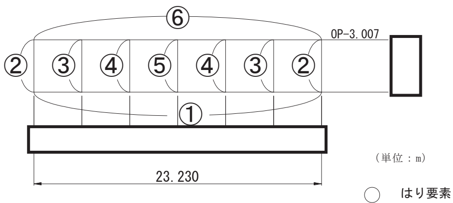
図11.2-11(1) 等価剛性設定用モデル（取水口（漸縮部））
