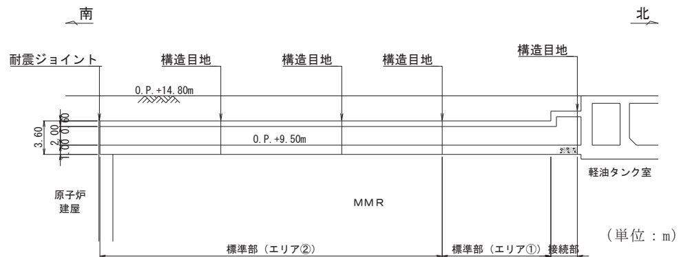
図 4.4-6 軽油タンク連絡ダクト縦断面図 (C-C 断面)
