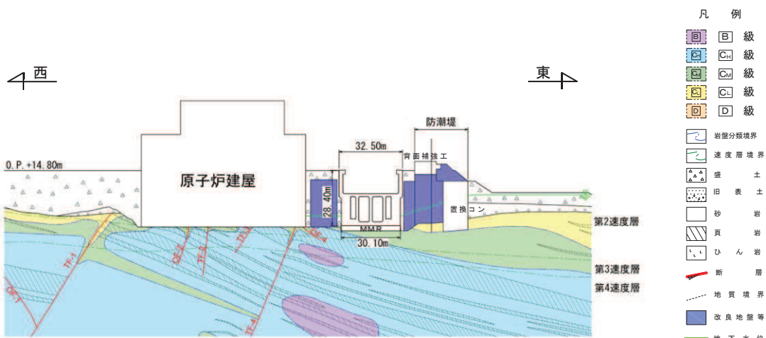
図 4.10-12(2) 海水ポンプ室 地震時荷重算出断面図（東西方向：補機ポンプエリア）
