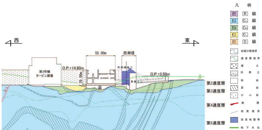
図 4.15-8 第3号機海水ポンプ室地質断面図 (A-A 断面)
