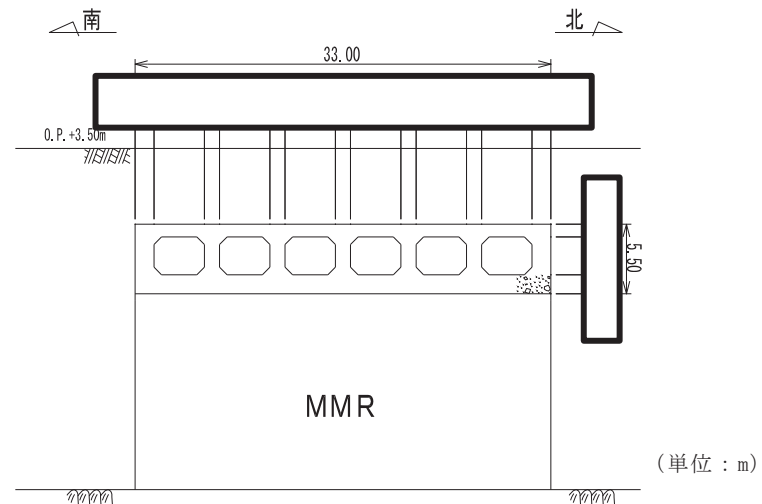
図 4.11-4 取水口断面図 (B-B 断面，南北 (漸縮部))
