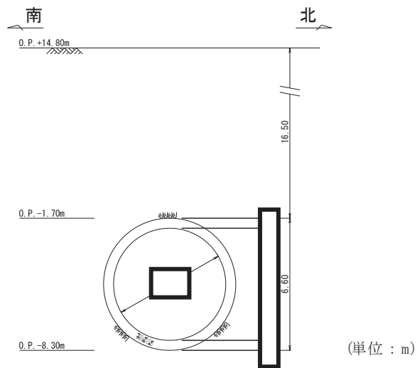
図 4.5-4 排気筒連絡ダクト断面図 (B-B 断面, 岩盤部)
