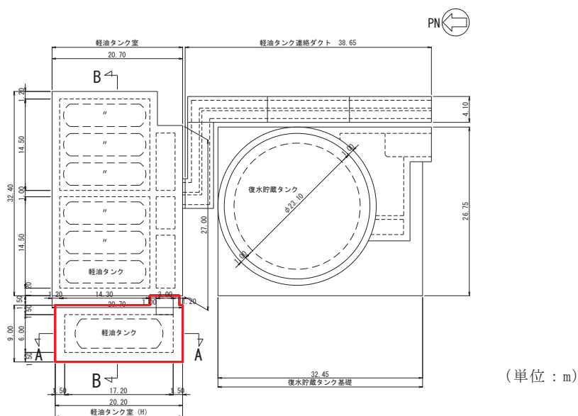
図 4.9-2 軽油タンク室 (H) 平面図
