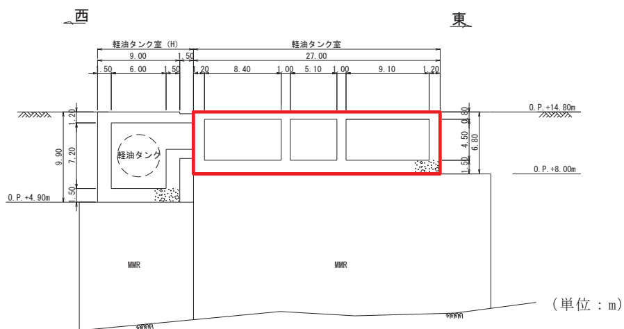
図 4.8-5 軽油タンク室断面図 (C-C 断面, 東西 (ポンプ室))
