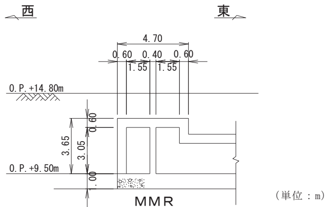
図 4.4-5 軽油タンク連絡ダクト断面図 (B-B 断面, 接続部)
