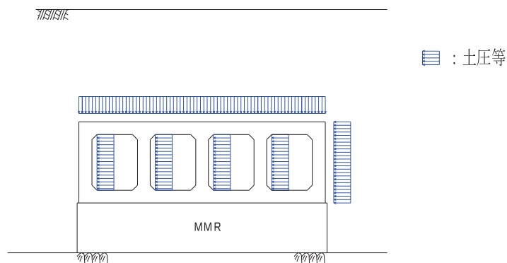
図 4.7-11 荷重イメージ図
