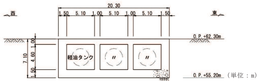
図11.2-3 ガスタービン発電設備軽油タンク室断面図 (B-B断面)
