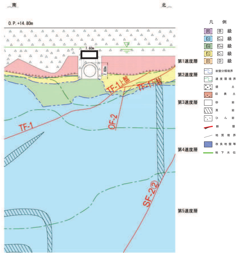
図 4.5-10 排気筒連絡ダクト（土砂部） 評価対象断面図（断面③）
