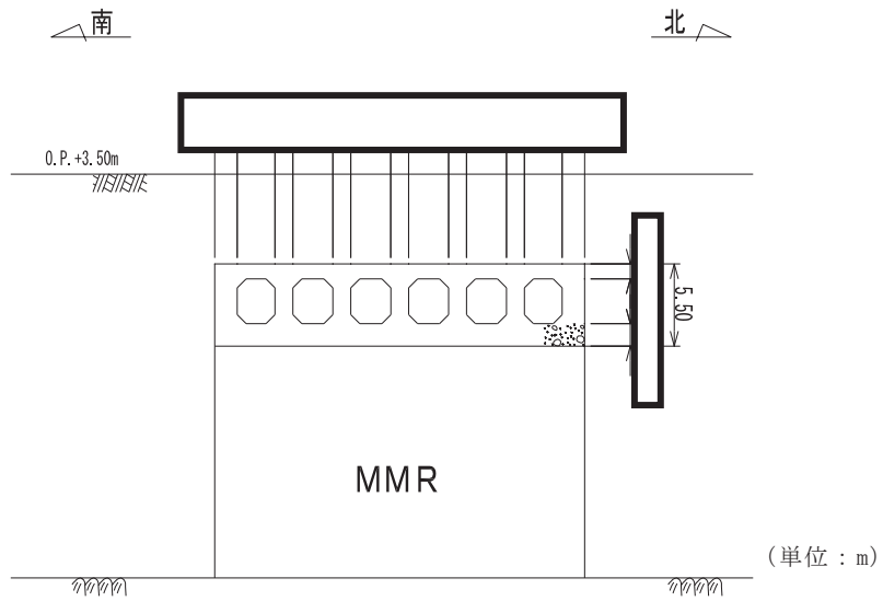
図11.2-8 取水口断面図 (B-B断面図, 漸縮部)
