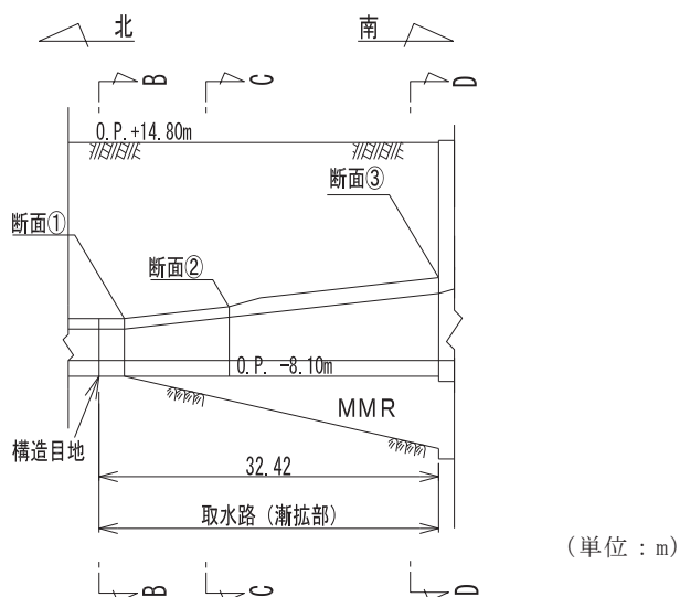
図 4.7-5 取水路（漸拡部）縦断図（A-A 断面）及び候補断面位置
