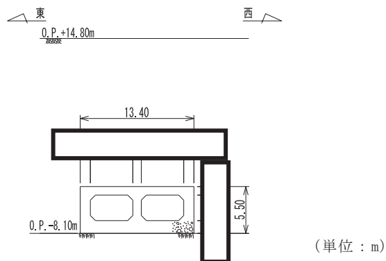
図 4.7-6 取水路（漸拡部）断面図（B-B 断面：断面①）
