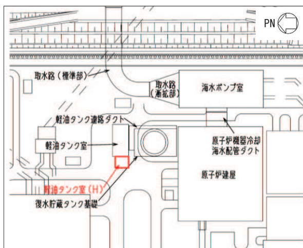
図 4.9-1 軽油タンク室 (H) 配置図
