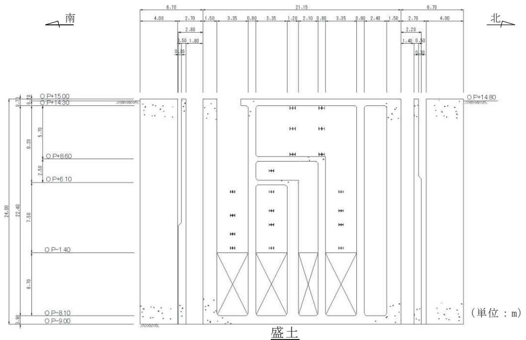
図 4.6-3 原子炉機器冷却海水配管ダクト（水平部）断面図（A-A 断面）
