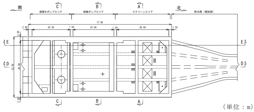
図 4.10-2 海水ポンプ室平面図
