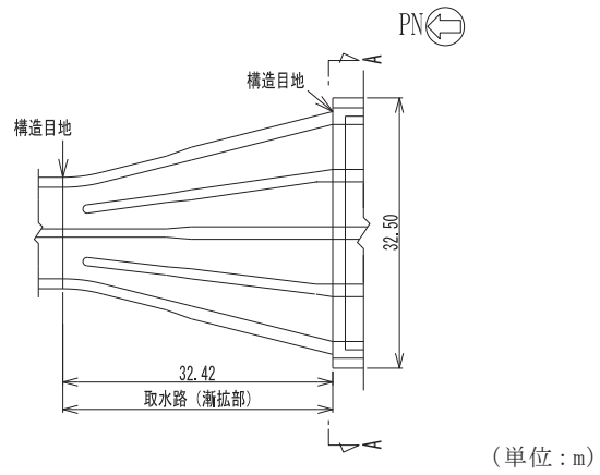
図 4.7-2 取水路（漸拡部）平面図
