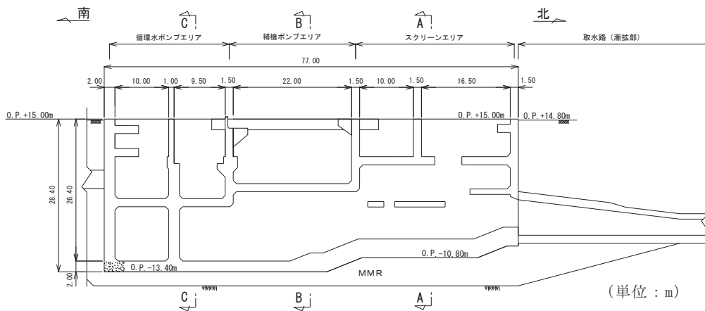
図 4.10-7 海水ポンプ室縦断面図 (E-E 断面, 南北)
