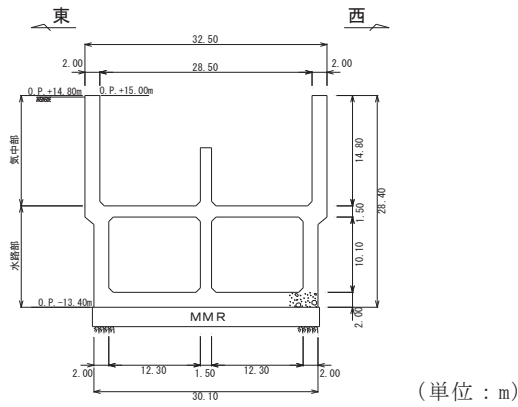
図 4.10-5 海水ポンプ室断面図 (C-C 断面, 東西 (循環水ポンプエリア))
