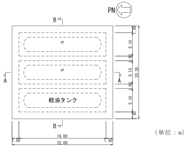
図 4.14-2 ガスタービン発電設備軽油タンク室平面図
