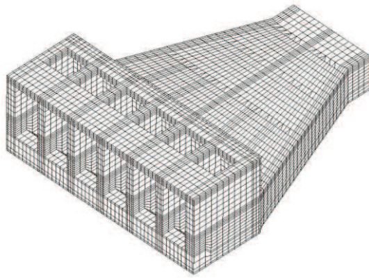
図 4.11-8 取水口，貯留堰 三次元モデル図
