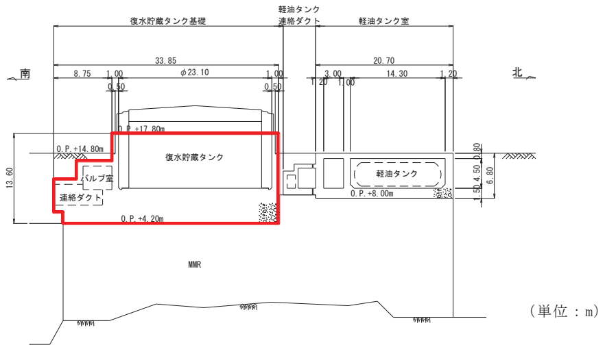
図 4.13-3 復水貯蔵タンク基礎断面図 (A-A 断面, 南北)
