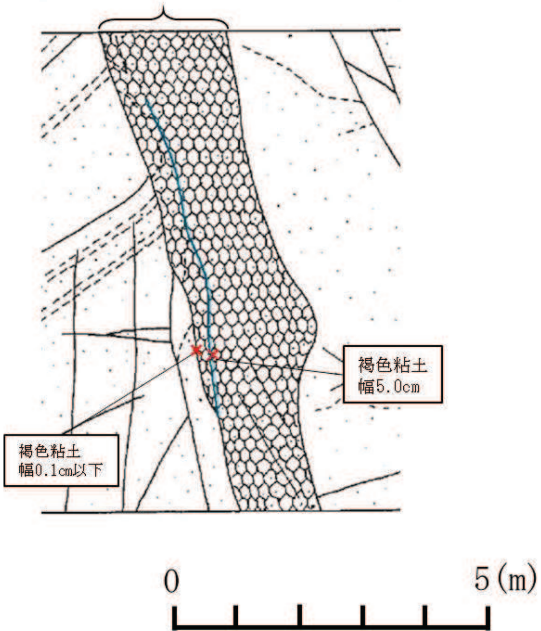
図1-3 排気筒連絡ダクト（土砂部） 底盤スケッチ（TF-1断層横断部）
