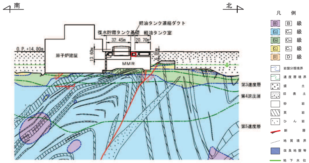
図 4.4-8 軽油タンク連絡ダクト地質断面図 (A-A 断面)
