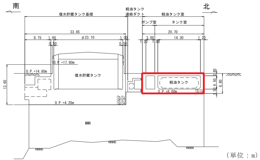
図 4.8-3 軽油タンク室断面図 (A-A 断面, 南北)
