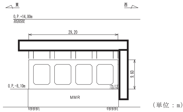
図 4.7-8 取水路（漸拡部）断面図（D-D 断面：断面③）
