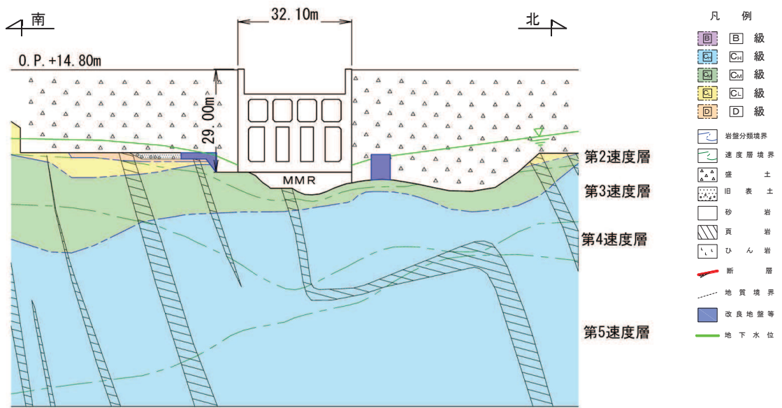
図 4.15-9 第 3 号機海水ポンプ室地質断面図 (B-B 断面)
