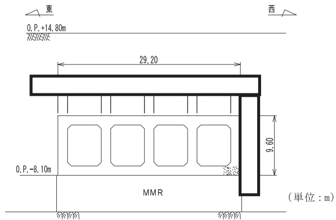
図 4.7-3 取水路（漸拡部）断面図（A-A 断面）
