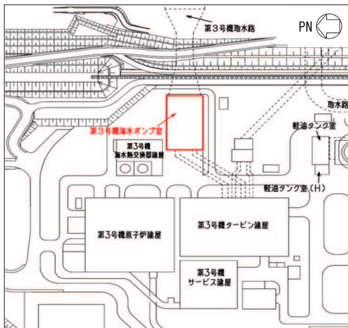
図4.15-1 第3号機海水ポンプ室配置図
