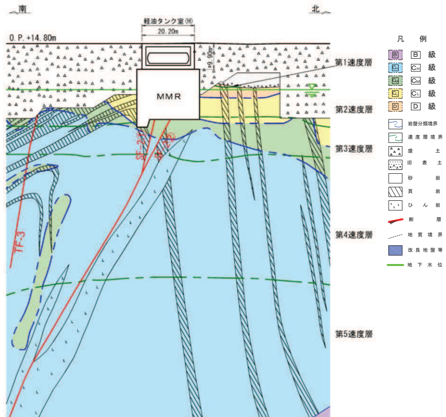
図 4.9-8 軽油タンク室 (H) 地質断面図 (B-B 断面)
