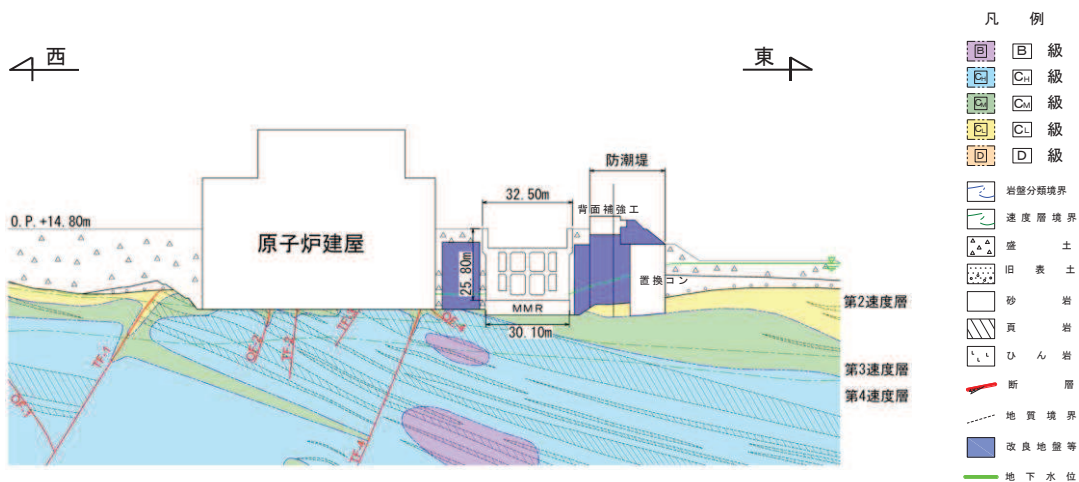
図 4.10-12(1) 海水ポンプ室 地震時荷重算出断面図（東西方向：スクリーンエリア）
