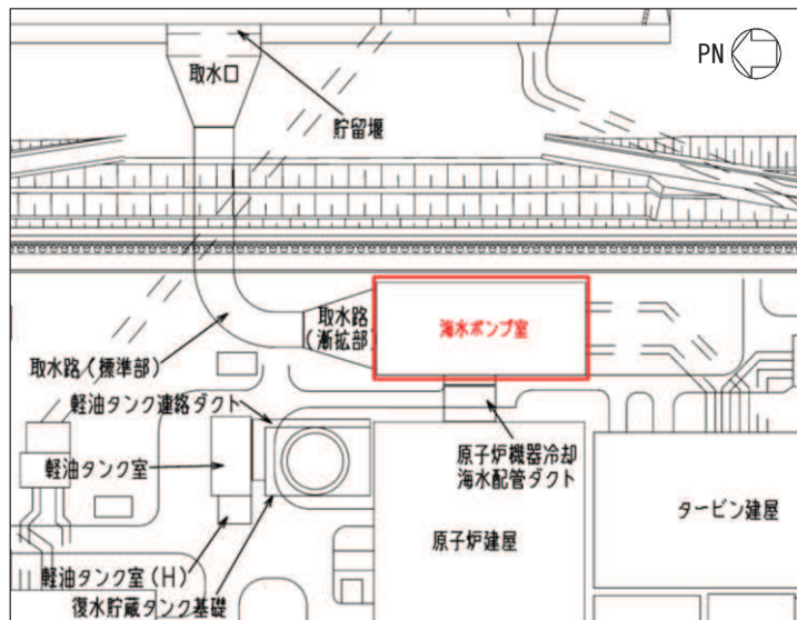
図 4.10-1 海水ポンプ室配置図
