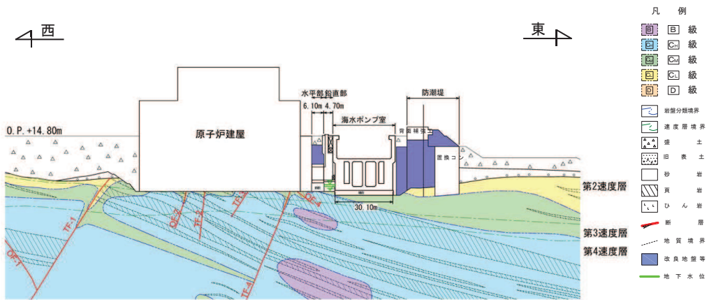
図 4.6-7 原子炉機器冷却海水配管ダクト（水平部）地質断面図（B-B 断面）
