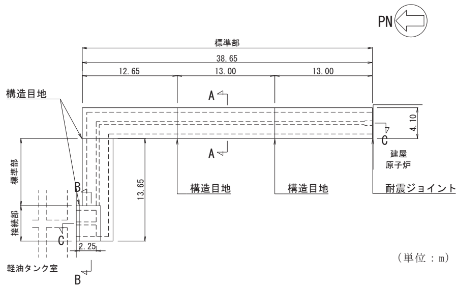
図 4.4-3 軽油タンク連絡ダクト平面図 (詳細)
