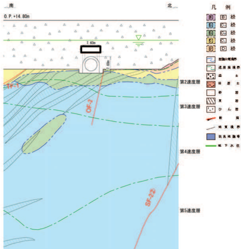
図 4.5-8 排気筒連絡ダクト（土砂部） 評価対象断面図（断面①）
