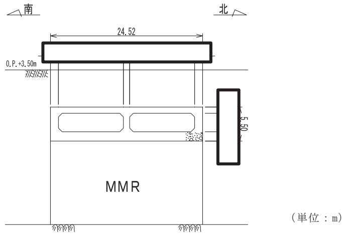
図 4.11-5 取水口断面図 (C-C 断面, 南北 (漸縮部))
