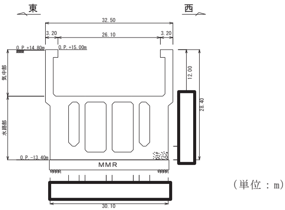
図 4.10-3 海水ポンプ室断面図 (A-A 断面, 東西 (スクリーンエリア))
