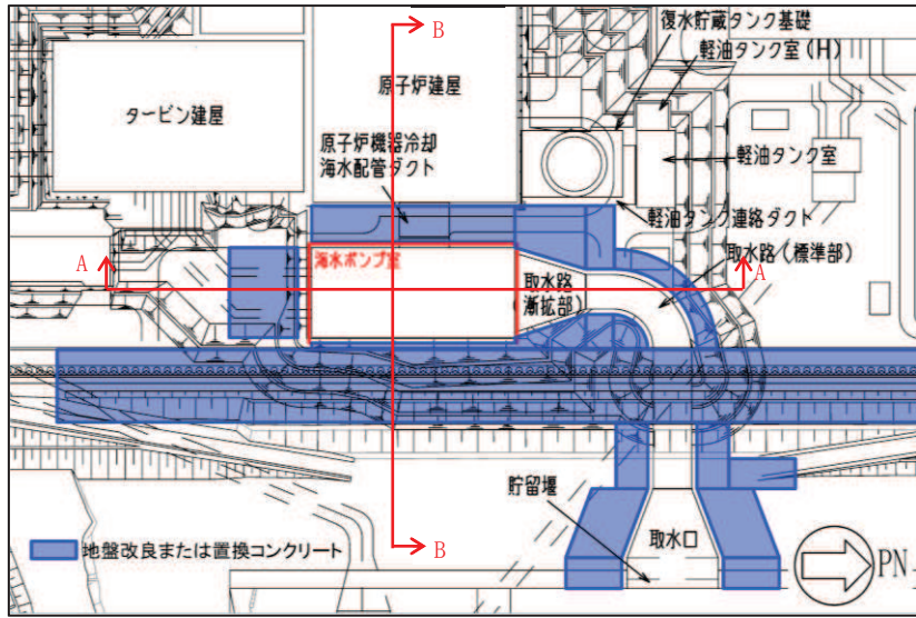
図 4.10-9 海水ポンプ室掘削図
