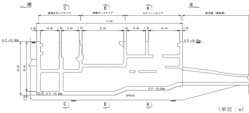
図 4.10-6 海水ポンプ室縦断面図 (D-D 断面, 南北)
