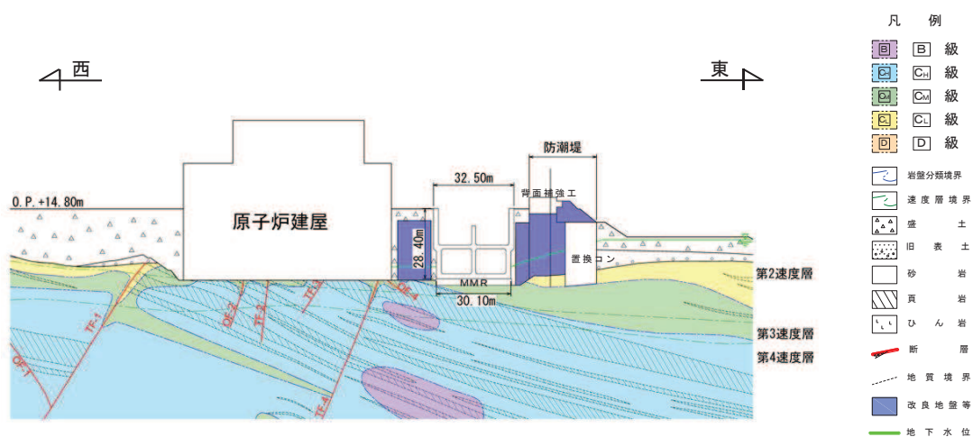
図 4.10-12(3) 海水ポンプ室 地震時荷重算出断面図（東西方向：循環水ポンプエリア）
