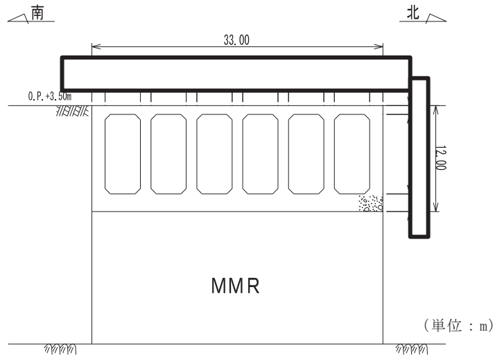
図 4.11-3 取水口断面図 (A-A 断面，南北 (標準部))
