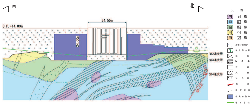
図 4.6-10 原子炉機器冷却海水配管ダクト（鉛直部）地質断面図（A-A 断面）
