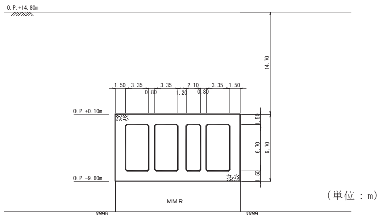
図 4.6-3 原子炉機器冷却海水配管ダクト（水平部）断面図（A-A 断面）
