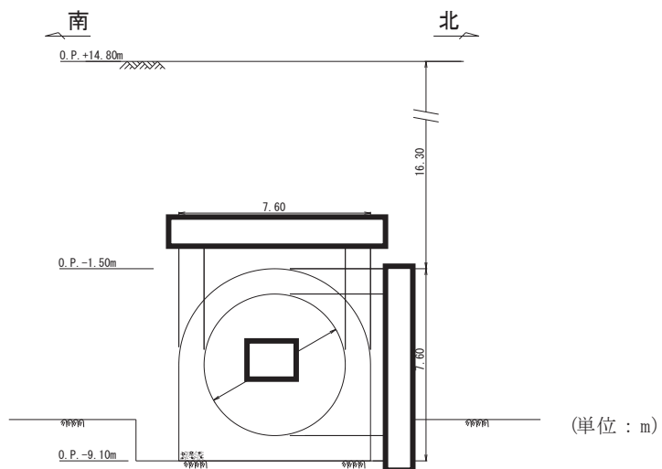
図 4.5-3 排気筒連絡ダクト断面図 (A-A 断面, 土砂部)
