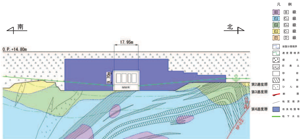
図 4.6-6 原子炉機器冷却海水配管ダクト（水平部）地質断面図（A-A 断面）
