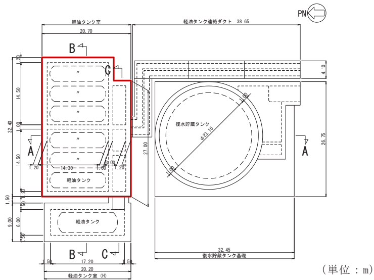
図 4.8-2 軽油タンク室平面図
