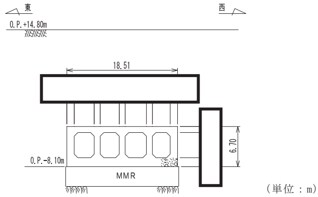
図 4.7-7 取水路（漸拡部）断面図（C-C 断面：断面②）
