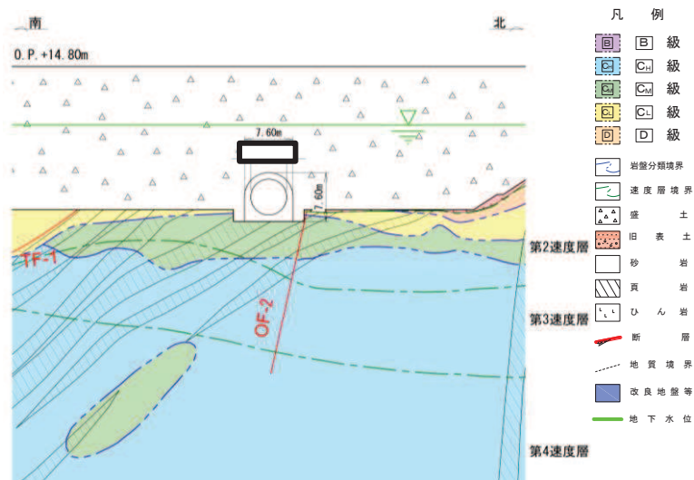
図 4.5-5 排気筒連絡ダクト (土砂部) 地質断面図 (A-A 断面)
