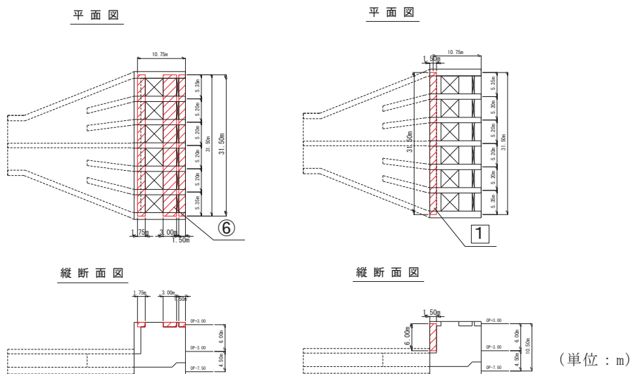
図11.2-10(3) 取水口（標準部）の等価剛性モデル（はり部材番号⑥，平面応力要素①）
