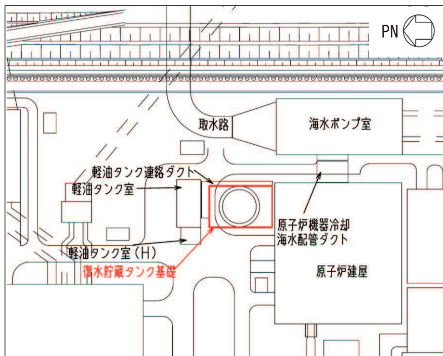
図 4.13-1 復水貯蔵タンク基礎配置図
