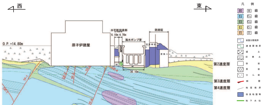
図 4.6-11 原子炉機器冷却海水配管ダクト（鉛直部）地質断面図（B-B 断面）
