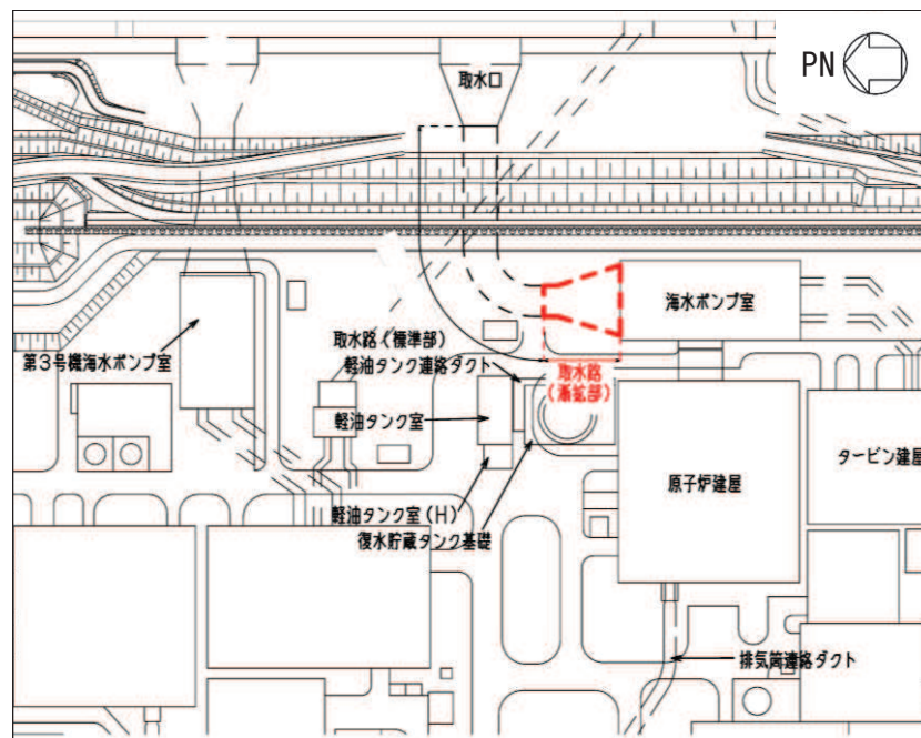
図 4.7-1 取水路（漸拡部）配置図
