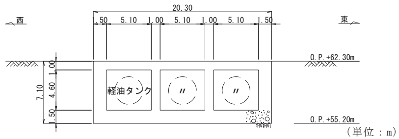
図 4.14-4 ガスタービン発電設備軽油タンク室断面図 (B-B 断面, 東西)
