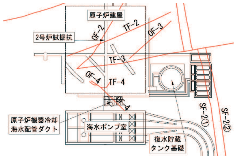
図 1-1 屋外重要土木構造物等の位置と主要断層の分布状況 (O.P. 約-14m)
