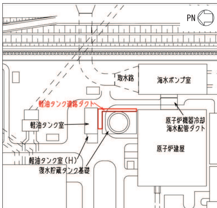
図 4.4-1 軽油タンク連絡ダクト配置図
