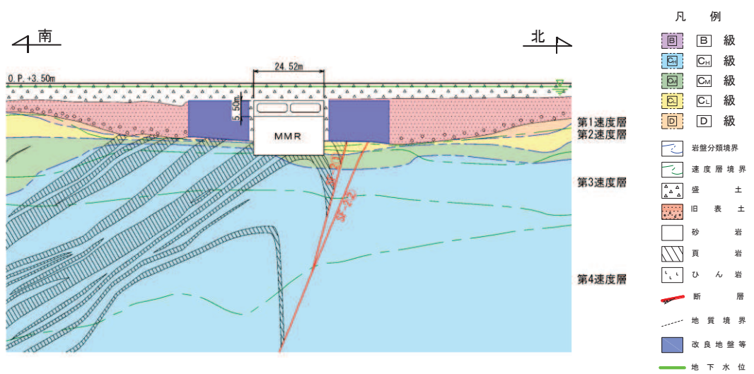
图 4.11-12 取水口地質断面图 (C-C 断面)
