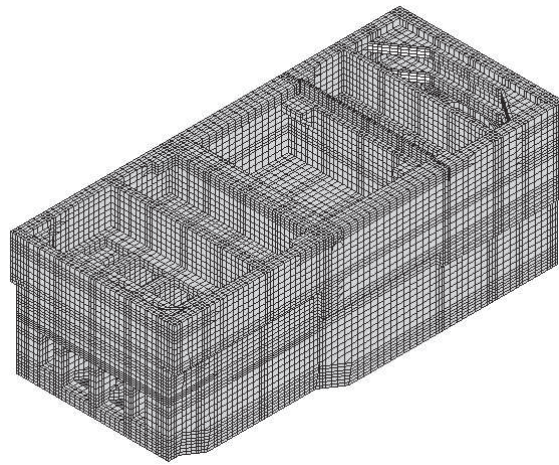
図 4.10-8 海水ポンプ室 三次元モデル図
