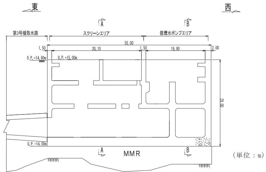
図 4.15-5 第3号機海水ポンプ室縦断図 (C-C 断面)
