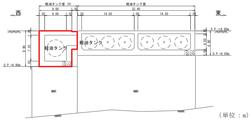
図 4.9-4 軽油タンク室 (H) 断面図 (B-B 断面, 東西)
