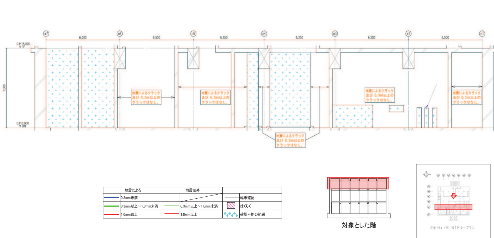
図 12 第 3 号機海水熱交換器建屋のひび割れ分布 耐震壁 (12) 地下 1 階 HE 通り
