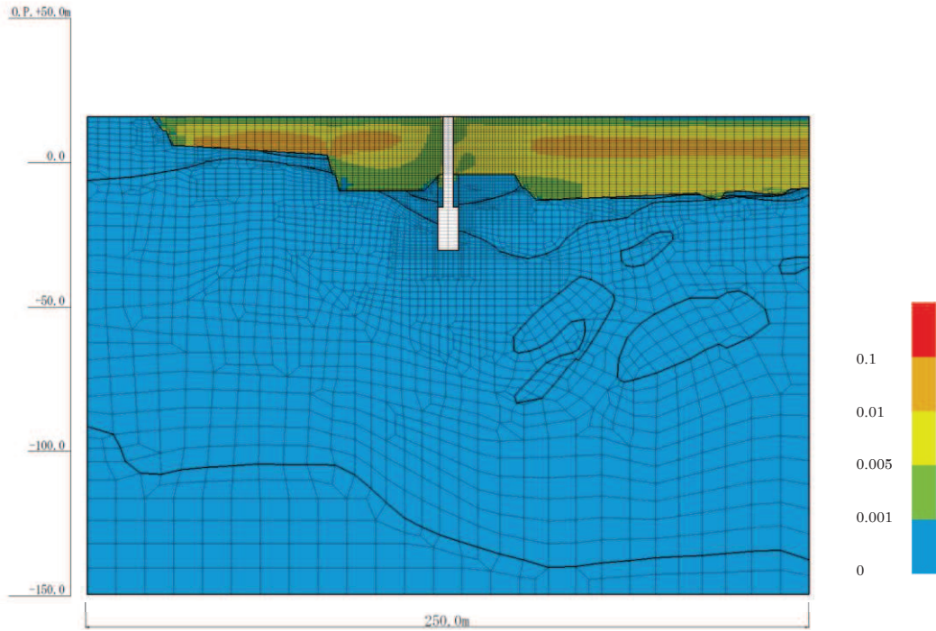
図 4-34(1) 最大せん断ひずみ分布 (No.1 揚水井戸, S s - N 1 ( - + ) , 解析ケース①) (全応力解析)
