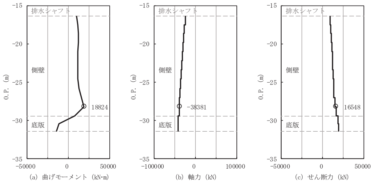
図 4-13(1) 集水ピット 軸方向照査におけるコンクリートの曲げ・軸力系の破壊に対する評価時刻での断面力 (No.1 揚水井戸, S s - N 1 (-+), 7.50s)
