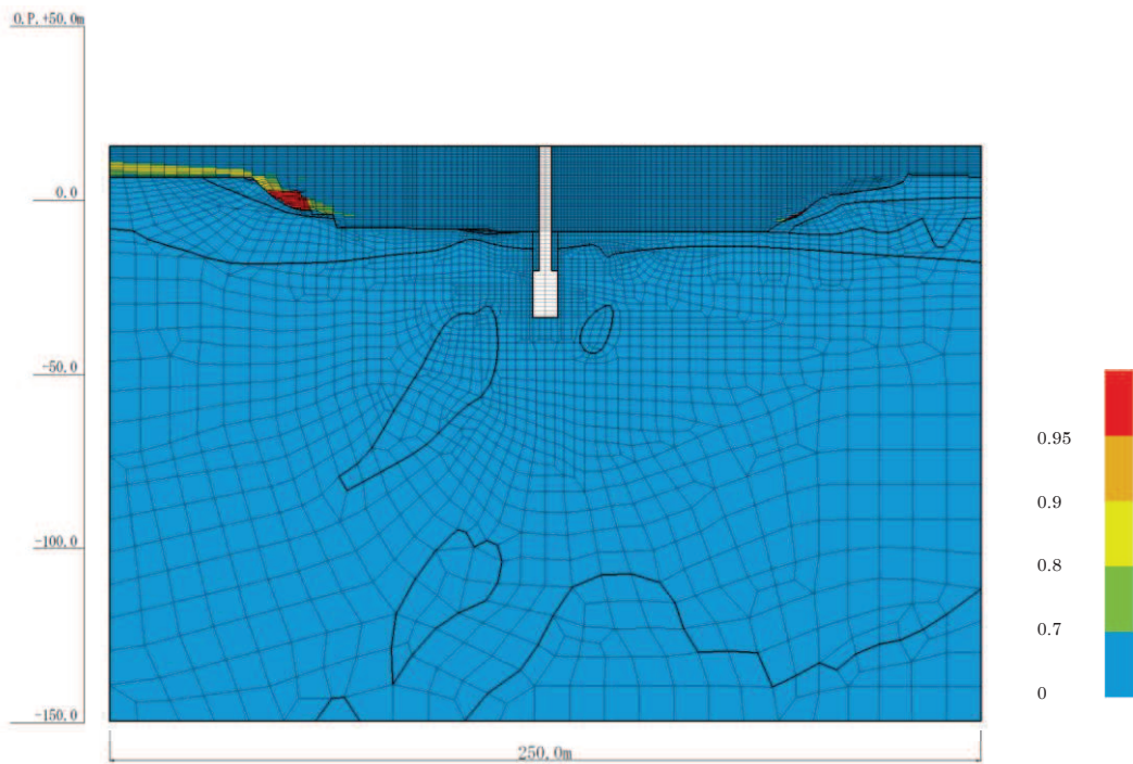
図 4-35(6) 最大過剰間隙水圧比分布 (No.2 揚水井戸, S_s - F1 (一十), 解析ケース③)
