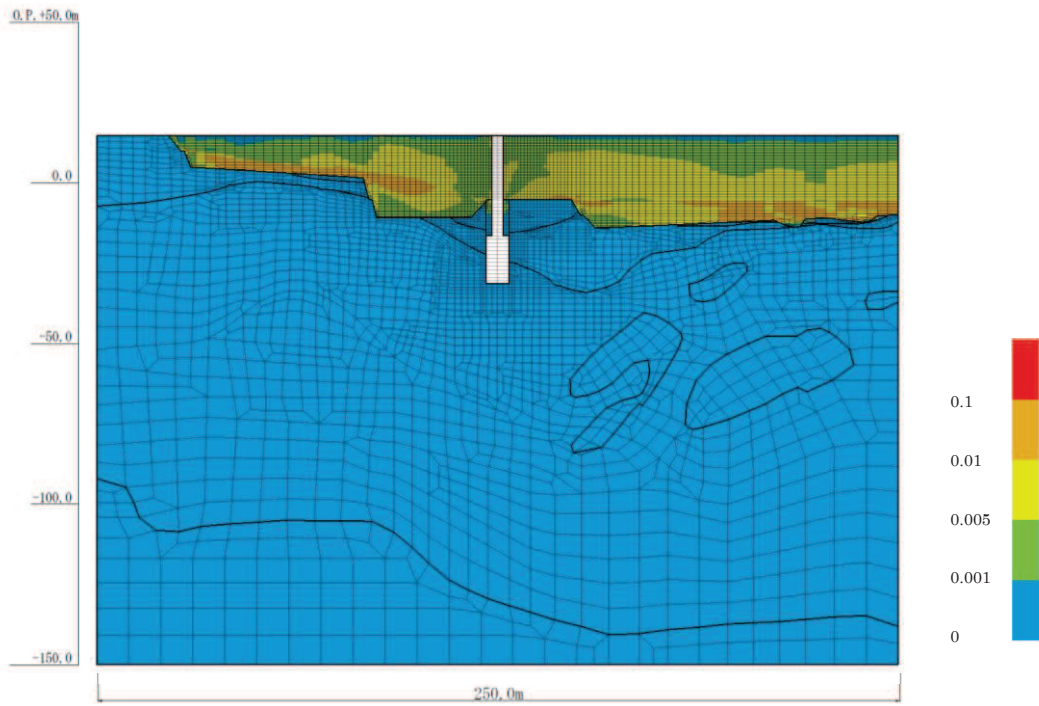
図 4-34(6) 最大せん断ひずみ分布 (No.1 揚水井戸, S s - N 1 ( - + ) , 解析ケース②) (有効応力解析)
