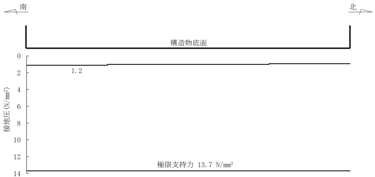
図 4-33(2) 最大接地圧分布図 (No. 1 揚水井戸, S s - D 1 ( - + ) , 解析ケース②) (有効応力解析)
