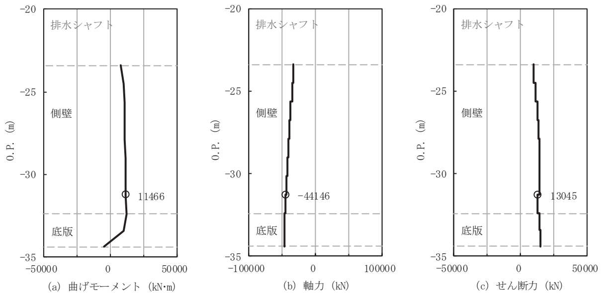
図 4-28(1) 集水ピット 軸方向照査におけるコンクリートの曲げ・軸力系の破壊に対する評価時刻での断面力 (No. 4 揚水井戸, S s - F 3 (++) , 27.63s) 解析ケース①：基本ケース (全応力解析)
