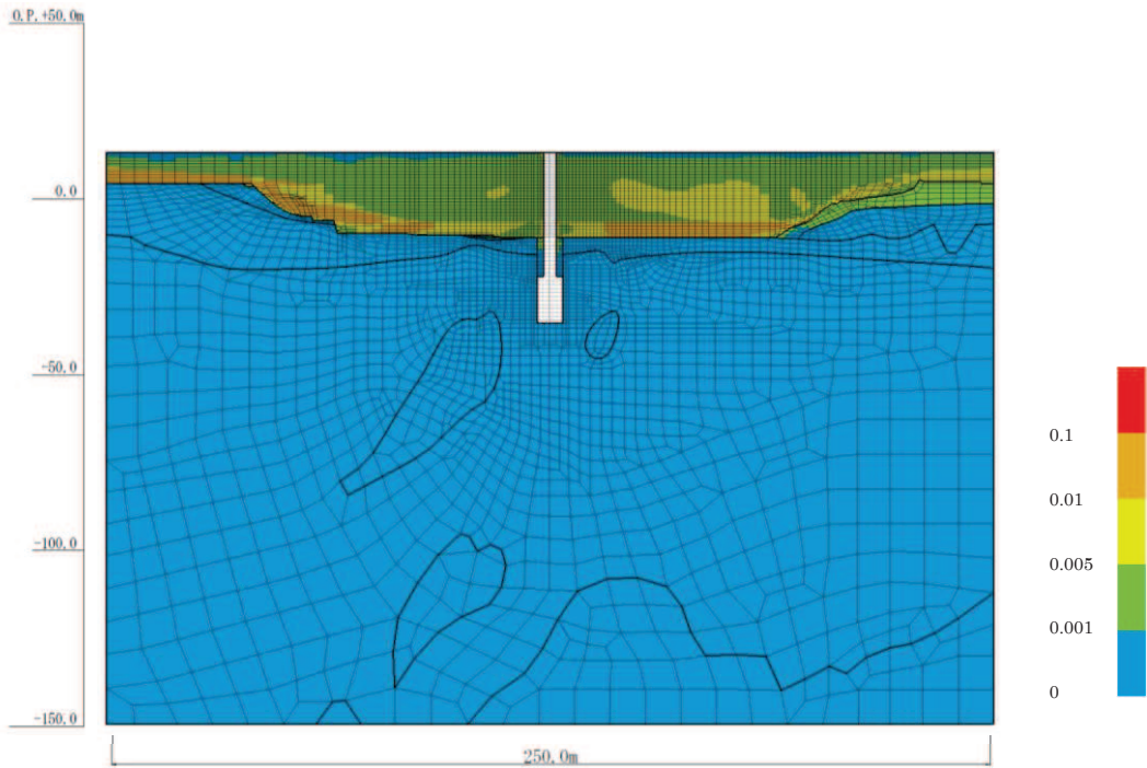
図 4-34(10) 最大せん断ひずみ分布 (No. 2 揚水井戸, S_s - F 1 (一+), 解析ケース②) (有効応力解析)
