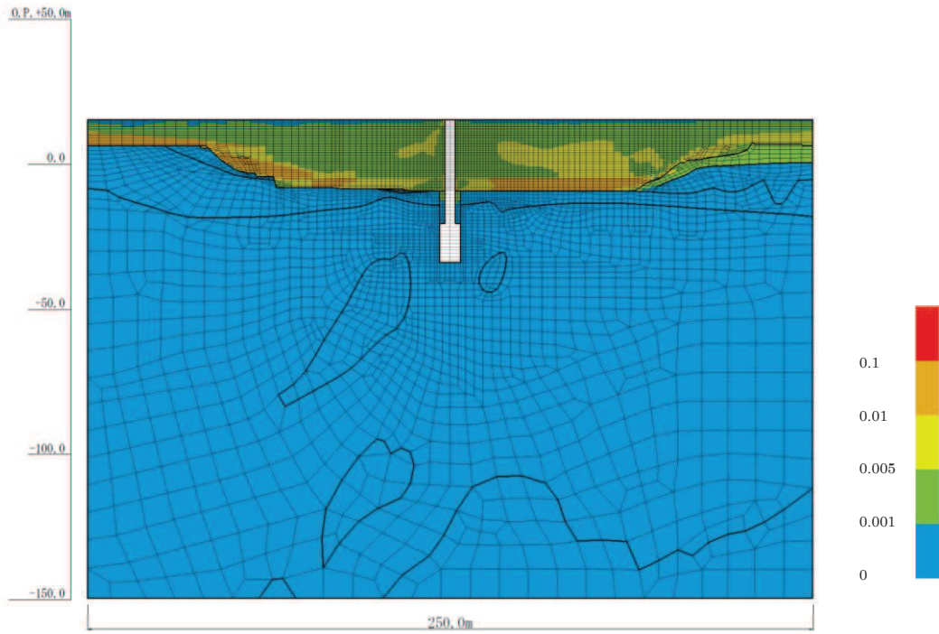
図 4-34(12) 最大せん断ひずみ分布 (No.2 揚水井戸, S s - F 1 ( - + ) , 解析ケース③) (有効応力解析)
