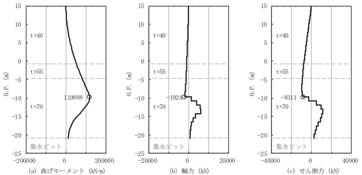
図 4-4(1) 排水シャフト 軸方向照査における曲げ・軸力系の破壊に対する評価時刻での断面力 (No.2 揚水井戸 (板厚 t=70 mm) , S s -N1 (++) , 7.78s)
