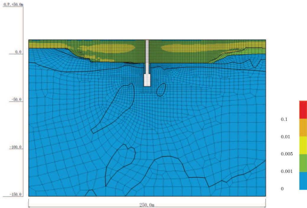
図 4-34(7) 最大せん断ひずみ分布 (No.2 揚水井戸, S s - D 2 (++) , 解析ケース①) (全応力解析)
