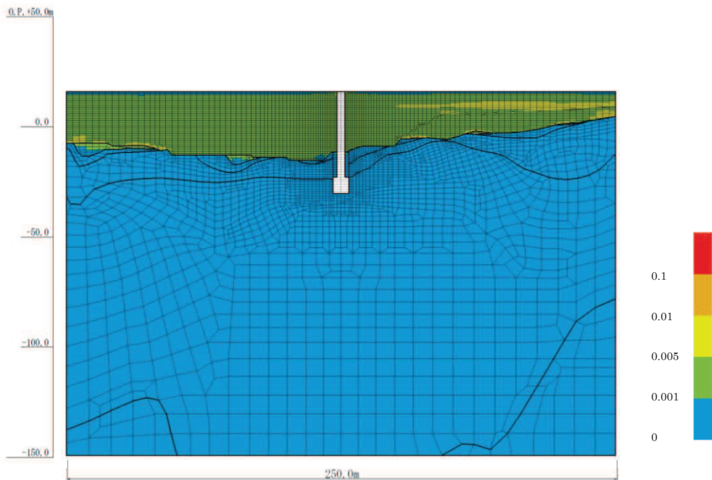
図 4-34(14) 最大せん断ひずみ分布 (No. 3 揚水井戸, S s - D 3 (++) , 解析ケース②) (全応力解析)
