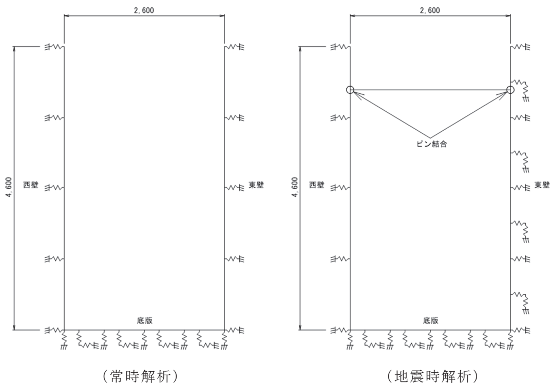
図 2-2 フレームモデル（単位：mm）
