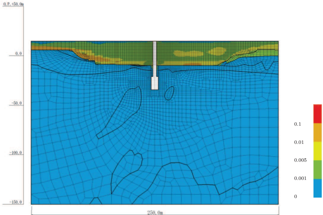
図 4-34(11) 最大せん断ひずみ分布 (No. 2 揚水井戸, S_s - D 2 (++) , 解析ケース②) (有効応力解析)
