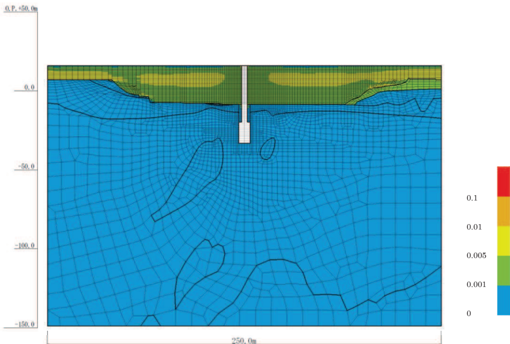
図 4-34(8) 最大せん断ひずみ分布 (No.2 揚水井戸, S s - D 2 (-+) , 解析ケース①) (全応力解析)
