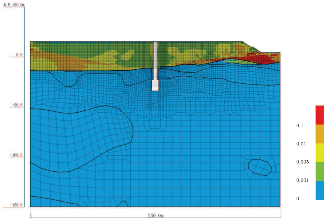
図 4-34(23) 最大せん断ひずみ分布 (No. 4 揚水井戸, S s - D 1 (++) , 解析ケース③) (有効応力解析)
