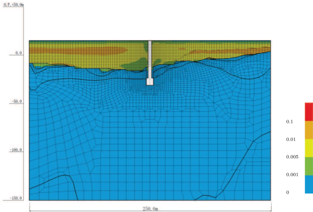
図 4-34(15) 最大せん断ひずみ分布 (No.3 揚水井戸, S s - N 1 ( - + ) , 解析ケース①) (全応力解析)
