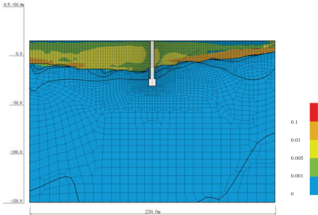
図 4-34(16) 最大せん断ひずみ分布 (No. 3 揚水井戸, S s - N 1 (++) , 解析ケース②) (有効応力解析)
