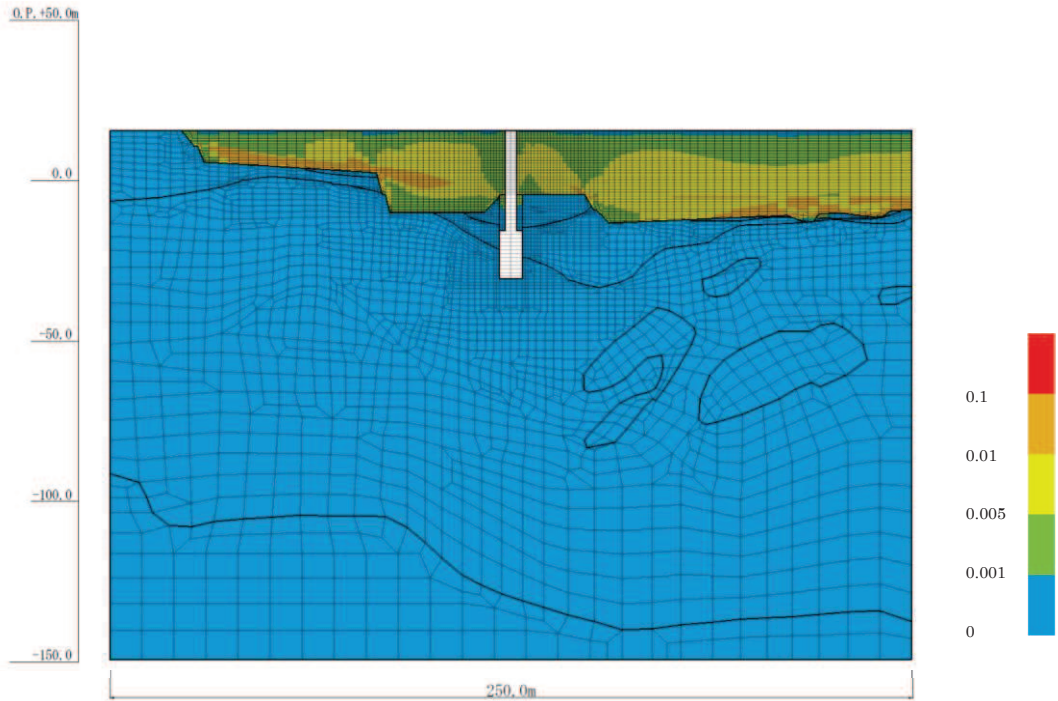
図 4-34(4) 最大せん断ひずみ分布 (No.1 揚水井戸, S s -N1 (++) , 解析ケース②) (有効応力解析)
