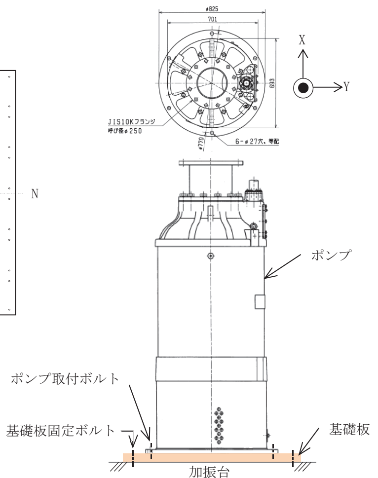
図 2-2 加振台の取付状態
