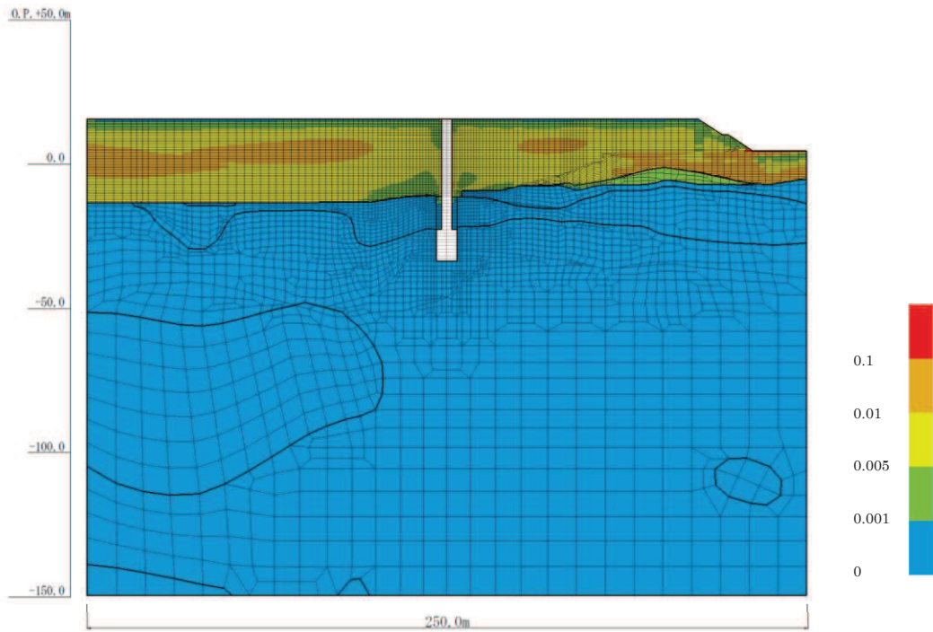
図 4-34(19) 最大せん断ひずみ分布 (No. 4 揚水井戸, S s - N 1 ( - + ) , 解析ケース①) (全応力解析)
