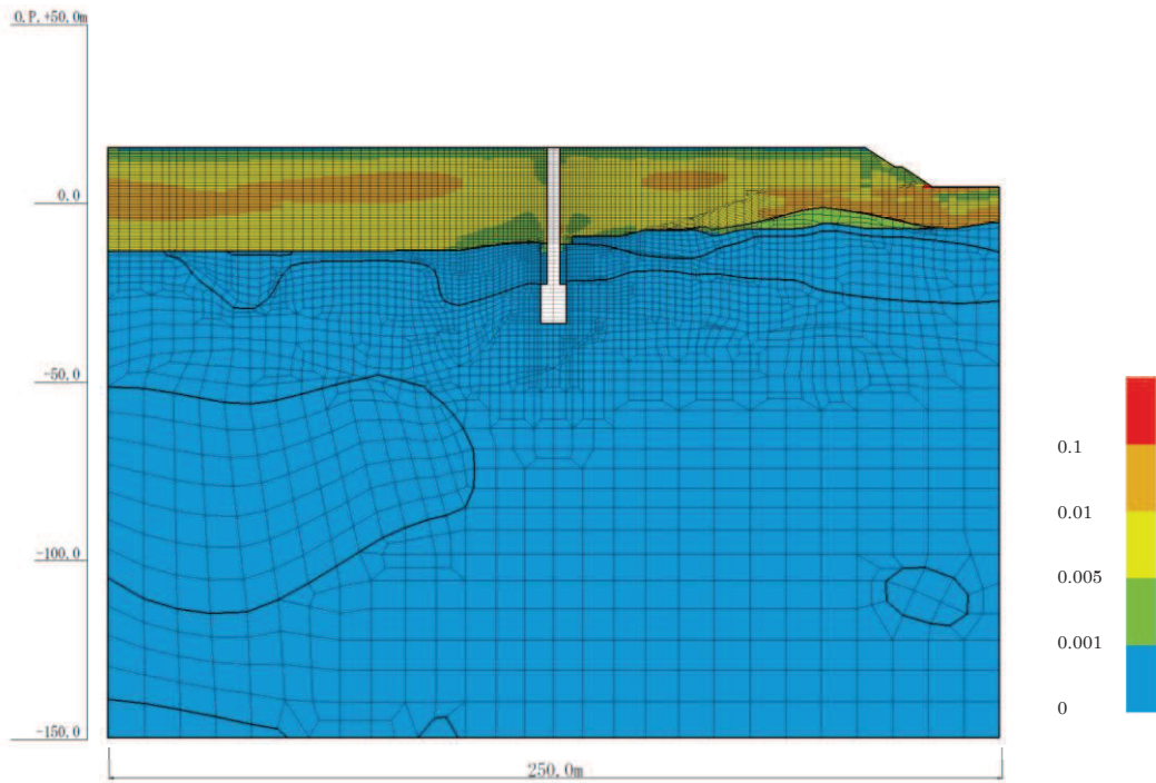
図 4-34(21) 最大せん断ひずみ分布 (No. 4 揚水井戸, S s - N 1 ( - + ) , 解析ケース①) (全応力解析)
