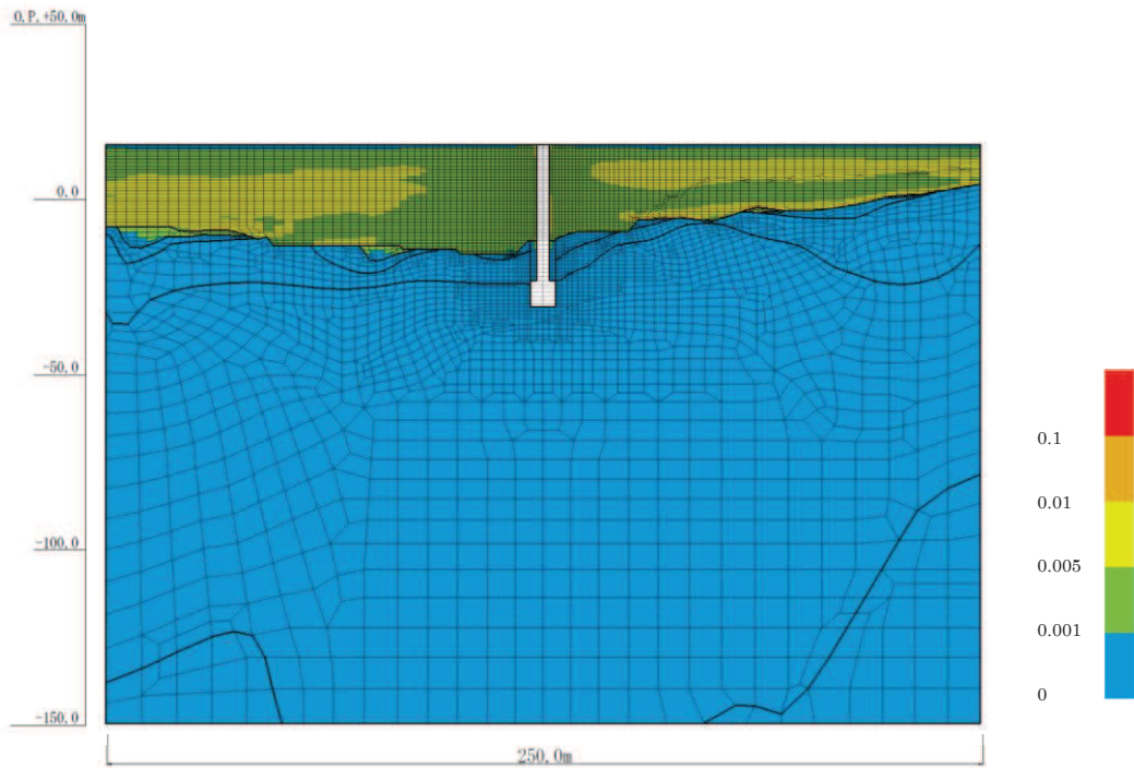
図 4-34(13) 最大せん断ひずみ分布 (No. 3 揚水井戸, S s - D 2 (一+), 解析ケース②) (全応力解析)
