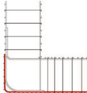
断面図
