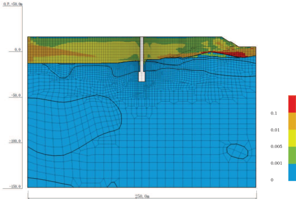
図 4-34(22) 最大せん断ひずみ分布 (No. 4 揚水井戸, S s - N 1 (++) , 解析ケース②) (有効応力解析)
