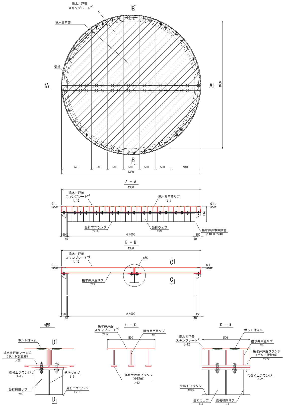
図 3-1(1) 評価対象部位 (No. 1, No. 2 揚水井戸蓋) (単位: mm)
