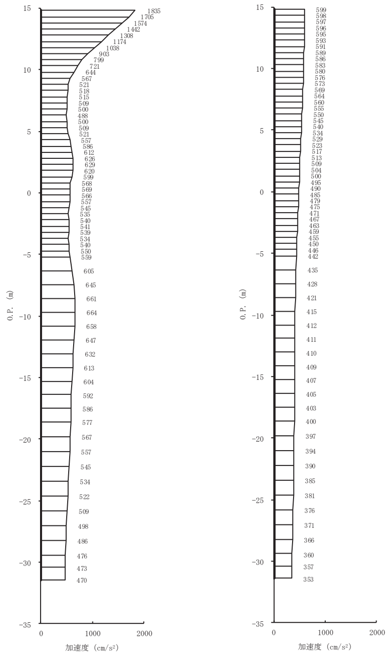
(a) S s - D 2 (++) 水平 (b) S s - D 2 (++) 鉛直 図 1-1(2) 最大加速度分布図 (2/7) (No. 1 揚水井戸)
