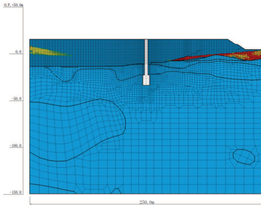
図 4-35(12) 最大過剰間隙水圧比分布 (No.4 揚水井戸, S_s - D 1 (++) , 解析ケース②)
