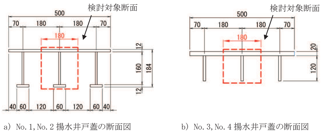
図 5-2 断面力算定区間及び断面計算の検討断面 (単位: mm)
