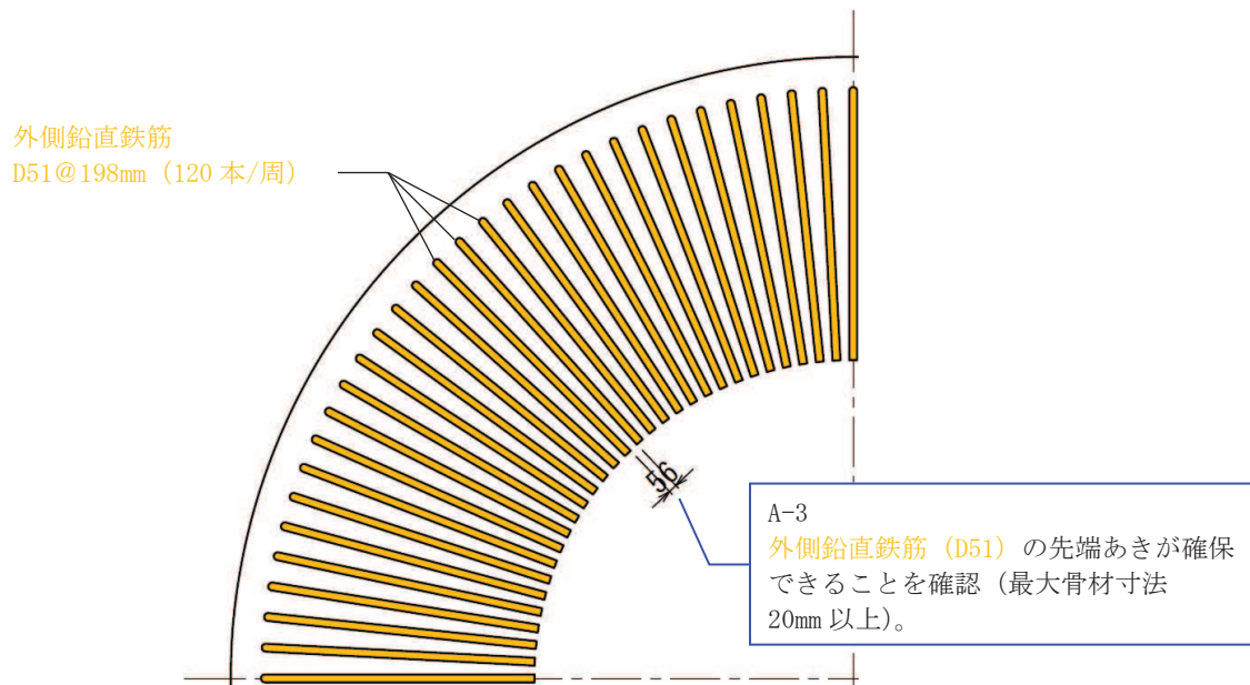
図 3 (3) 配筋上の留意点に対する対応内容 (その 3) (単位 : mm)
