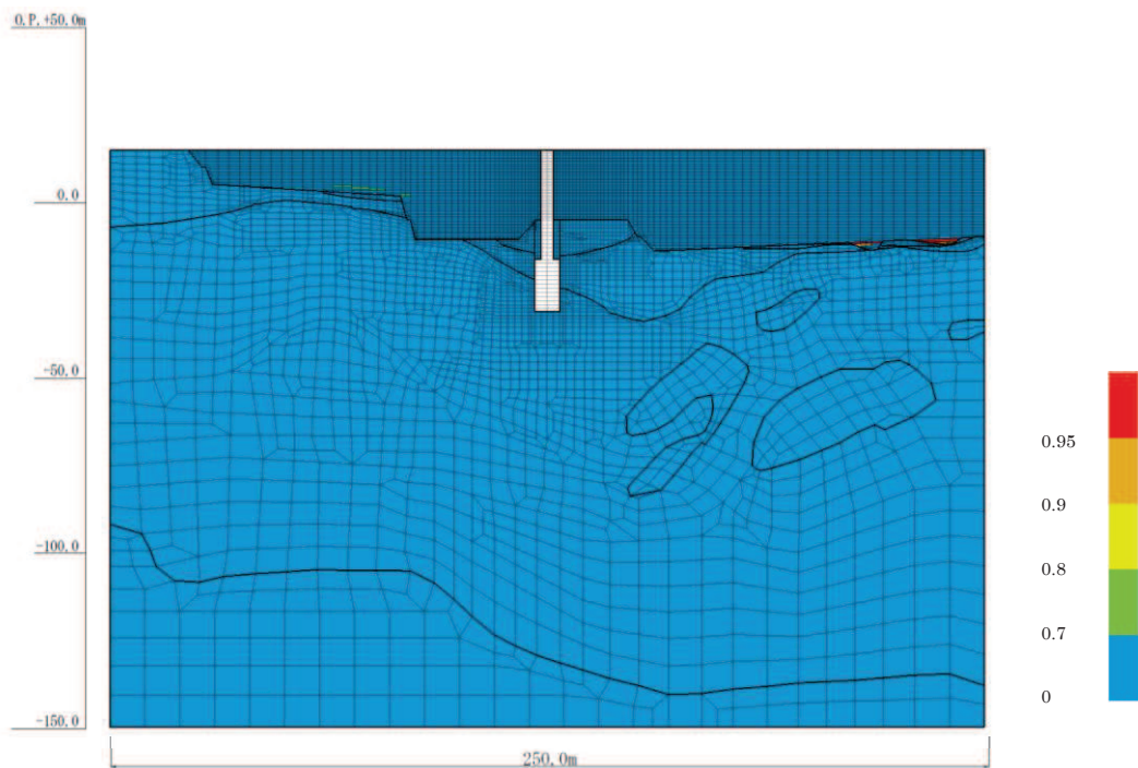
図 4-35(1) 最大過剰間隙水圧比分布 (No.1 揚水井戸, S_s - N1 (++) , 解析ケース②)
