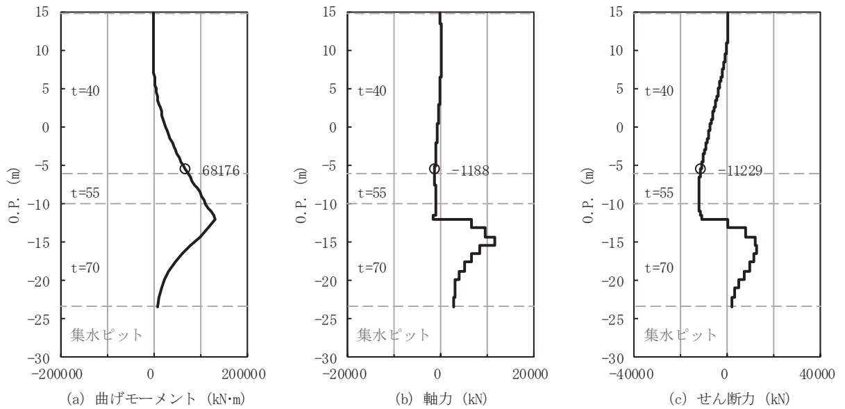
図 4-11(2) 排水シャフト 軸方向照査におけるせん断破壊に対する評価時刻での断面力 (No. 4 揚水井戸 (板厚 t=40 mm) , S s - N 1 (++) , 7.81s)
