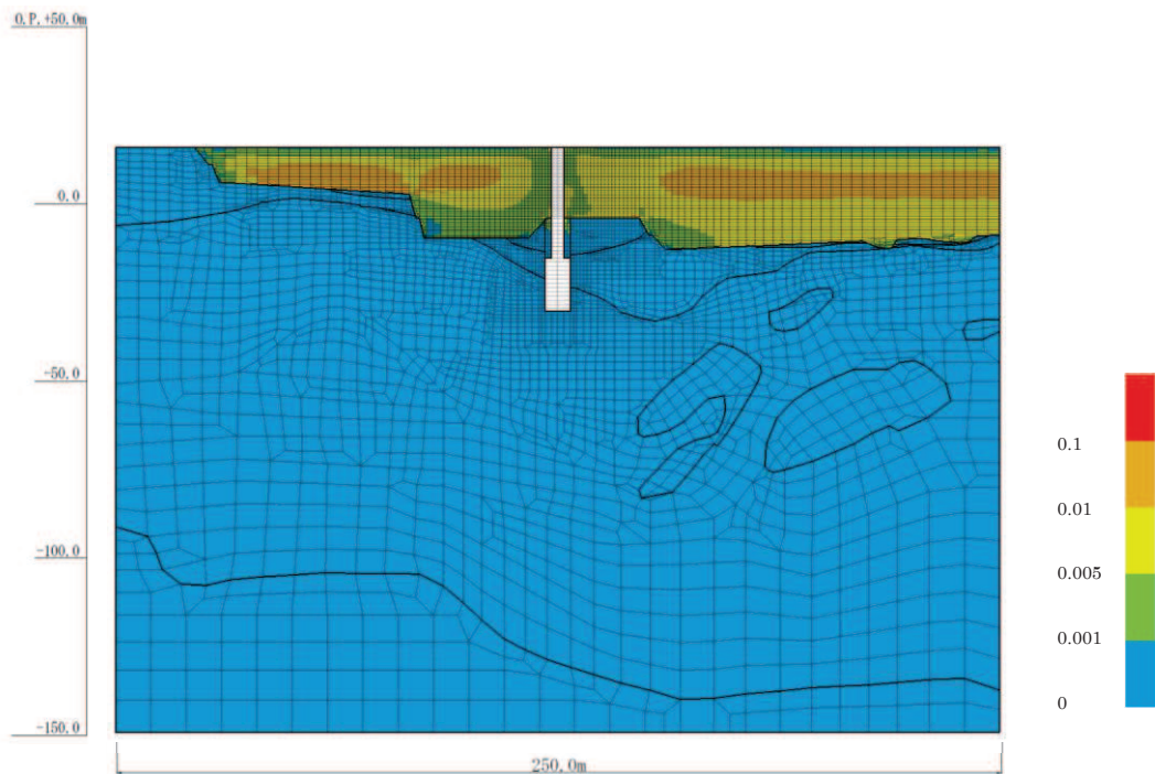
図 4-34(2) 最大せん断ひずみ分布 (No.1 揚水井戸, S s - N 1 ( + + ) , 解析ケース③) (全応力解析)
