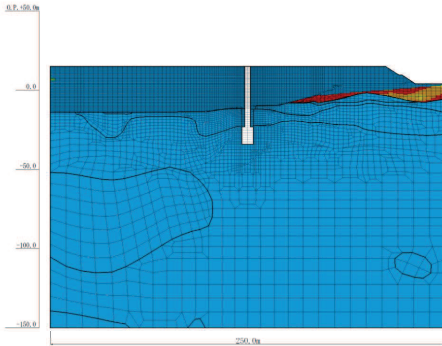
図 4-35(10) 最大過剰間隙水圧比分布 (No.4 揚水井戸, S s -N1 (++) , 解析ケース②)
