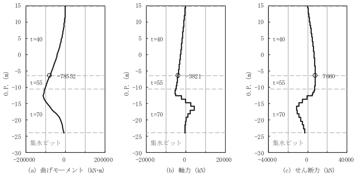
図 4-7(1) 排水シャフト 軸方向照査における曲げ・軸力系の破壊に対する評価時刻での断面力 (No.3 揚水井戸 (板厚 t=40\text{mm} ) , S s -N1 (-+), 7.83s) 解析ケース①：基本ケース (全応力解析)
