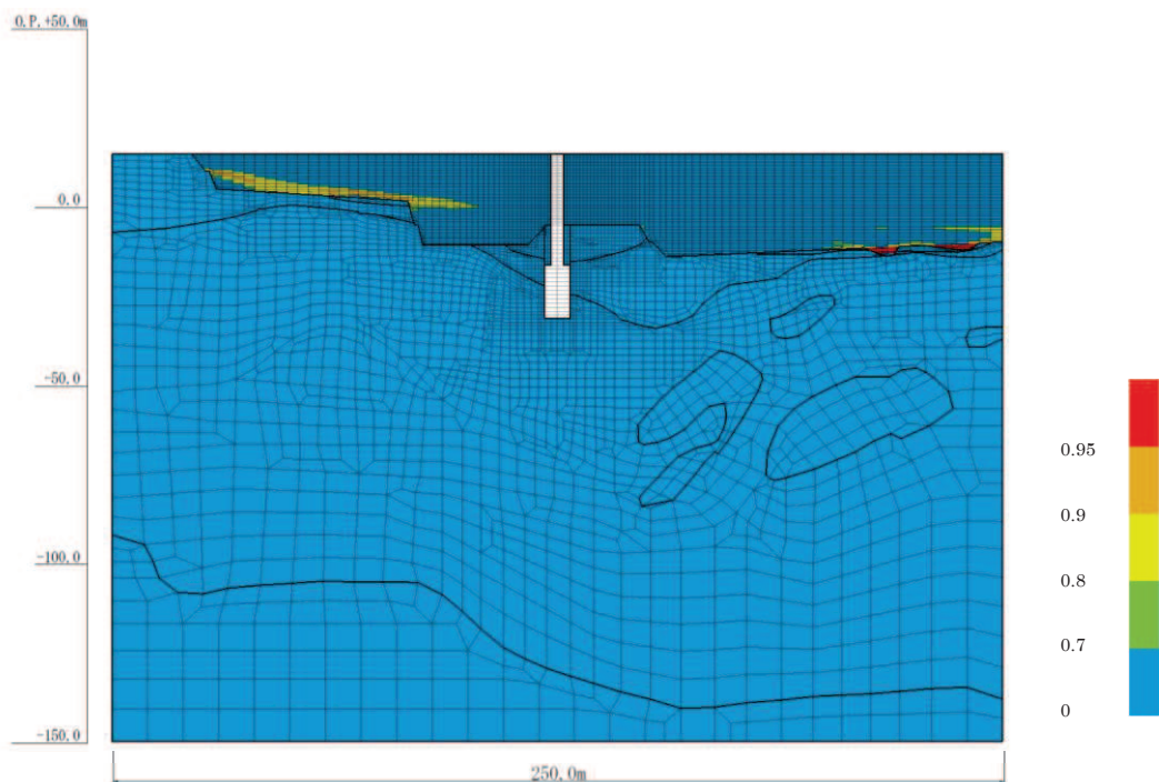
図 4-35(2) 最大過剰間隙水圧比分布 (No.1 揚水井戸, S_s - D1 (-+) , 解析ケース①)
