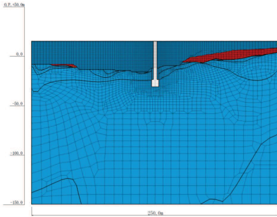
図 4-35(7) 最大過剰間隙水圧比分布 (No.3 揚水井戸, S s -N1 (++) , 解析ケース②)
