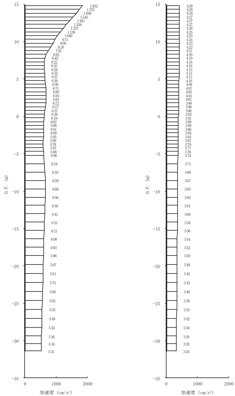
(a) S s -F 2 (++) 水平 (b) S s -F 2 (++) 鉛直 図 1-1(5) 最大加速度分布図 (5/7) (No. 1 揚水井戸)
