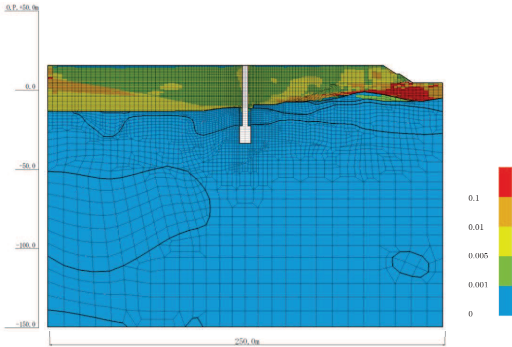
図 4-34(24) 最大せん断ひずみ分布 (No. 4 揚水井戸, S s - D 1 (++) , 解析ケース②) (有効応力解析)
