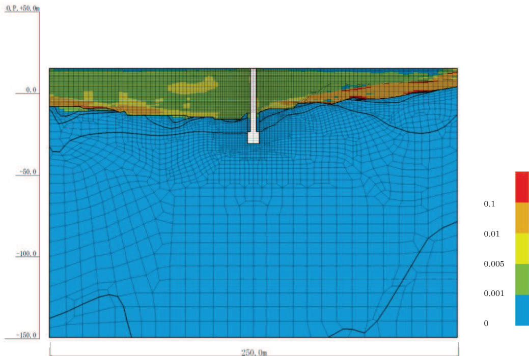
図 4-34(17) 最大せん断ひずみ分布 (No. 3 揚水井戸, S s - D 1 (-+) , 解析ケース①) (有効応力解析)
