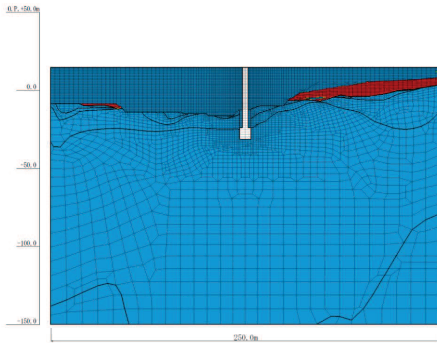
図 4-35(9) 最大過剰間隙水圧比分布 (No.3 揚水井戸, S_s - N1 (一十), 解析ケース①)
