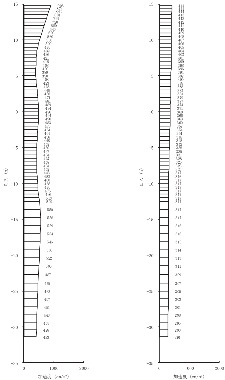
(a) S s -F 1 (++) 水平 (b) S s -F 1 (++) 鉛直 図 1-3(4) 最大加速度分布図 (4/7) (No. 3 揚水井戸)
