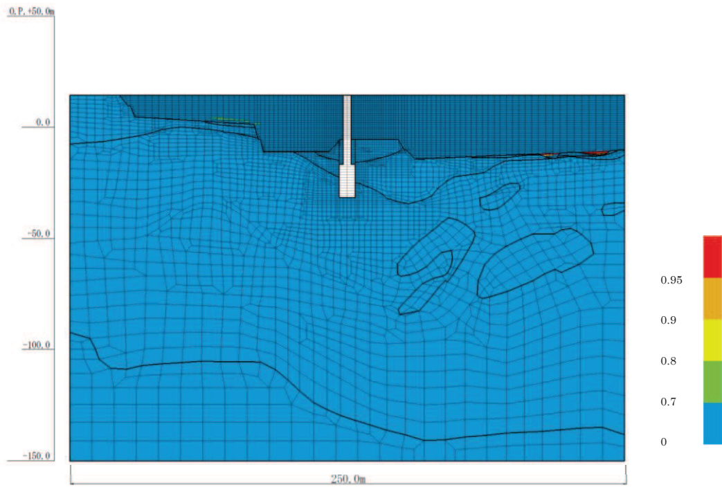
図 4-35(3) 最大過剰間隙水圧比分布 (No.1 揚水井戸, S_s - N1 (一十), 解析ケース②)
