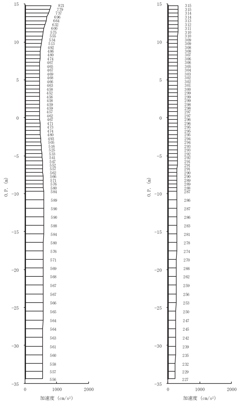
(a) S s - N 1 (++) 水平 (b) S s - N 1 (++) 鉛直 図 1-2(7) 最大加速度分布図 (7/7) (No. 2 揚水井戸)
