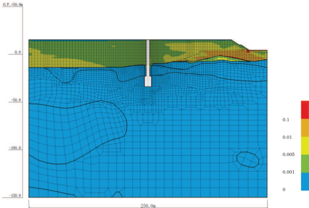
図 4-34(20) 最大せん断ひずみ分布 (No. 4 揚水井戸, S s - D 2 ( - + ) , 解析ケース③) (全応力解析)
