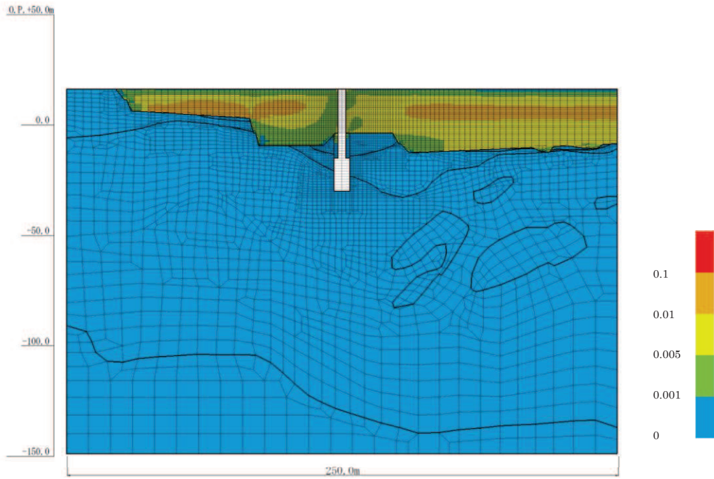
図 4-34(3) 最大せん断ひずみ分布 (No.1 揚水井戸, S s - N 1 (一+), 解析ケース②) (全応力解析)
