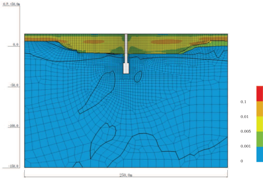
図 4-34(9) 最大せん断ひずみ分布 (No.2 揚水井戸, S s - N 1 (一+), 解析ケース①) (全応力解析)
