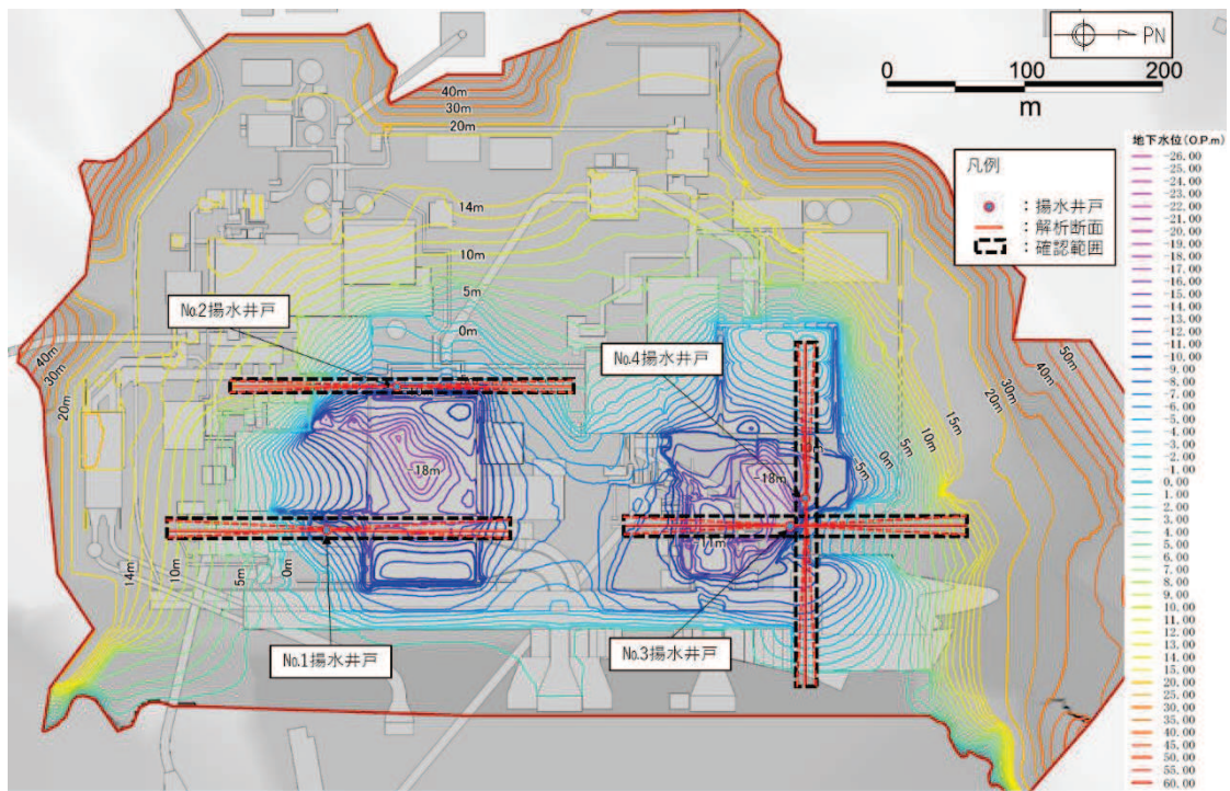
図 1-4 地下水位分布 (解析結果 包絡水位)
