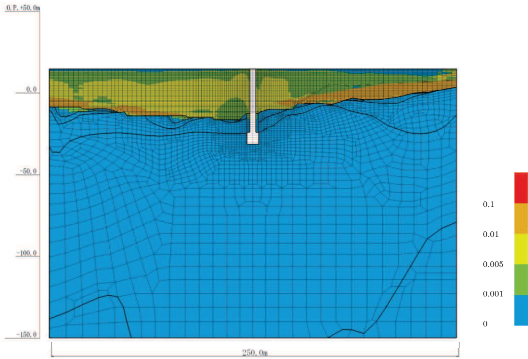
図 4-34(18) 最大せん断ひずみ分布 (No. 3 揚水井戸, S s - N 1 ( - + ) , 解析ケース①) (有効応力解析)
