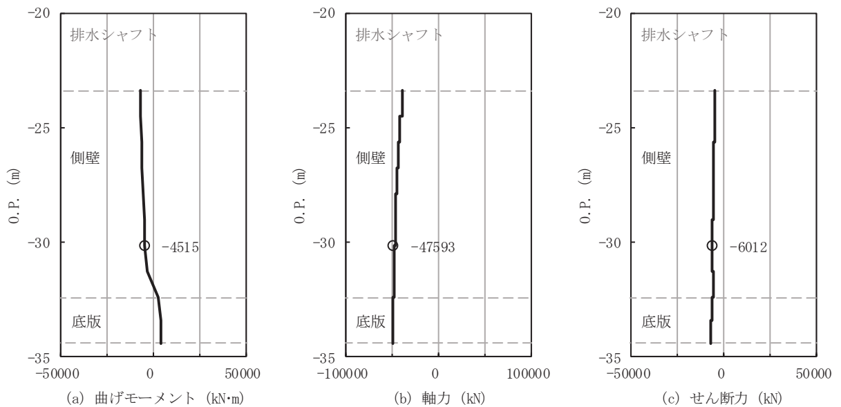
図 4-28(2) 集水ピット 軸方向照査におけるコンクリートの曲げ・軸力系の破壊に対する 評価時刻での断面力 (No. 4 揚水井戸, S s - D 1 (-+), 31.33s)
