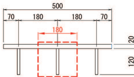
図 5-7(2) 断面力算定区間及び断面計算の検討断面 (No. 3, No. 4 揚水井戸蓋) (単位 : mm)
