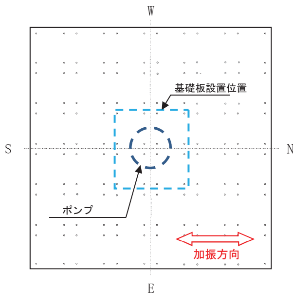
図 2-1 加振台（平面図）
