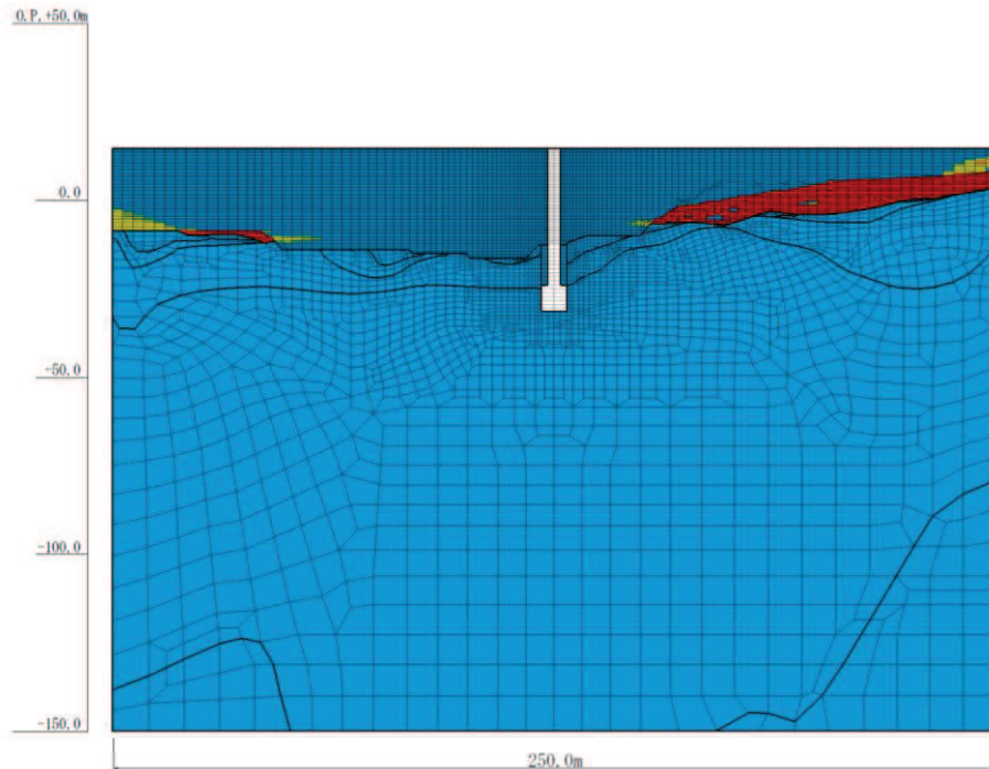
図 4-35(8) 最大過剰間隙水圧比分布 (No.3 揚水井戸, S s -D1 (-+) , 解析ケース①)
