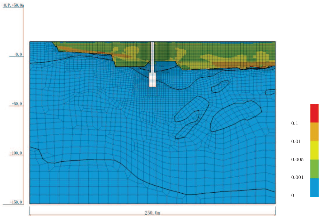
図 4-34(5) 最大せん断ひずみ分布 (No.1 揚水井戸, S s -D1 (-+) , 解析ケース①) (有効応力解析)
