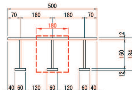
図 5-7(1) 断面力算定区間及び断面計算の検討断面 (No. 1, No. 2 揚水井戸蓋) (単位 : mm)
