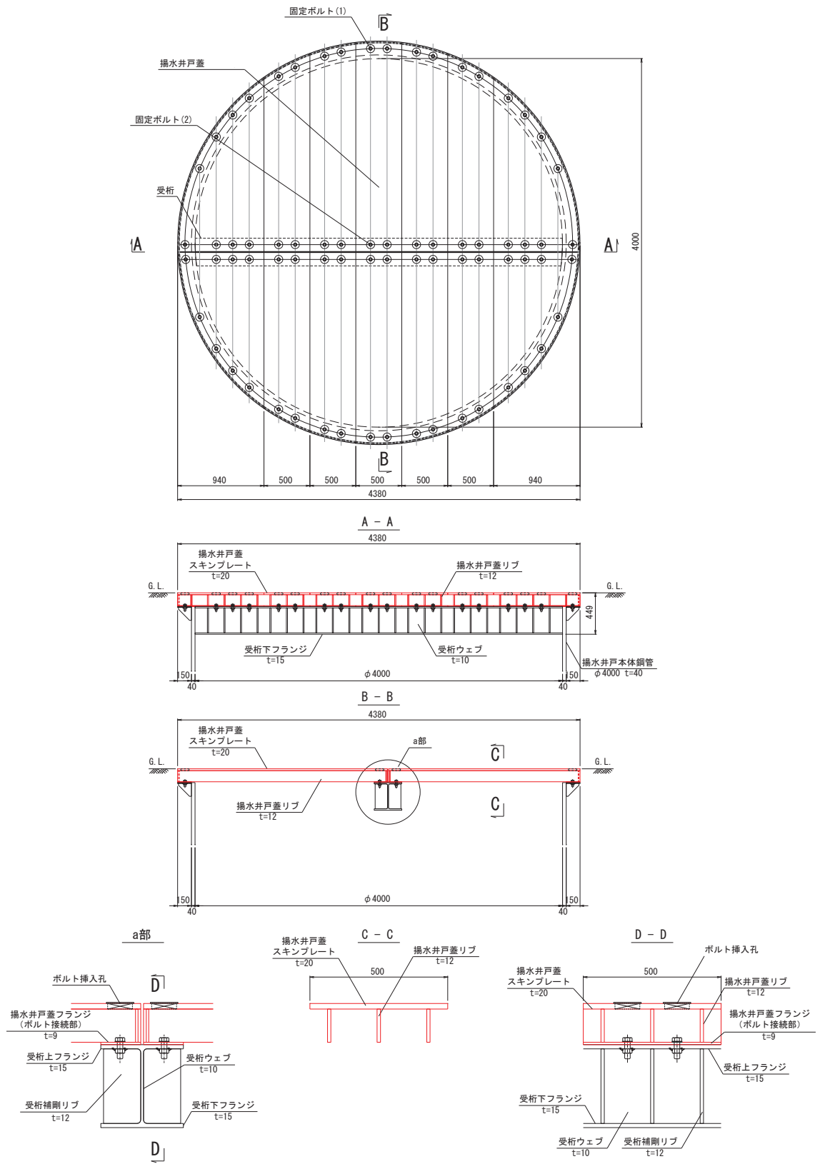
図 3-1(2) 評価対象部位 (No. 3, No. 4 揚水井戸蓋。朱書き部は蓋本体を示す。) (単位: mm)
