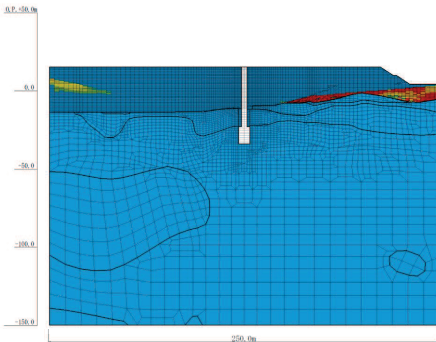
図 4-35(11) 最大過剰間隙水圧比分布 (No.4 揚水井戸, S s -D1 (++) , 解析ケース③)
