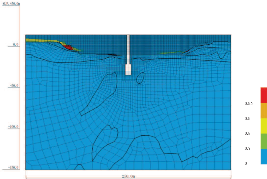
図 4-35(4) 最大過剰間隙水圧比分布 (No.2 揚水井戸, S_s - F 1 (一+), 解析ケース②)
