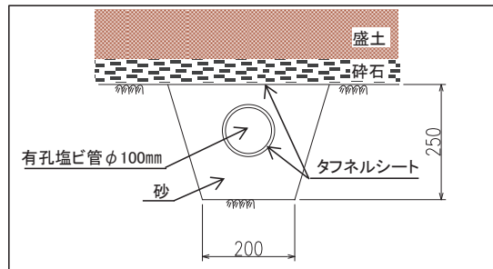
図 1-1-4 ドレーン (塩ビ管) 概要 (建屋間の施工例) (単位: mm)
