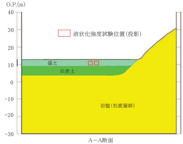
A-A断面
