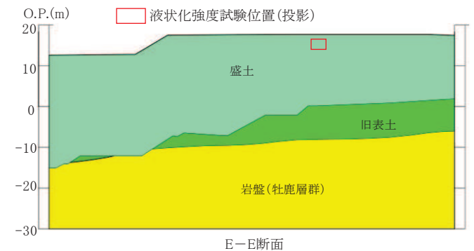
E-E断面
