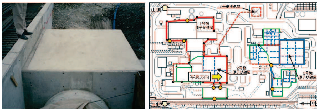
図 1-1-8 原子炉建屋周囲の接続柵の設置状況
