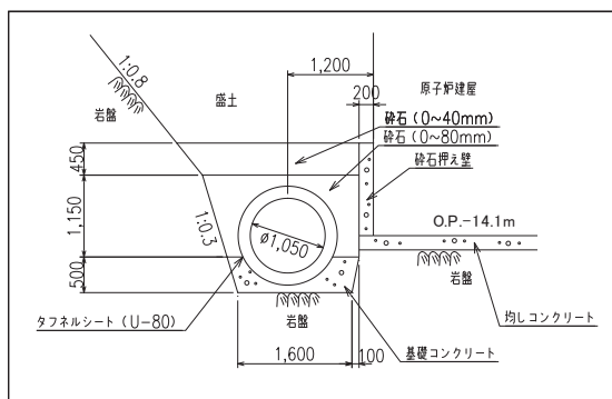
図 1-1-2 建屋外周のヒューム管概要 (単位：mm) (φ 1050 mm ヒューム管の例)
