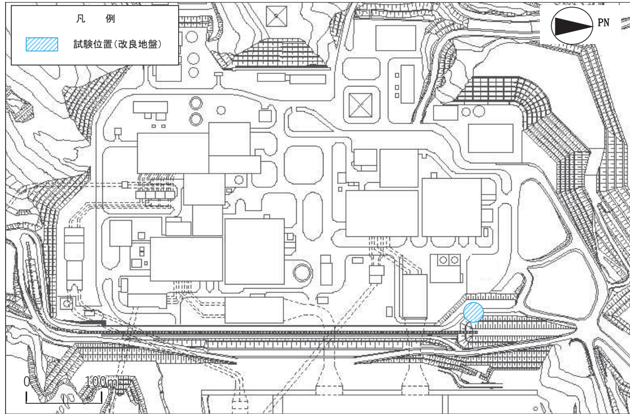
図 5.1-3 支持力試験実施位置(改良地盤)
