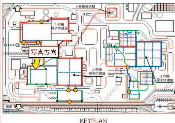
図 1-1-3 (2) 建屋等の直下のヒューム管設置状況 (タービン建屋直下の φ 500 ヒューム管の例)
