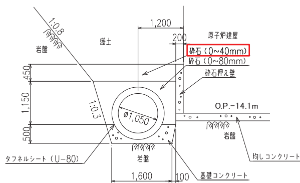
図 4-8 ヒューム管周辺のフィルター材設置状況（単位：mm）
