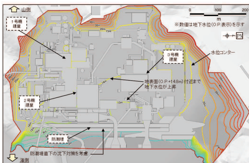
図 3-2 地下水位低下設備が機能しない場合の地下水位分布算定結果* 1
