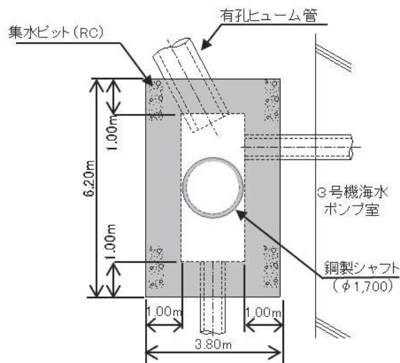
【揚水井戸⑧】平面図
