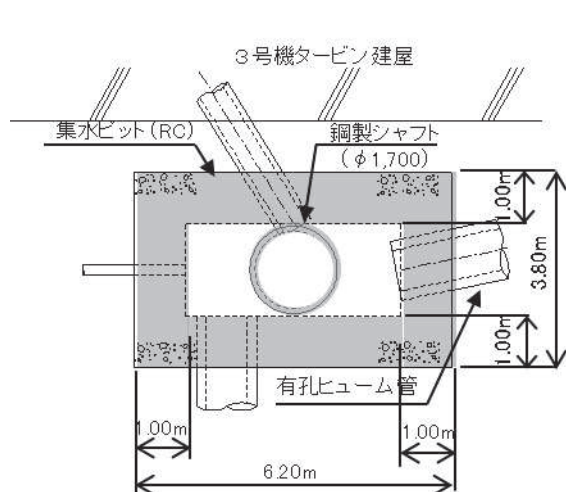
【揚水井戸⑦】平面図
