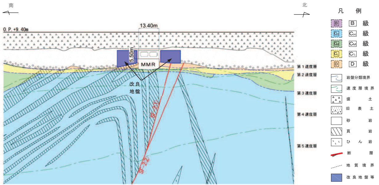
図 3.1-17(2) 取水路の地質断面図 (㉔-㉔断面)
