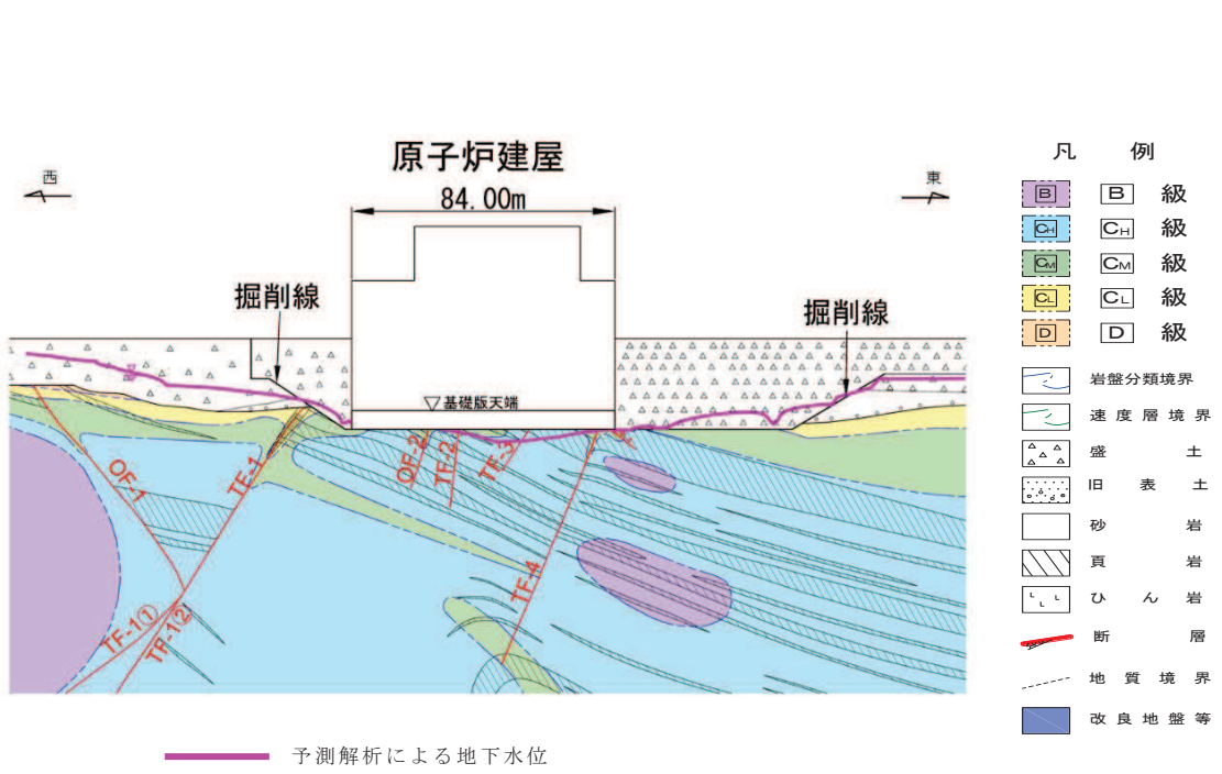
図 3.3-38 原子炉建屋周辺の地下水位分布(東西)
