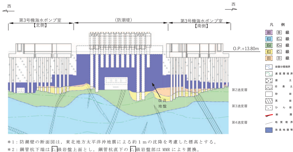
図 3.1-21(3) 防潮壁（第3号機海水ポンプ室）の地質断面図（②⑦-②⑦断面）
