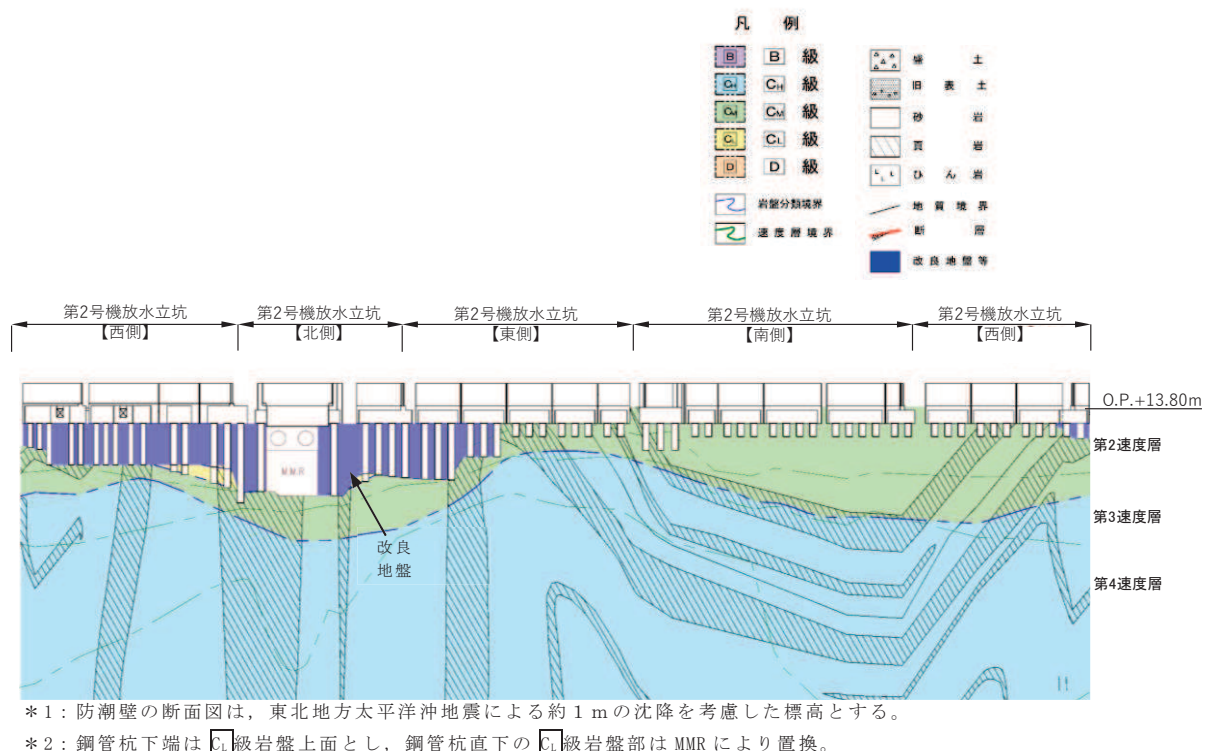
図 3.1-21(2) 防潮壁（第2号機放水立坑）の地質断面図（②⑥-②⑥断面）
