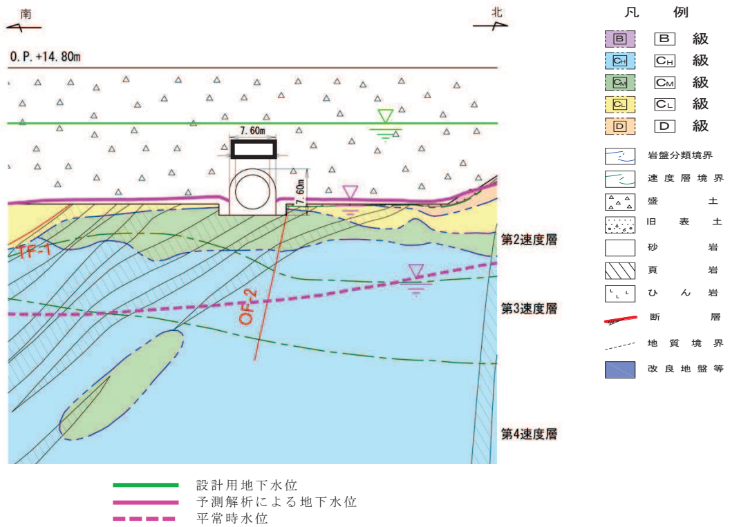
図 3.3-70 (2) 排気筒連絡ダクトにおける 設計用地下水位と平常時水位の比較 (横断(断面①))
