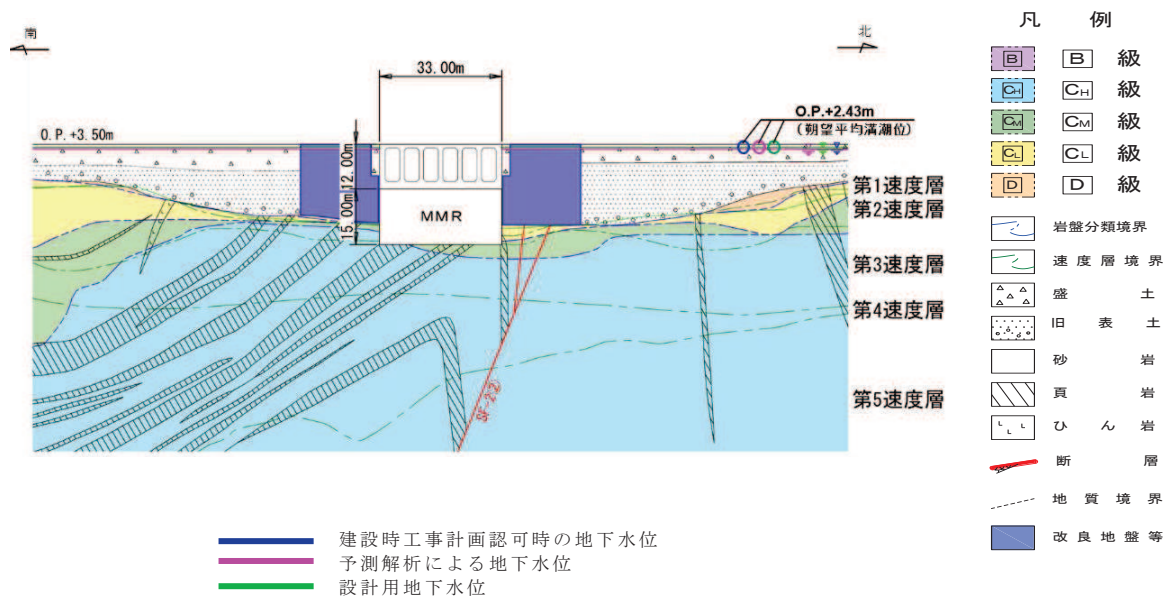
図 3.3-50(1) 取水口 (標準部) の設計用地下水位 (南北)
