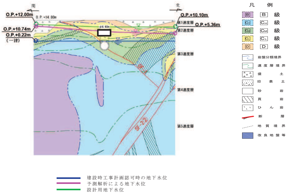
図 3.3-44(6) 排気筒連絡ダクトの設計用地下水位（横断(断面⑦)）
