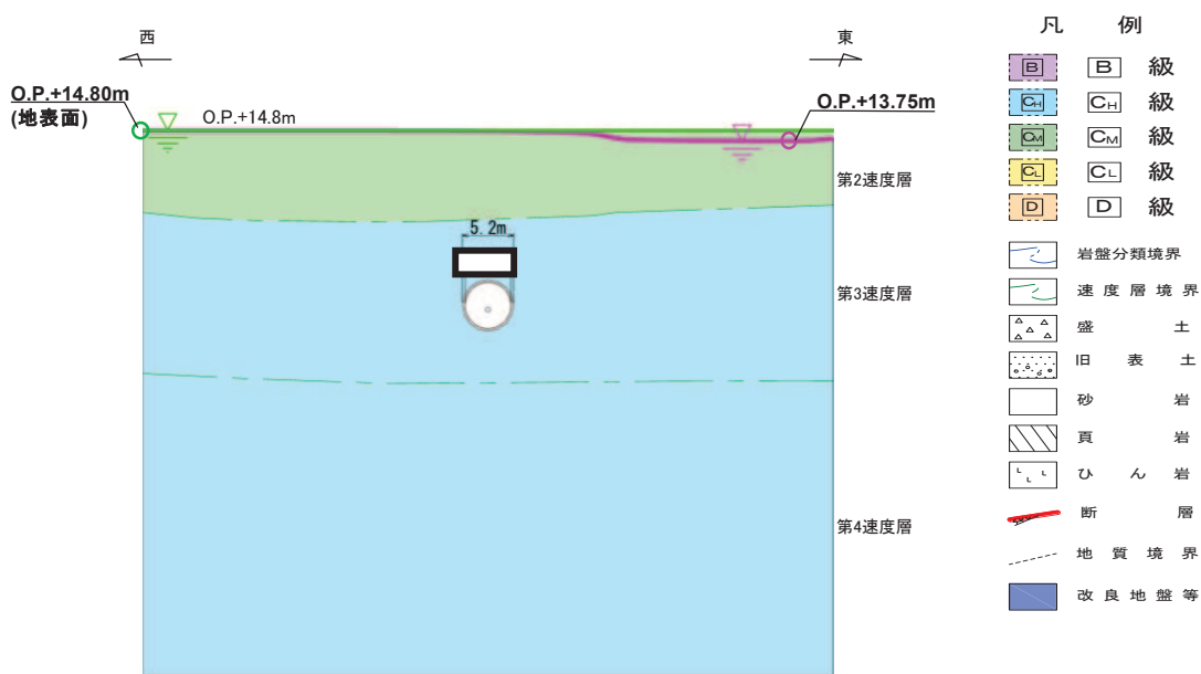
図 3.3-54(1) 取放水路流路縮小工の設計用地下水位 (1号機取水路)
