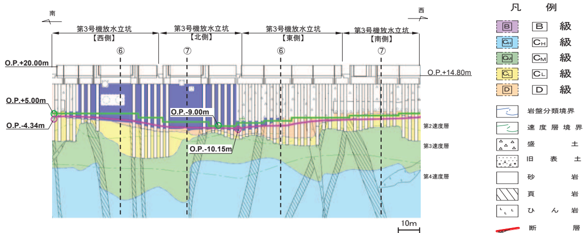
図 3.3-53(8) 防潮壁の設計用地下水位 (3号機海水ポンプ室) (3号機海水ポンプ室横断方向の地下水位分布 (南北) ⑤-⑤) (2/2)
