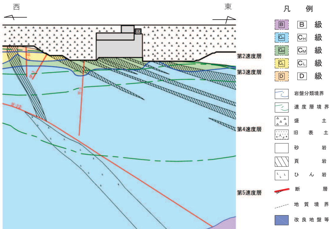
図 3.1-15 軽油タンク連絡ダクトの地質断面図 (⑰-⑰断面)
