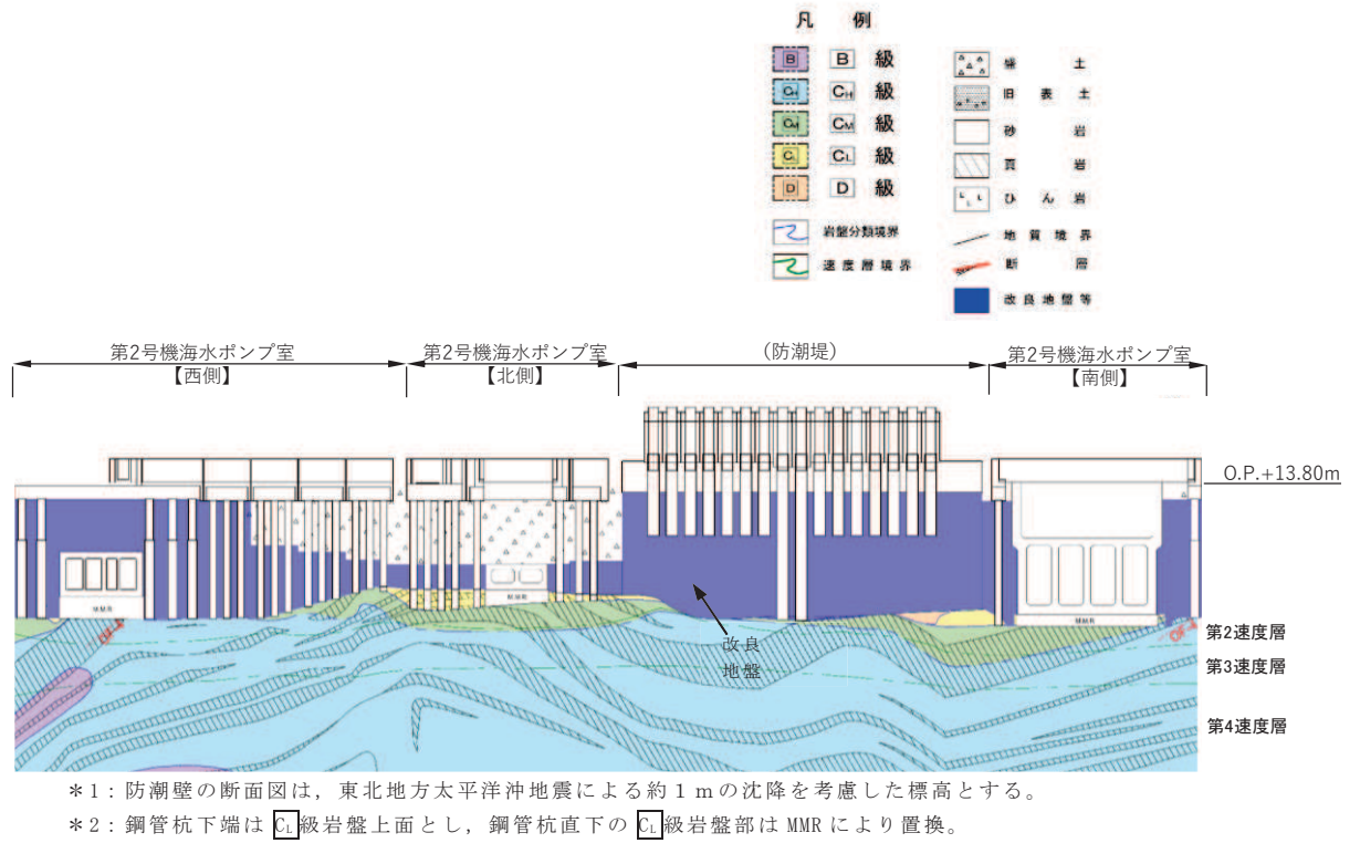
図 3.1-20 防潮堤（盛土堤防）の地質断面図（㉔-㉔断面）
