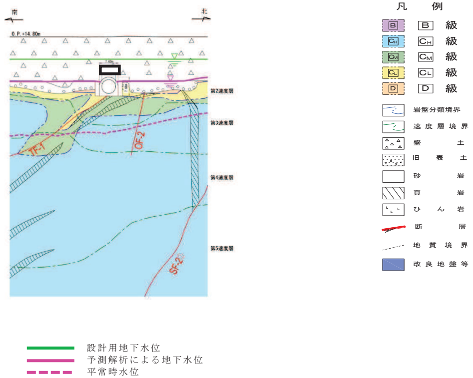
図 3.3-70 (3) 排気筒連絡ダクトにおける 設計用地下水位と平常時水位の比較 (横断(断面②))
