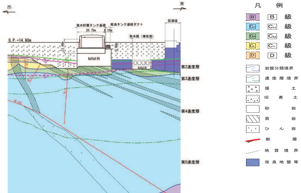
図 3.3-70 (6) 排気筒連絡ダクトにおける 設計用地下水位と平常時水位の比較 (横断(断面⑦))
