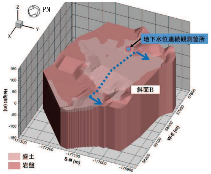
解析モデル
