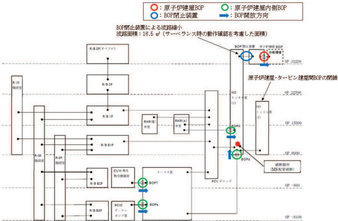
図 2-1 解析モデル
