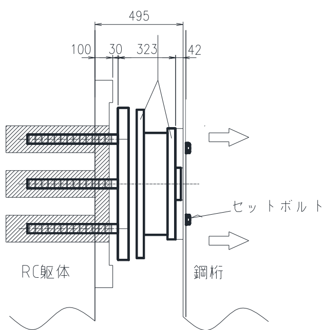
図 2(4) 水平支承の施工ステップ図
