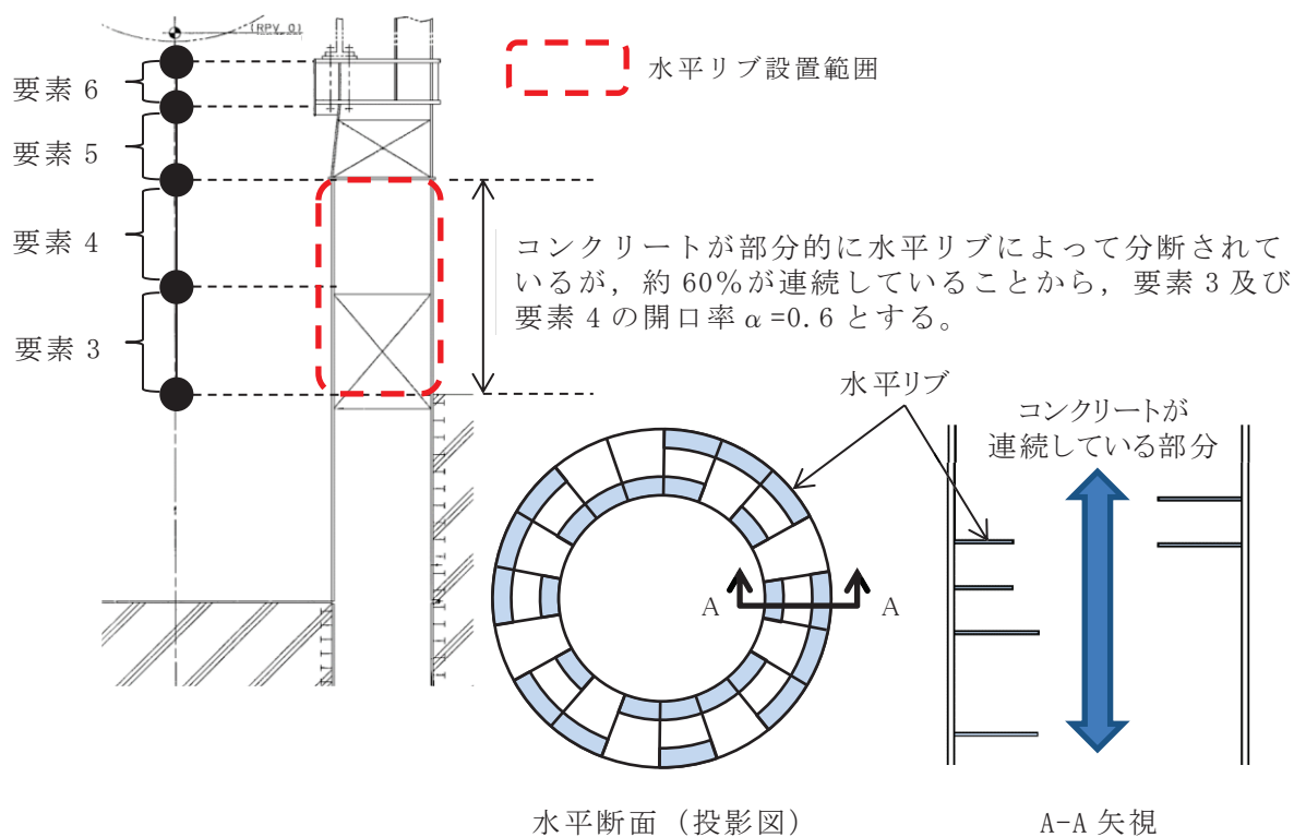
図4-4 水平リブがある場合の開口率の考え方
