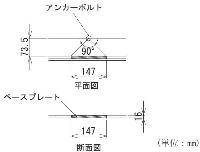
図 6.3-13 ベースプレートの断面照査諸元
