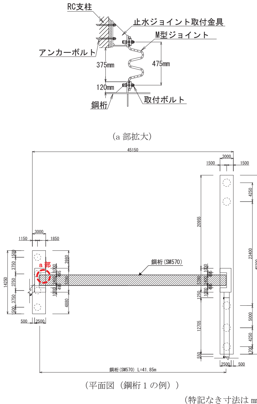
図 1-1 ブラケットの構造図 (RC 支柱と鋼桁間 (鋼桁 1, 4))
