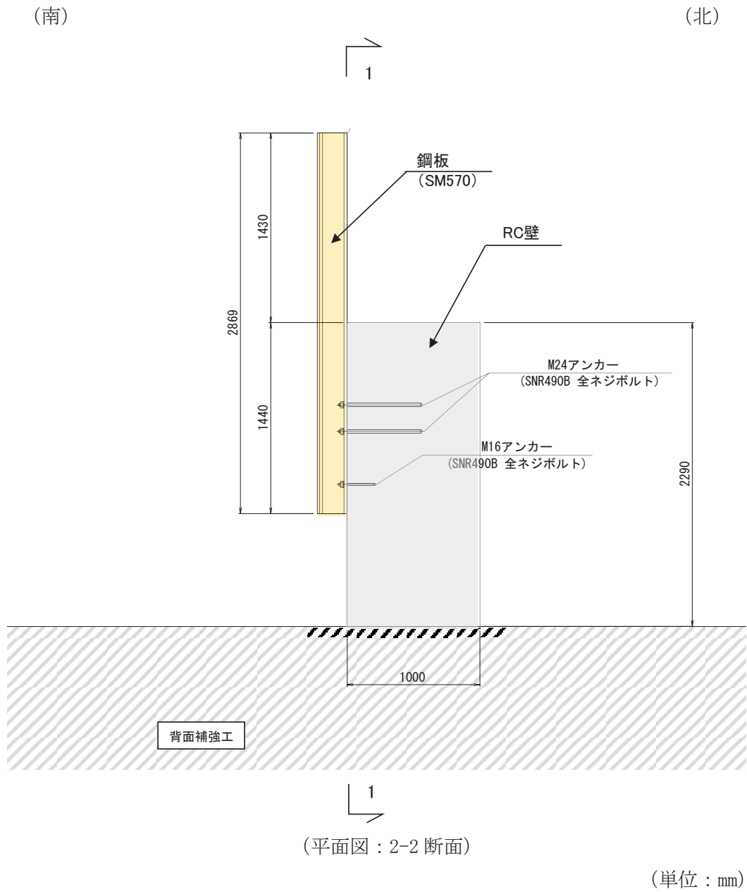
図 1-4(2) 防潮堤取り合い部の構造概要図 (防潮堤取り合い部②)
