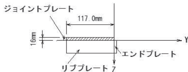
(D-D 断面)
