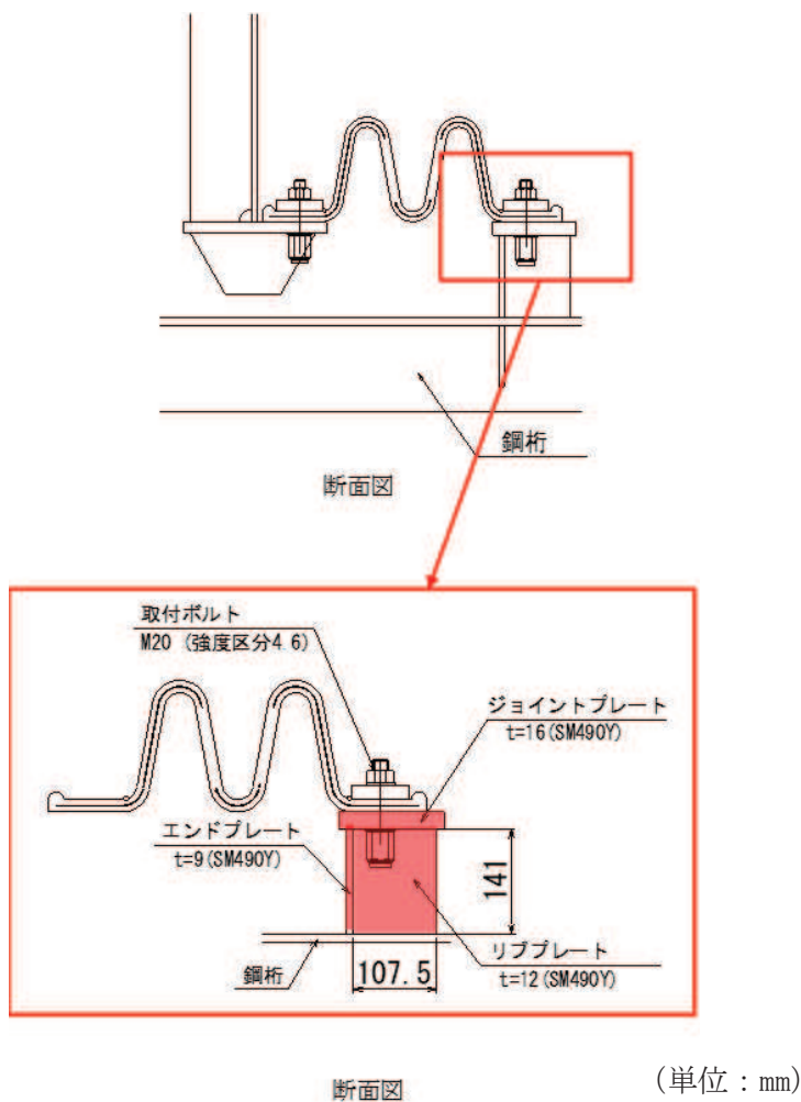
図 6.6-1 鋼桁端部ブラケットの構造概要
