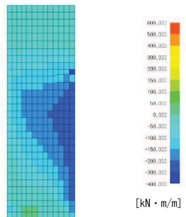
図 7.2-11(3) 曲げモーメント M_y 図
