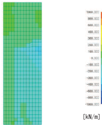
図 7.2-10(6) せん断力 Q_x 図
