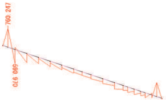
せん断力 Sy 図 角型鋼管 (kN)
