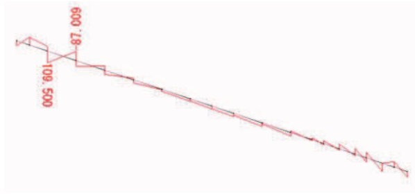
曲げモーメント Mz 図 角型鋼管 (kN・m)
