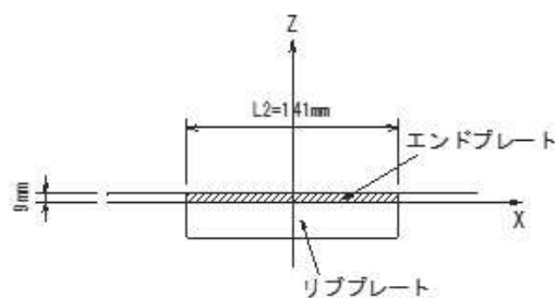
(F-F 断面)
