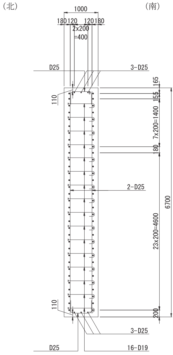
(正面図)
