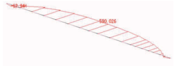
曲げモーメント My 図 角型鋼管 (kN・m)
