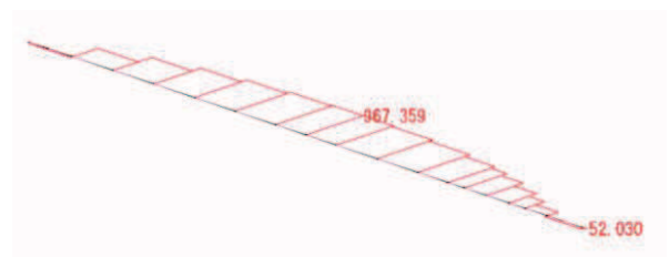
曲げモーメント My 図 角型鋼管 (負の周面摩擦力)
