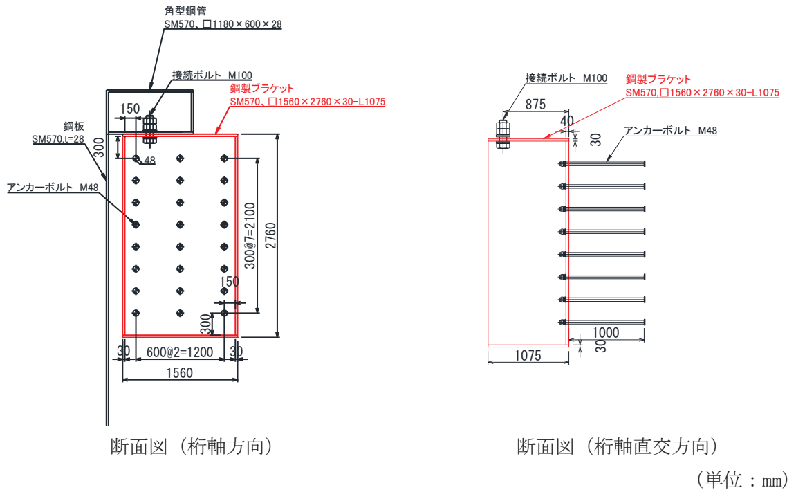
図 6.3-1(1) 鋼製ブラケットの構造概要（鋼桁 5）
