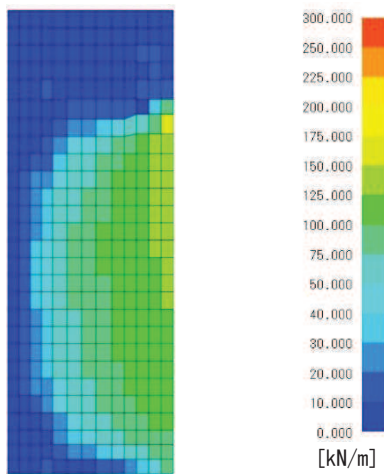
図 7.2-3 (8) 面内せん断力 N_{xy} 図
