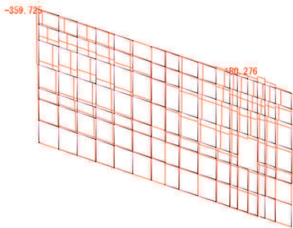
せん断力 S_x 図(縦方向はり要素) 鋼板 (kN)
