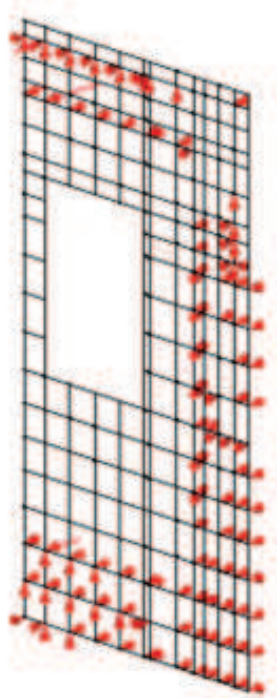
図 6.2-3(2) 反力図 (重疊時 (地下トレンチ② 右側))
