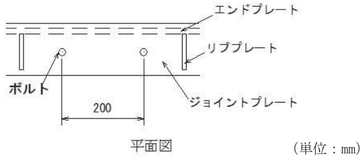
図 6.6-8 取り付けボルトの配置図
