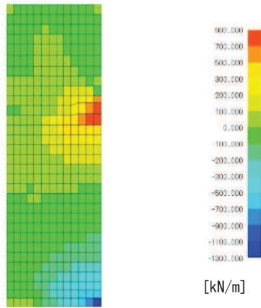
図 7.2-12(4) 軸力 N_x 図
