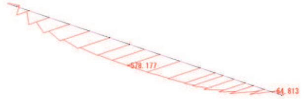
曲げモーメント My 図 角型鋼管 (kN・m)
