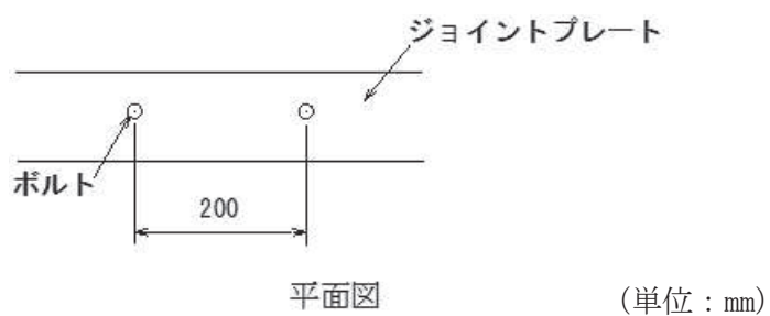
図 6.8-5 取り付けボルトの配置図
