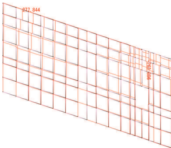
せん断力 S_x 図 (縦方向はり要素) 鋼板 (kN) せん断力 S_y 図 (横方向はり要素) 鋼板 (kN)
