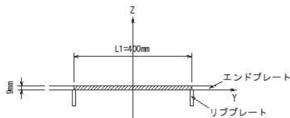
(E-E 断面)
