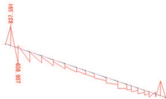
曲げモーメント Mz 図 角型鋼管 (負の周面摩擦力)
