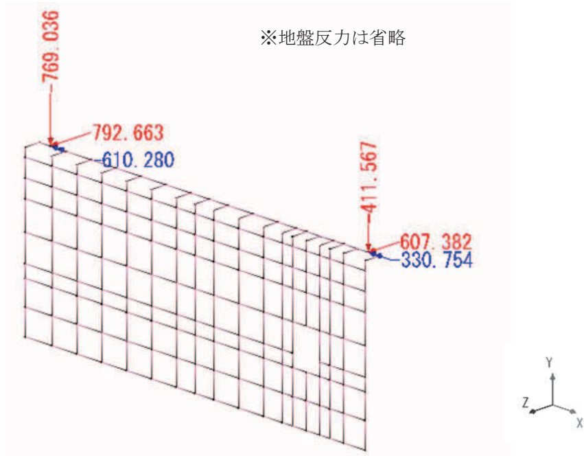
図 7.2-2(3) 反力図 (地震時①：外→内方向) (赤字：反力(kN)、青字：回転反力(kN・m))
