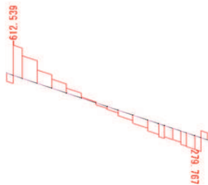
せん断力 Sy 図 角型鋼管 (kN)
