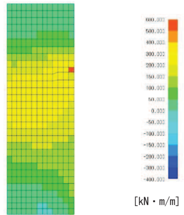
図 7.2-9(3) 曲げモーメント M_y 図
