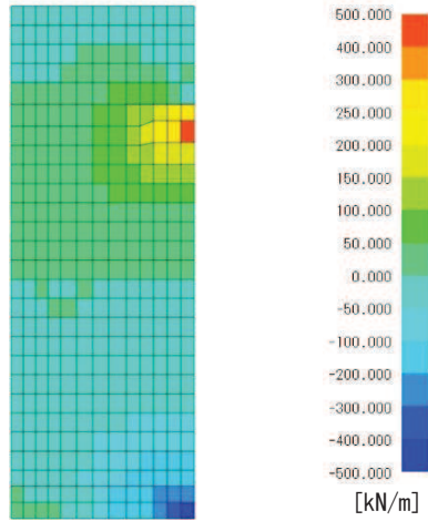
図 7.2-2 (4) 軸力 N_x 図
