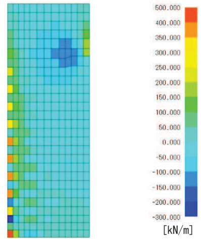
図 7.2-3 (7) せん断力 Q_y 図
