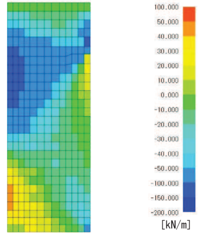
図 7.2-2 (5) 軸力 N_y 図
