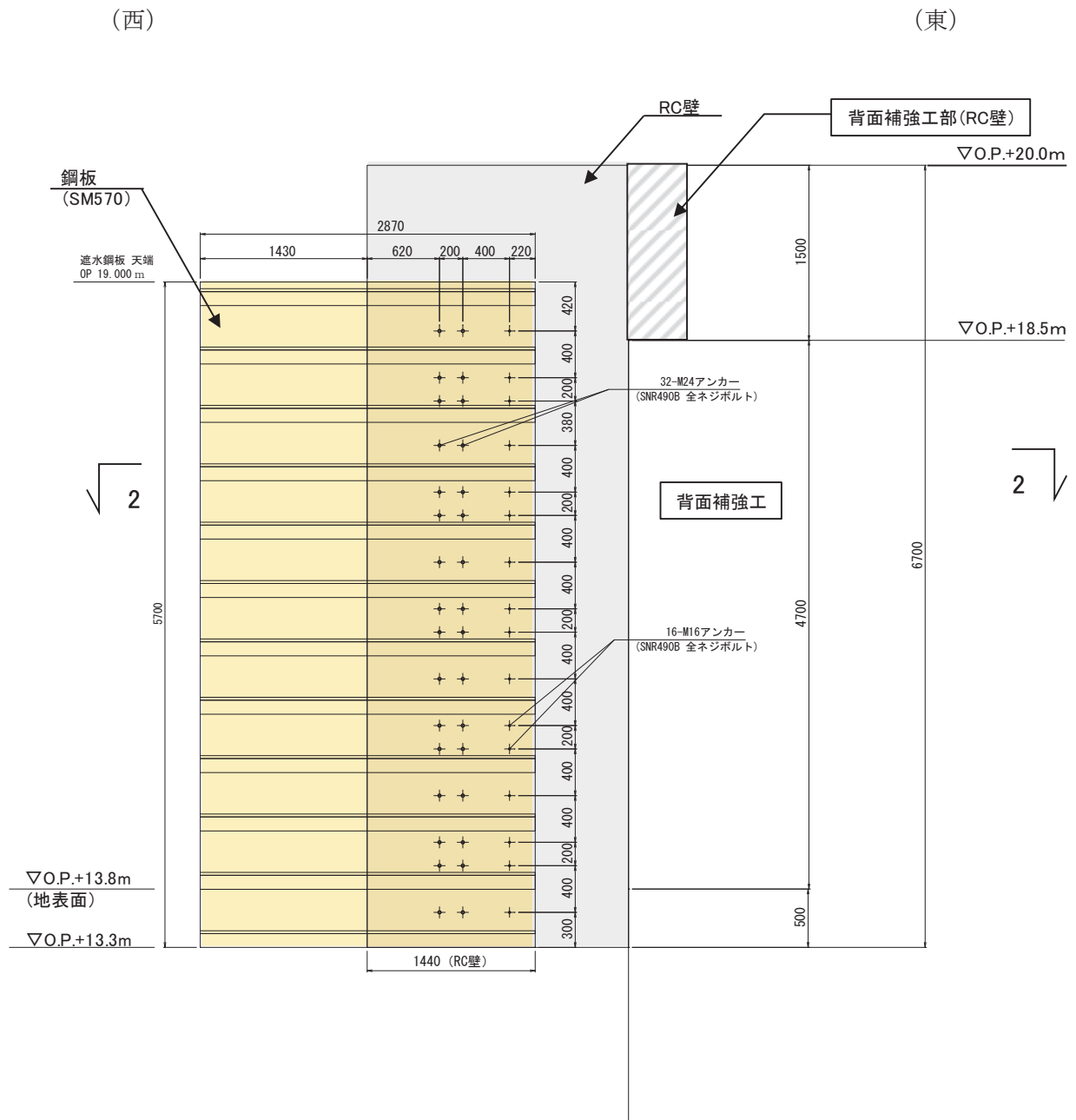
(正面図：1-1 断面)
