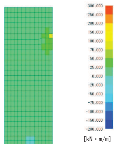
図 7.2-2 (3) 曲げモーメント M_y 図
