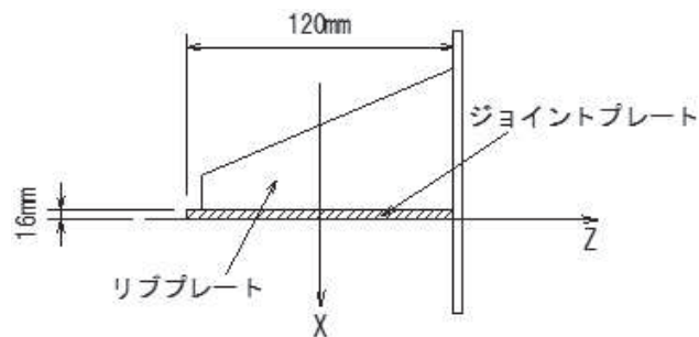
(C-C 断面)
