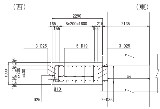
(平面図)
