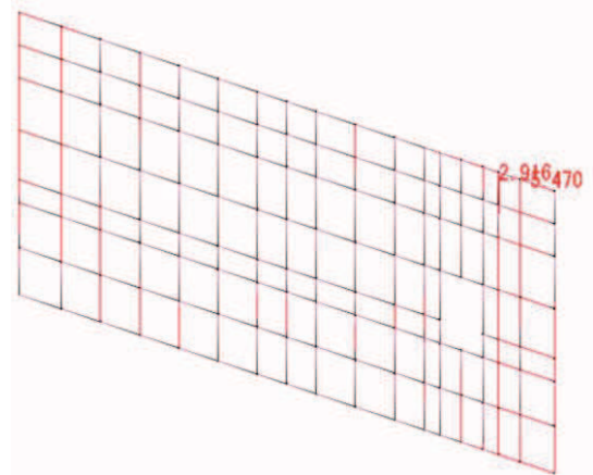
曲げモーメント M_x 図 (縦方向はり要素) 鋼板 曲げモーメント M_y 図 (横方向はり要素) 鋼板 (負の周面摩擦力)
