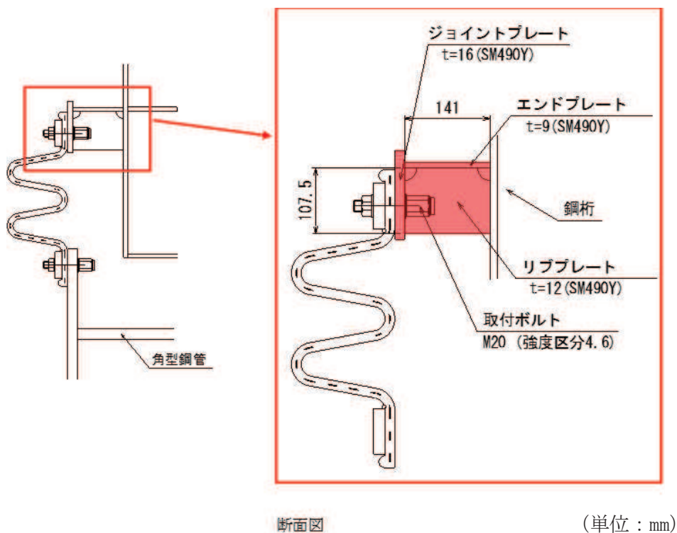
図 6.5-1 鋼桁支間部ブラケットの構造概要
