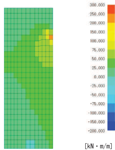
図 7.2-1(3) 曲げモーメント M_y 図
