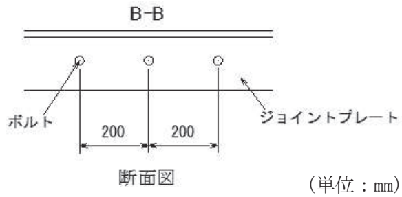
図 6.1-6 取り付けボルトの配置図
