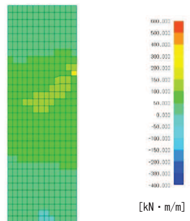
図 7.2-10(3) 曲げモーメント M_y 図
