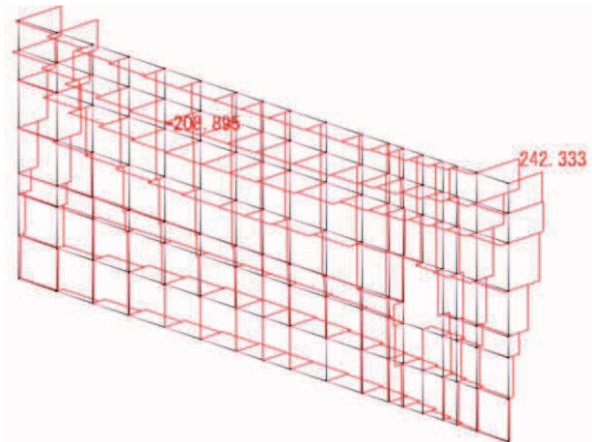
軸力 N_x 図(横方向はり要素) 鋼板(kN) 軸力 N_y 図(縦方向はり要素) 鋼板(kN)
