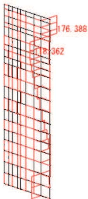
せん断力 S_z 図 (kN)
