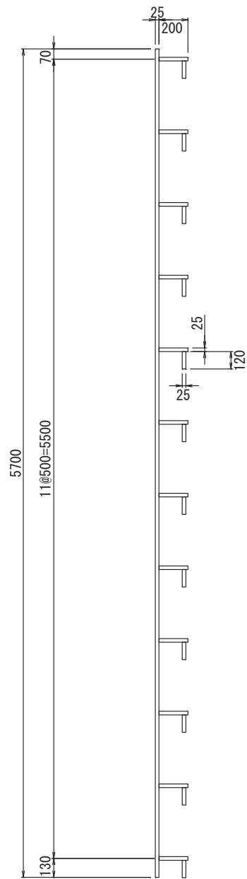
(鋼板断面図)
