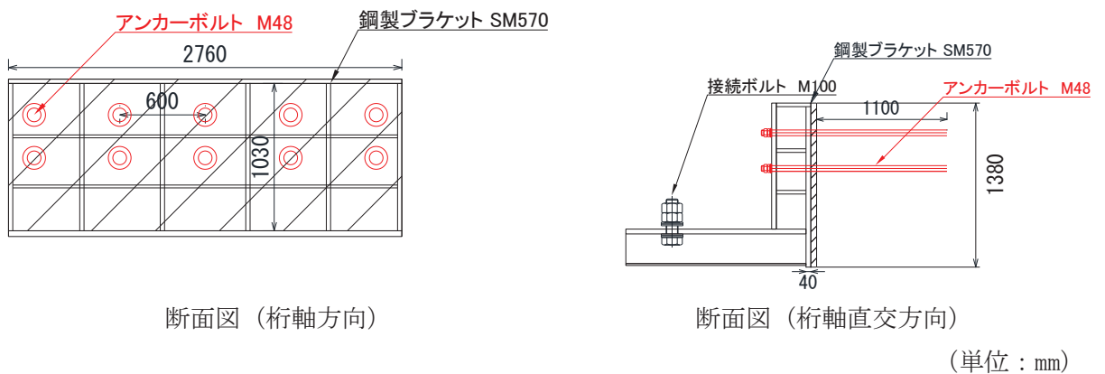
図 6.4-1(2) アンカーボルトの構造概要(防潮堤取り合い部④ 防潮堤側)
