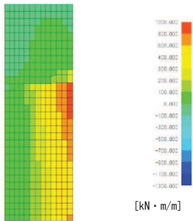
図 7.2-9(2) 曲げモーメント M_x 図
