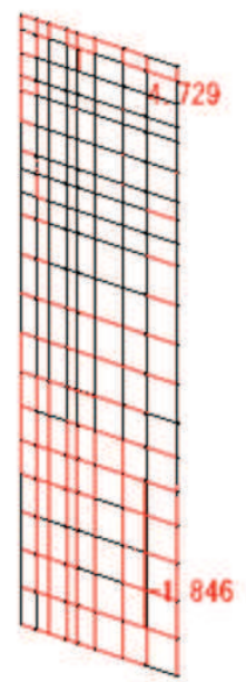
軸力 N_y 図 (縦方向はり要素) (kN)
