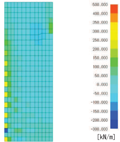
図 7.2-4 (7) せん断力 Q_y 図
