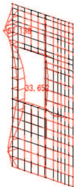
曲げモーメント M_x 図(縦方向はり要素) (kN・m) 曲げモーメント M_y 図(横方向はり要素) (kN・m)
