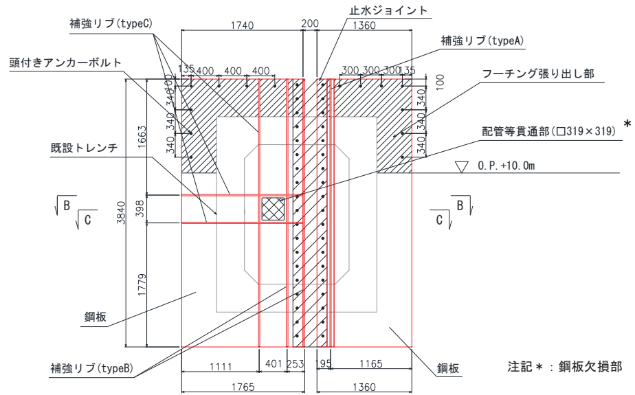
B - B 平面図
