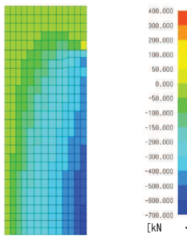
図 7.2-3 (2) 曲げモーメント M_x 図
