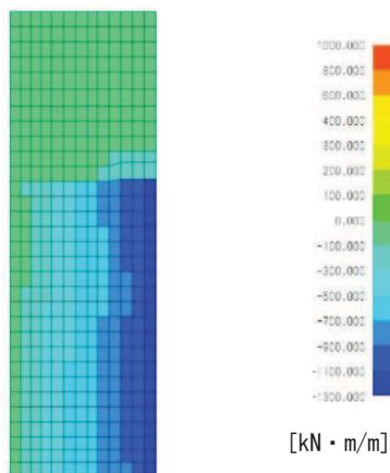
図 7.2-11(2) 曲げモーメント M_x 図
