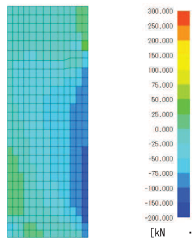
図 7.2-3 (3) 曲げモーメント M_y 図
