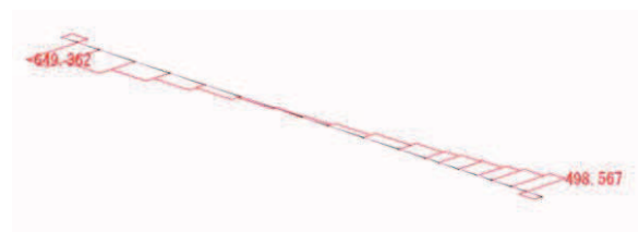
せん断力 Sz 図 角型鋼管 (kN)
