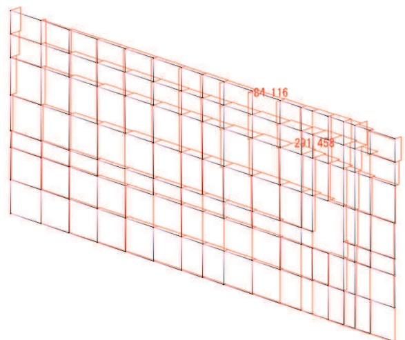
軸力 Nx 図(横方向はり要素) 鋼板(kN)
