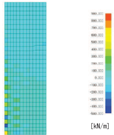
図 7.2-12(7) せん断力 Q_y 図
