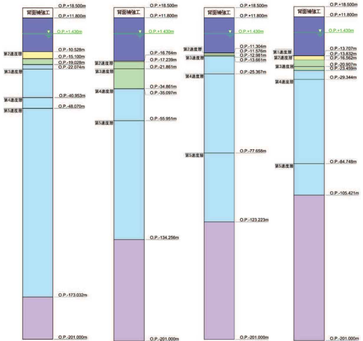
(防潮堤取り合い部④) (防潮堤取り合い部③) (防潮堤取り合い部②) (防潮堤取り合い部①)
