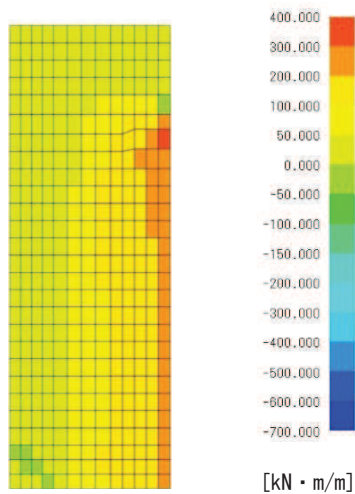
図 7.2-1(2) 曲げモーメント M_x 図
