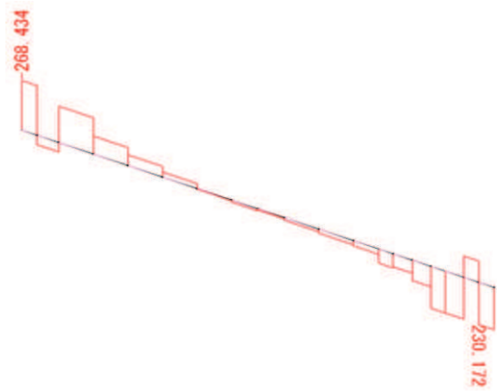
せん断力 S_y 図 角型鋼管
