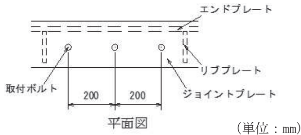
図 6.3-7 取り付けボルトの配置図
