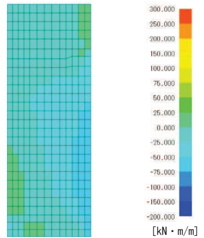
図 7.2-4 (3) 曲げモーメント M_y 図
