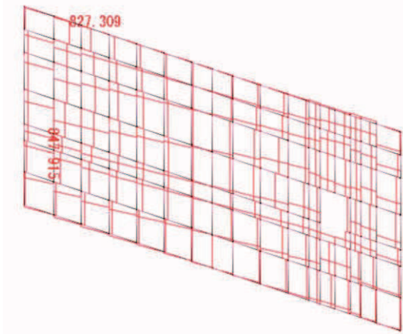
せん断力 S_x 図(縦方向はり要素) 鋼板 せん断力 S_y 図(横方向はり要素) 鋼板 (負の周面摩擦力)
