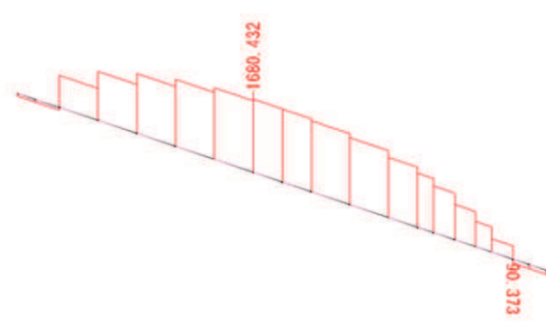
軸力 N_x 図 角型鋼管 (kN) (負の周面摩擦力)
