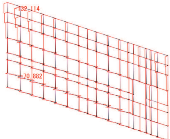
せん断力 S_z 図 鋼板
