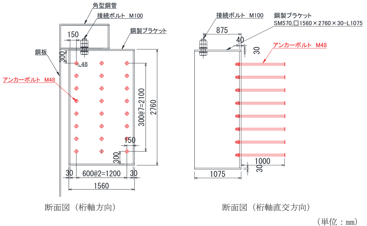
図 6.4-1(1) アンカーボルトの構造概要(鋼桁 5)
