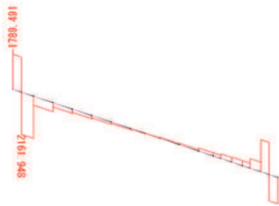
せん断力 Sy 図 角型鋼管 (負の周面摩擦力)
