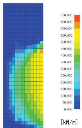
図 7.2-10(8) 面内せん断力 N_{xy} 図
