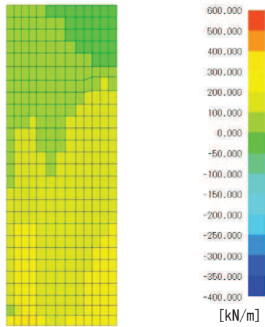
図 7.2-4 (6) せん断力 Q_x 図
