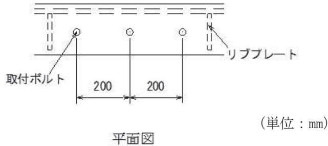
図 6.4-12 取り付けボルトの配置図
