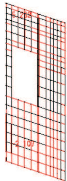
軸力 N_y 図(縦方向はり要素) (kN) 軸力 N_x 図(横方向はり要素) (kN)
