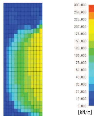
図 7.2-2 (6) 面内せん断力 N_{xy} 図
