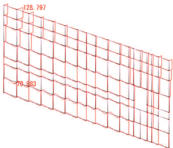
せん断力 S_z 図 鋼板
