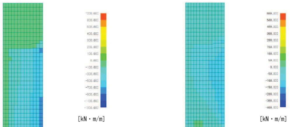
図 7.2-12(2) 曲げモーメント M_x 図
