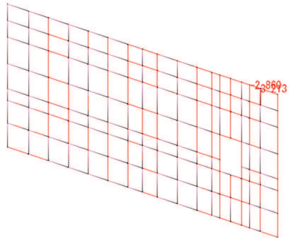
せん断力 S_z 図 鋼板 (負の周面摩擦力)
