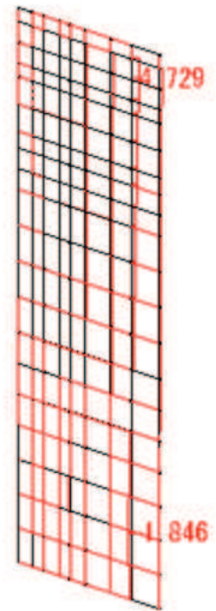
軸力 N_y 図(縦方向はり要素) (kN)
