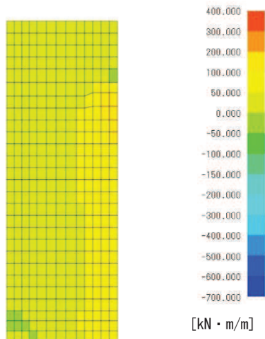
図 7.2-2 (2) 曲げモーメント M_x 図
