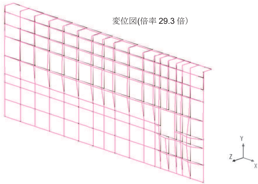
図 7.2-5(4) 変形図 (重畳時①)
