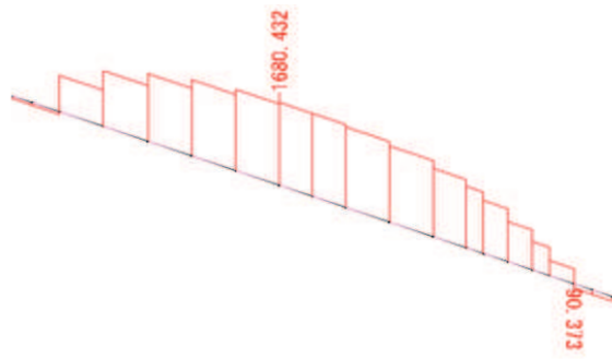
軸力 N_x 図 角型鋼管 (kN)
