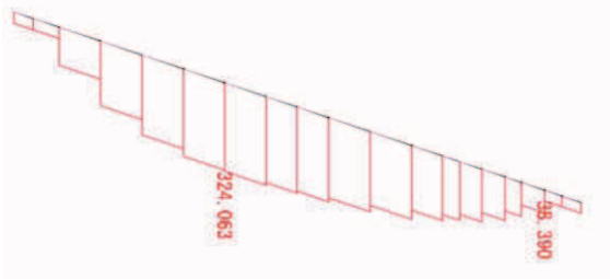
軸力 N_x 図 角型鋼管(kN)
