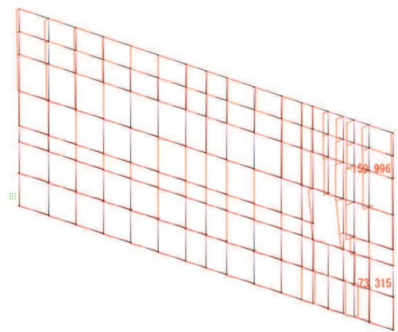
せん断力 S_z 図 鋼板 (kN)
