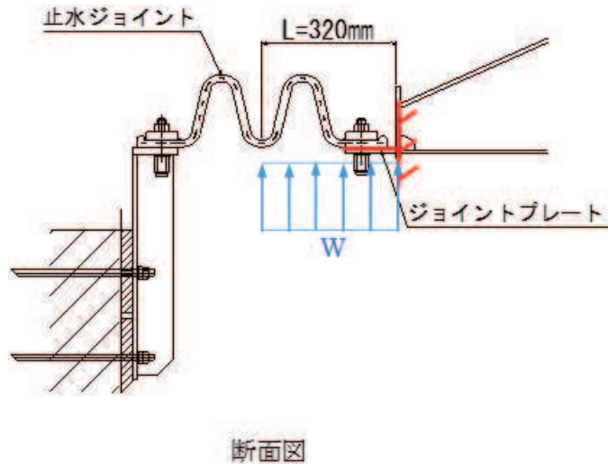
図 6.1-2 断面力の算定モデル
