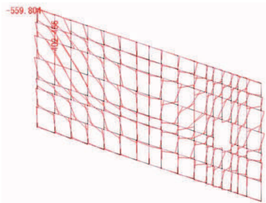
曲げモーメント M_z 図 鋼板 (負の周面摩擦力)
