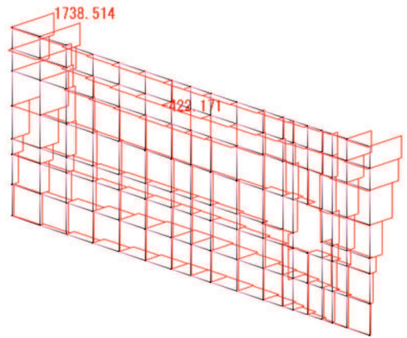
軸力 Nx 図 (横方向はり要素) 鋼板 (kN)
