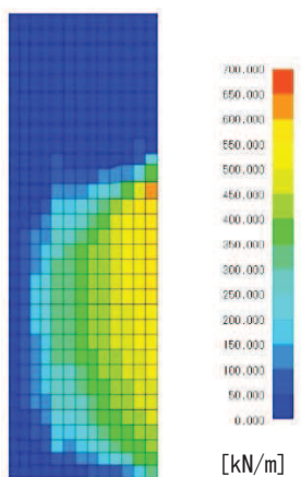
図 7.2-12(8) 面内せん断力 N_{xy} 図
