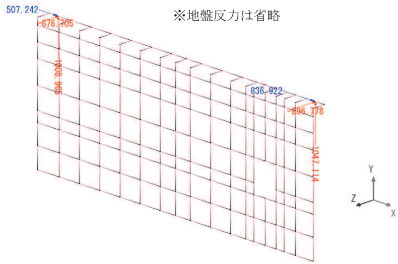
図 7.2-5(3) 反力図 (重畳時①) (赤字 : 反力 (kN)、青字 : 回転反力 (kN・m))
