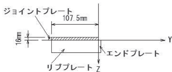
(C-C 断面)
