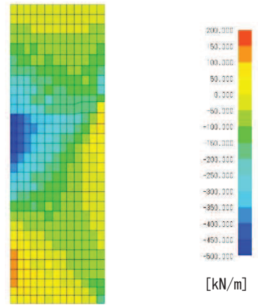
図 7.2-12(5) 軸力 N_y 図
