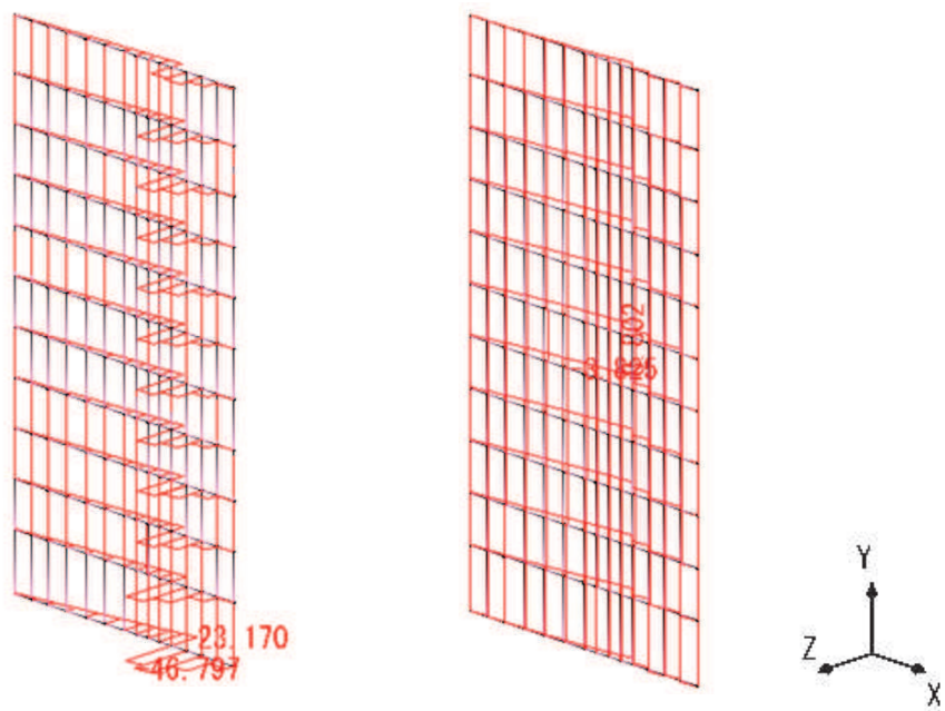
図 7.2-5(1) 断面力図 (地震時 1.0Ss 水平_0.4Ss 鉛直)
