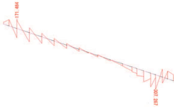
曲げモーメント Mz 図 角型鋼管 (kN・m)
