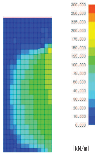
図 7.2-1 (8) 面内せん断力 N_{xy} 図
