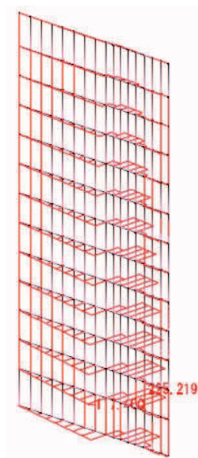
図 7.2-15(1) 断面力図 (重疊時 1.0Sd 水平_-0.4Sd 鉛直)
