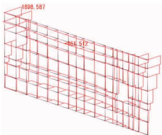
軸力 N_x 図 (横方向はり要素) 鋼板 (kN) 軸力 N_y 図 (縦方向はり要素) 鋼板 (kN) (負の周面摩擦力)
