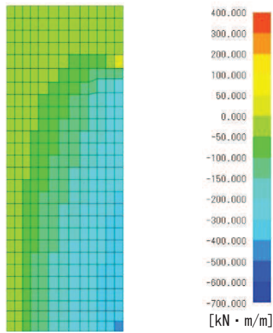
図 7.2-4 (2) 曲げモーメント M_x 図
