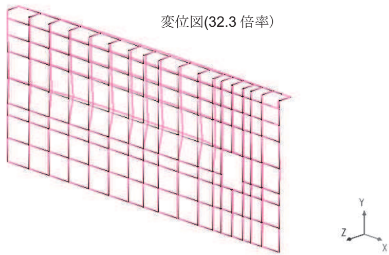
図 7.2-2(4) 変形図 (地震時①：外→内方向)
