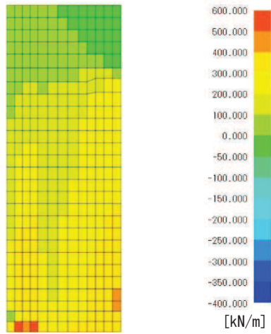
図 7.2-3 (6) せん断力 Q_x 図
