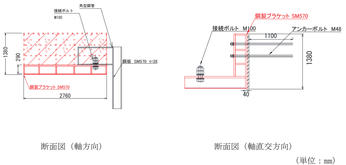
図 6.3-1(2) 鋼製ブラケットの構造図（防潮堤取り合い部④ 防潮堤側）
