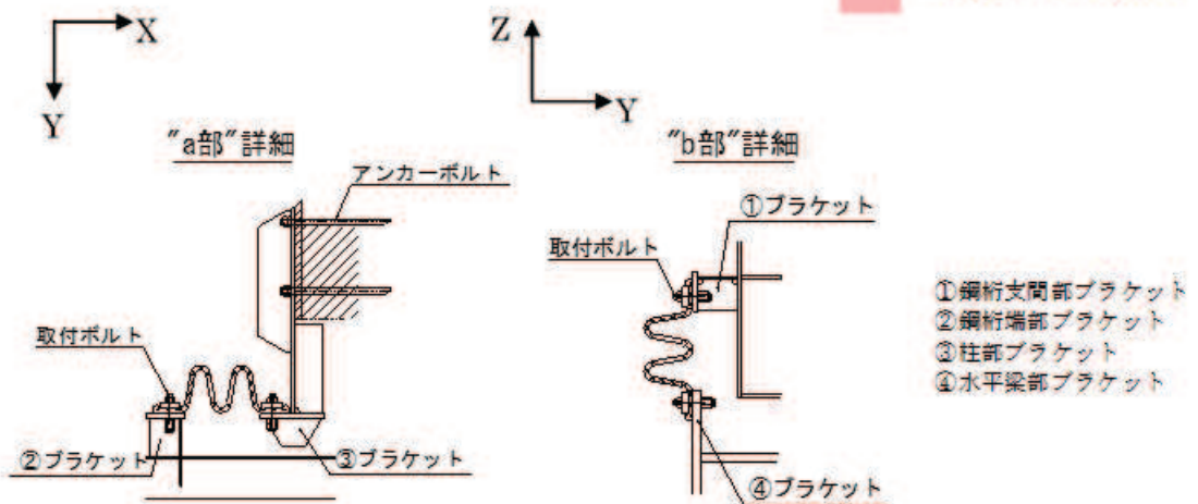
図 3-1(2) ブラケットの構造概要 (鋼桁 2・3・5・6)
