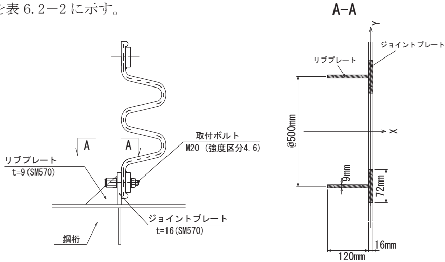
図 6.2-3 ジョイントプレートとリブプレートの断面照査諸元
