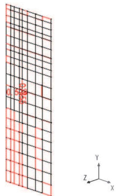
せん断力 S_x 図 (縦方向はり要素) (kN)
