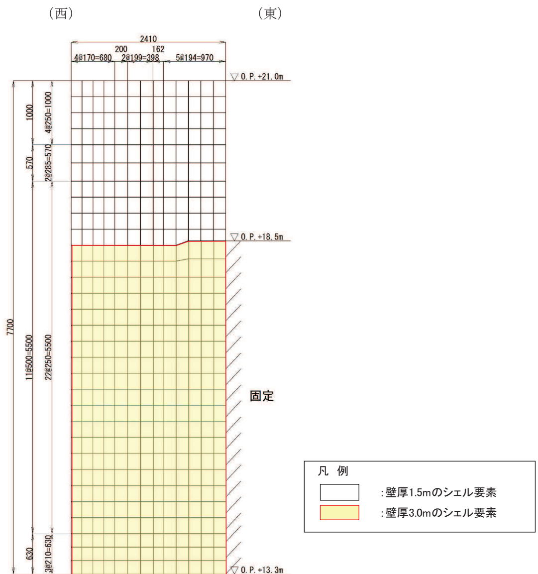
図 4.1-1 固有値解析モデル (RC 壁)
