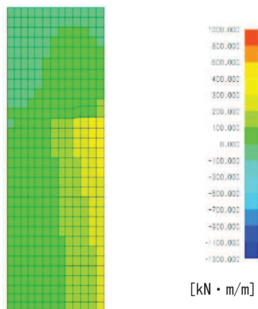
図 7.2-10(2) 曲げモーメント M_x
