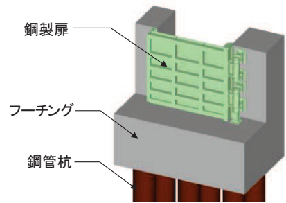
(鋼製扉)
