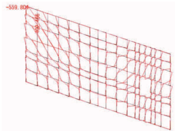
曲げモーメント M_z 図 鋼板 (負の周面摩擦力)
