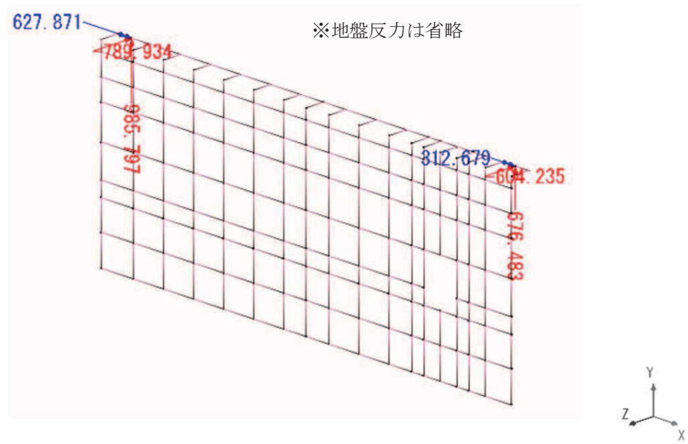
図 7.2-1(3) 反力図 (地震時①：内→外方向) (赤字：反力(kN)、青字：回転反力(kN・m))
