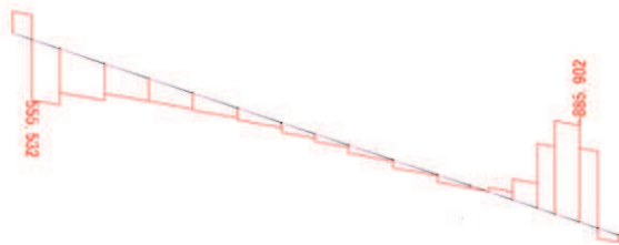
せん断力 S_y 図 角型鋼管
