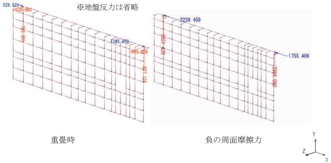
図 7.2-6(5) 反力図 (重畳時② (負の周面摩擦力の影響を考慮)) (赤字: 反力(kN)、青字: 回転反力(kN・m))
