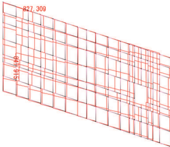
せん断力 S_x 図(縦方向はり要素) 鋼板 せん断力 S_y 図(横方向はり要素) 鋼板 (負の周面摩擦力)
