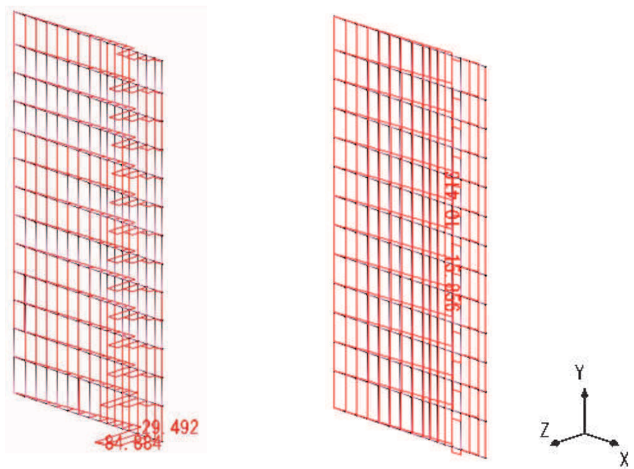
図7.2-13(1) 断面力図(地震時 1.0Ss 水平_-0.4Ss 鉛直)
