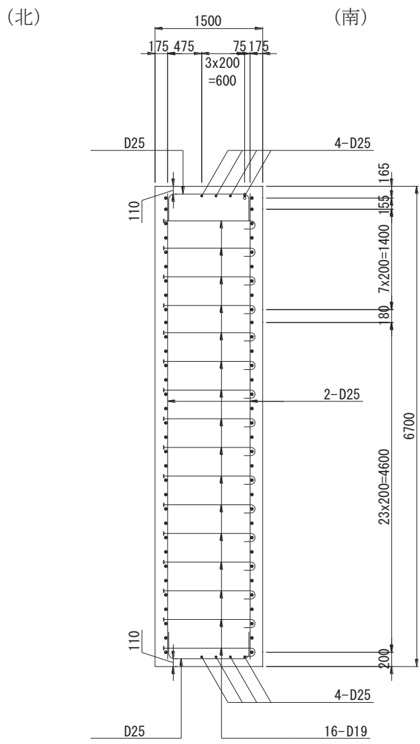
(正面図)
