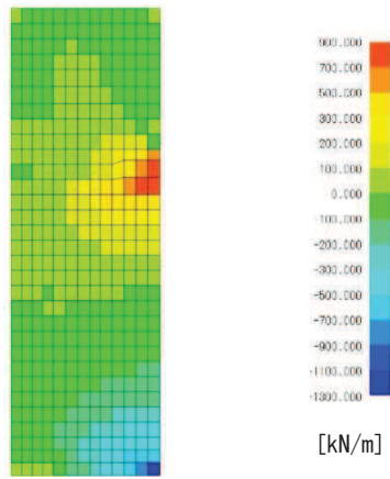
図 7.2-10(4) 軸力 N_x 図
