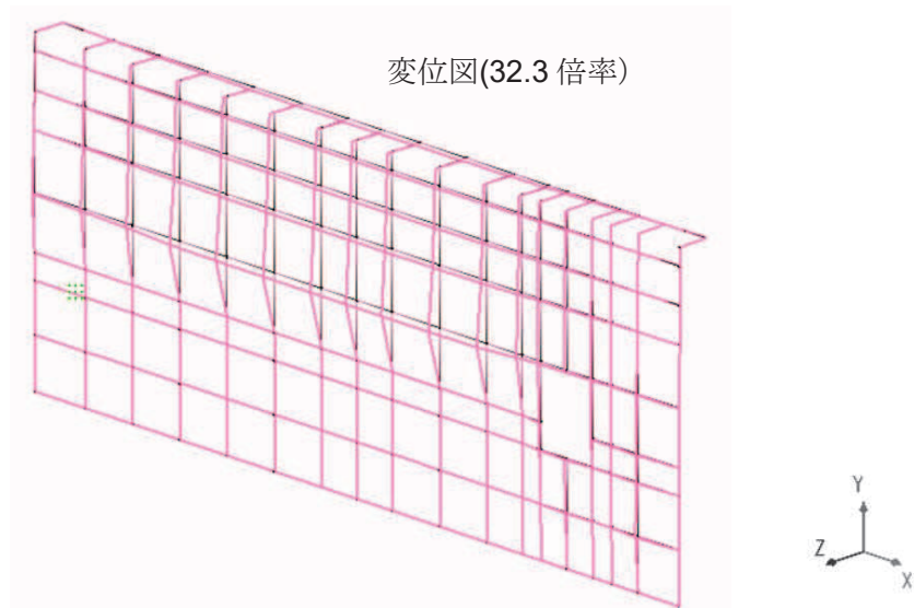
図 7.2-1(4) 変形図 (地震時①：内→外方向)
