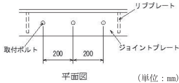
図 6.2-7 取り付けボルトの配置図
