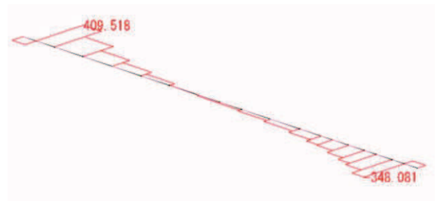
せん断力 S_z 図 角型鋼管
