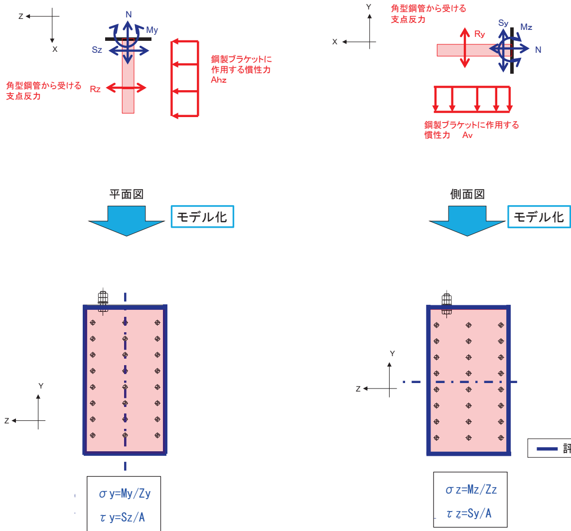
図 6.3-4 鋼製ブラケット 発生応力度算出概要図(鋼桁 5)
