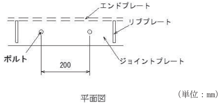
図 6.7-14 取り付けボルトの配置図
