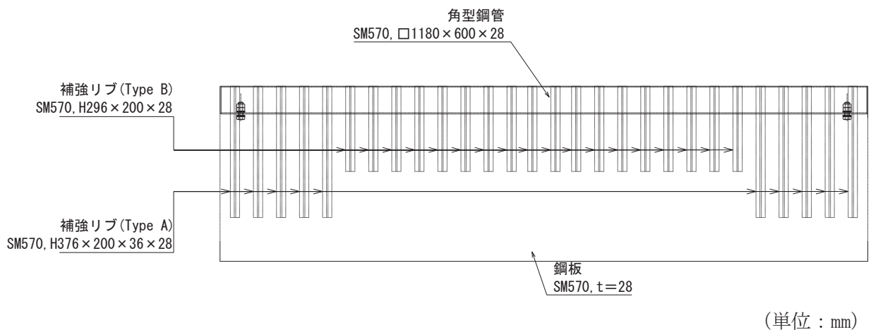
図 6.1-8 鋼板の構造図（正面図，断面図）
