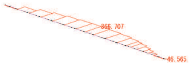
せん断力 Sz 図 角型鋼管 (kN)
