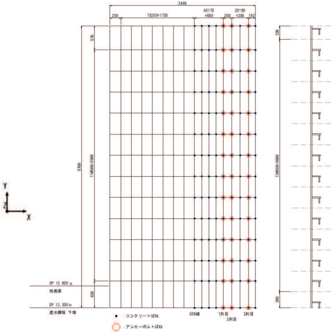
(平面図)
