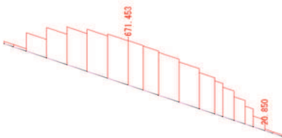
軸力 N_x 図 角型鋼管 (kN)
