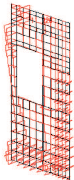
せん断力 S_z 図(kN)
