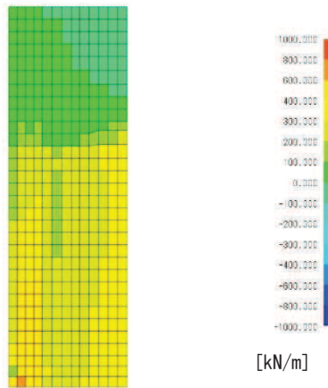
図 7.2-12(6) せん断力 Q_x 図
