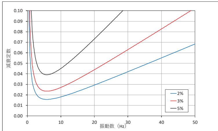
図 3.5-19 設定した Rayleigh 減衰 (断面⑧) _減衰 2%~5%
