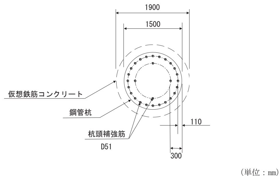
図 3.5-50 仮想鉄筋コンクリート断面概念図
