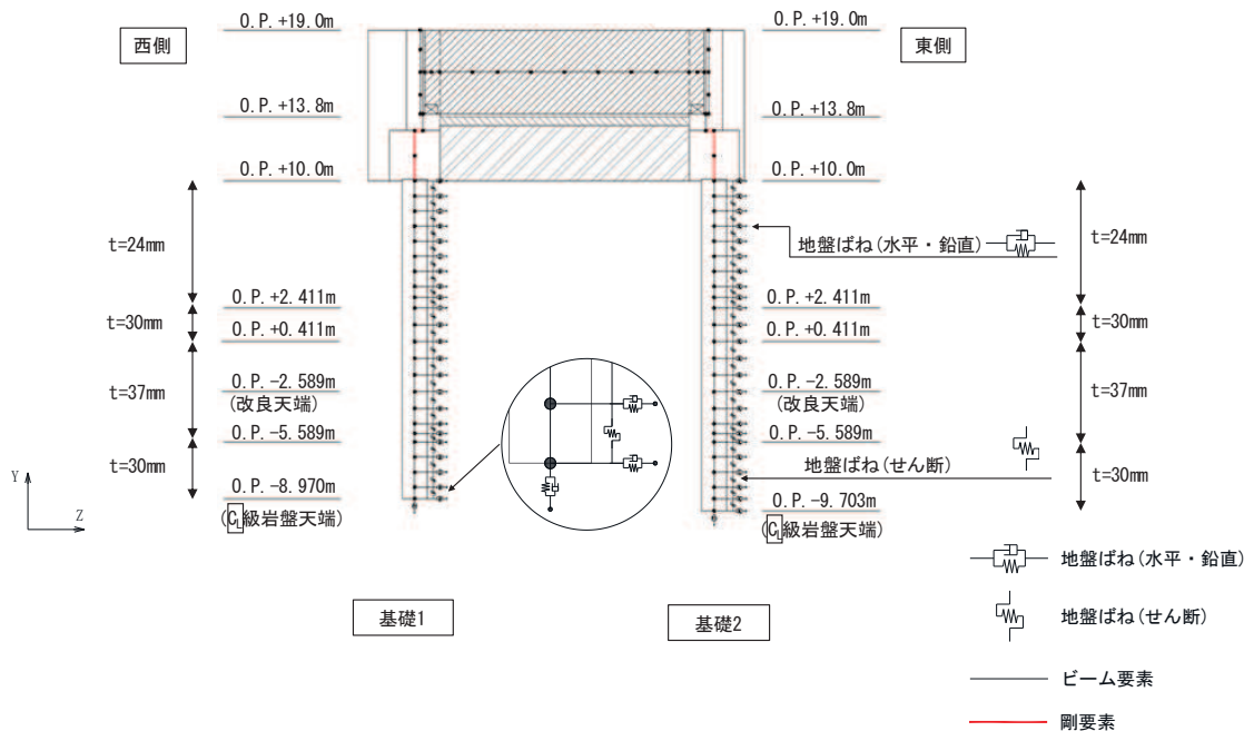
図 3.5-34 固有値解析モデル（鋼桁 2 の例）
