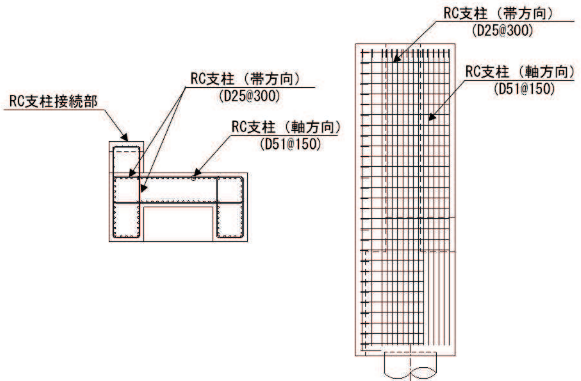
(平面図)
