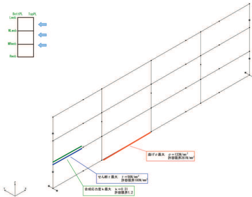
図 4.1-2 鋼桁の曲げ・軸力系の破壊及びせん断破壊に対する最大照査値発生箇所（鋼桁 2）
