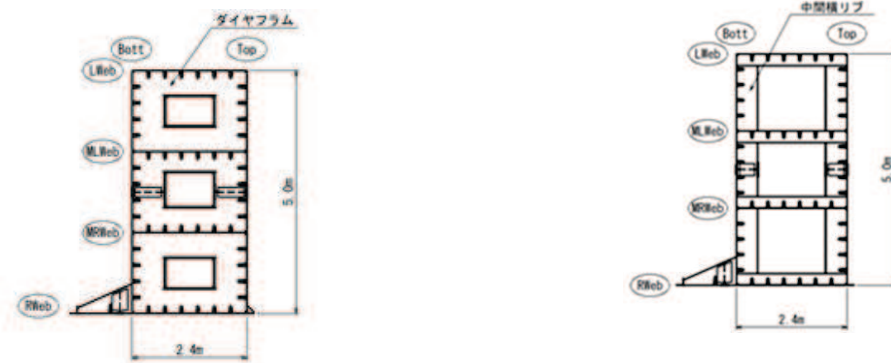
図 2.2-4(4) 鋼製遮水壁（鋼桁 1） 鋼桁構造図（底面図）
