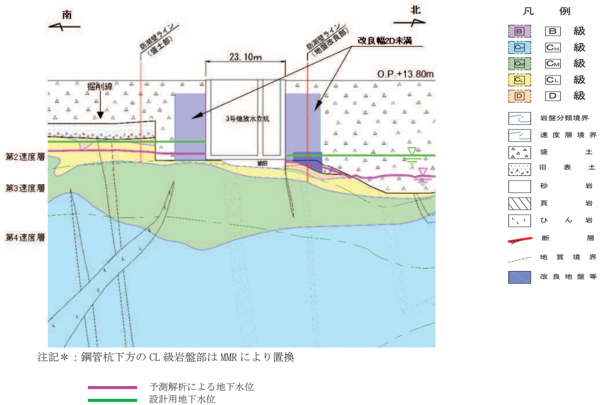
(3号機放水立坑横断方向(南北))
