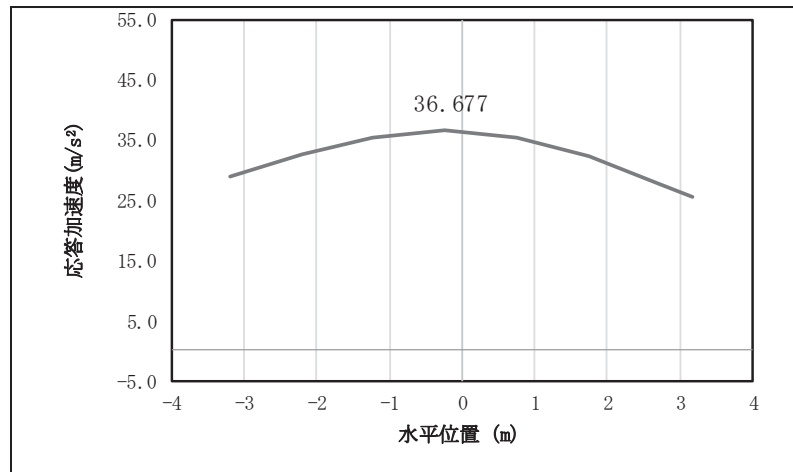
図 4.1-7(4) 扉体の水平応答震度分布（鋼製扉 2, S s-D 1 (---)）
