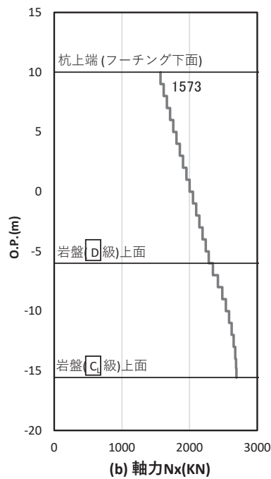
図 4.1-51 基礎地盤の支持性能照査時刻での軸力（押し込み時） (断面⑧, S d - D 2 (++) , t = 9.87s) 解析ケース①：基本ケース
