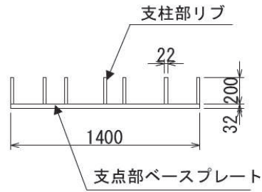
照査断面図
