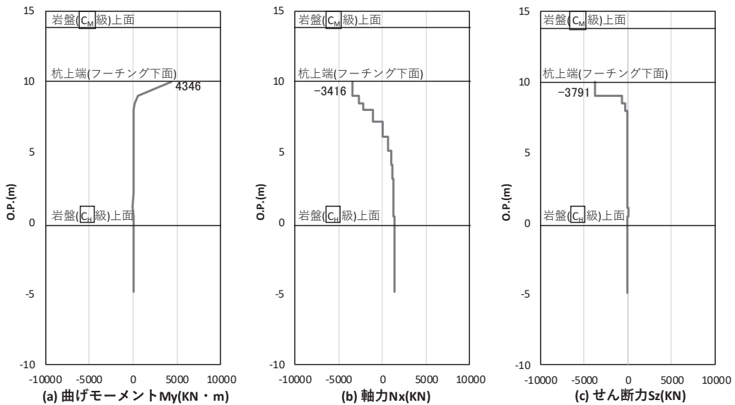
図 4.1-17 鋼管杭のせん断破壊に対する照査における照査時刻での断面力 (鋼製扉 2, S s - D 2 (- +), t = 20.42s) 解析ケース①: 基本ケース
