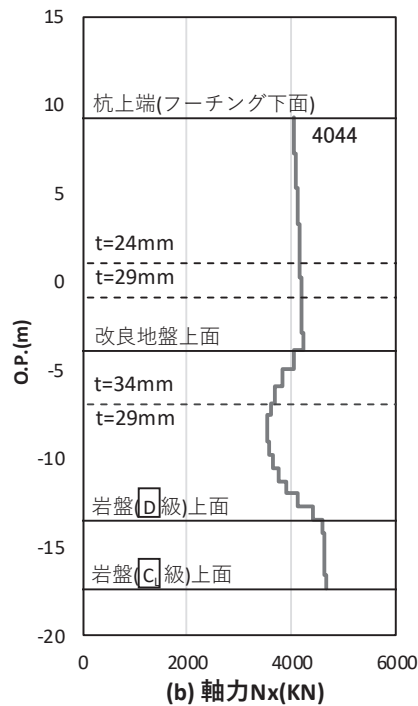
図 4.1-20 基礎地盤の支持性能照査時刻での軸力（押し込み時） （鋼製扉 3, S s - D 2 ( + + ) , t = 23.56s) 解析ケース②：地盤物性のばらつき (+ 1 \sigma ) を考慮した解析ケース
