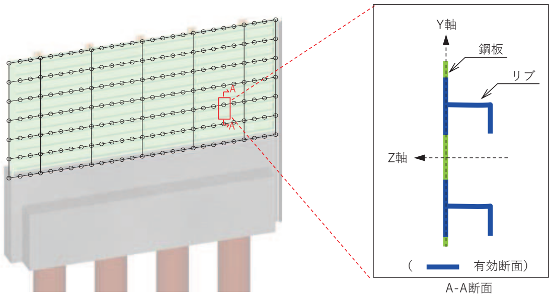
図 3.5-41 鋼板断面形状
