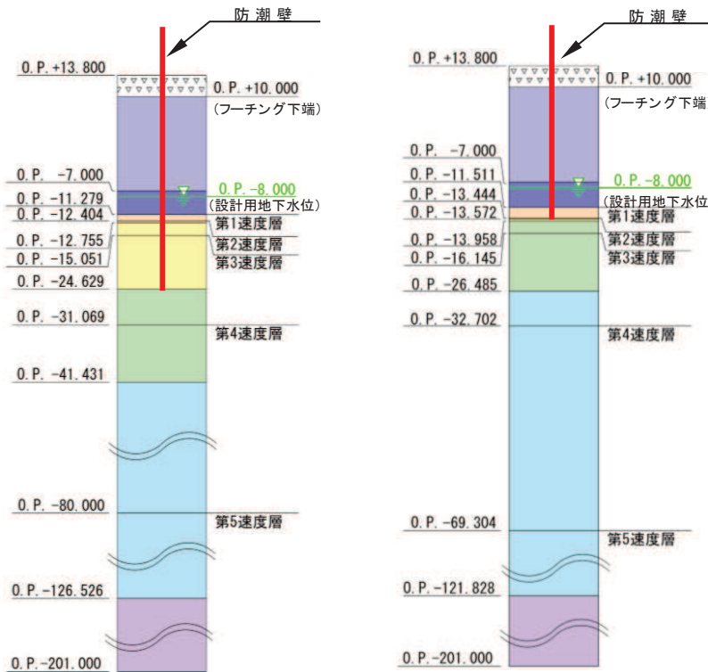
図 3.2-2(6) 評価対象断面の地層構成図 (鋼桁 6) (単位 : m)
