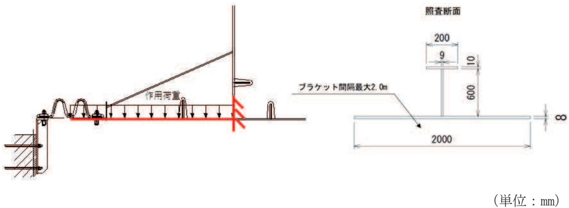
図 3.5-44 ブラケットの解析モデル図（断面図）
