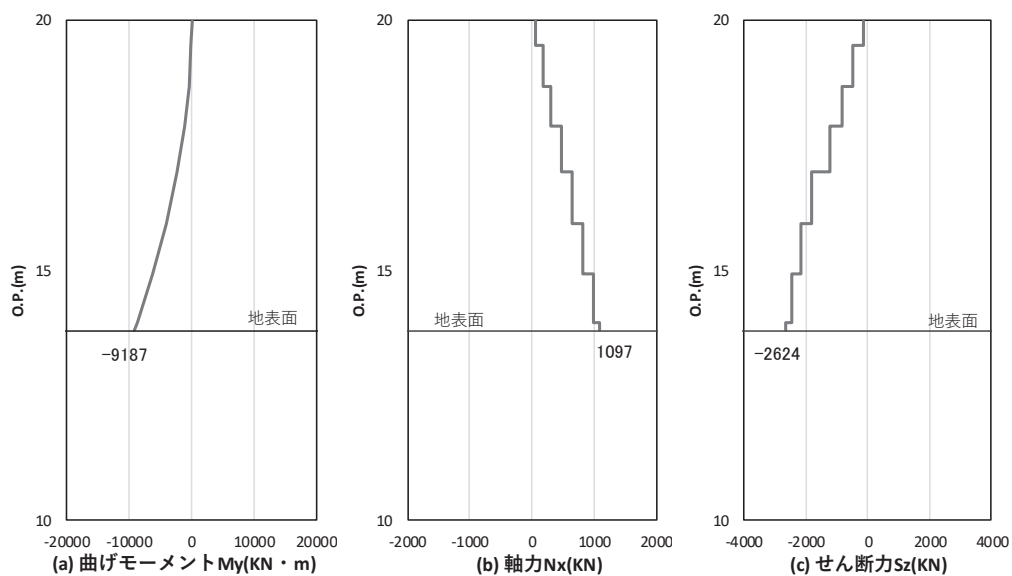
図 4.1-11(1) コンクリート及び鉄筋の曲げ・軸力系の破壊に対する照査における 最大曲げモーメント発生時刻での断面力 (鋼製扉 3, S_s - N_1 (-+) , t = 7.93\text{s} ) 解析ケース③: 地盤物性のばらつき ( -1\sigma ) を考慮した解析ケース
