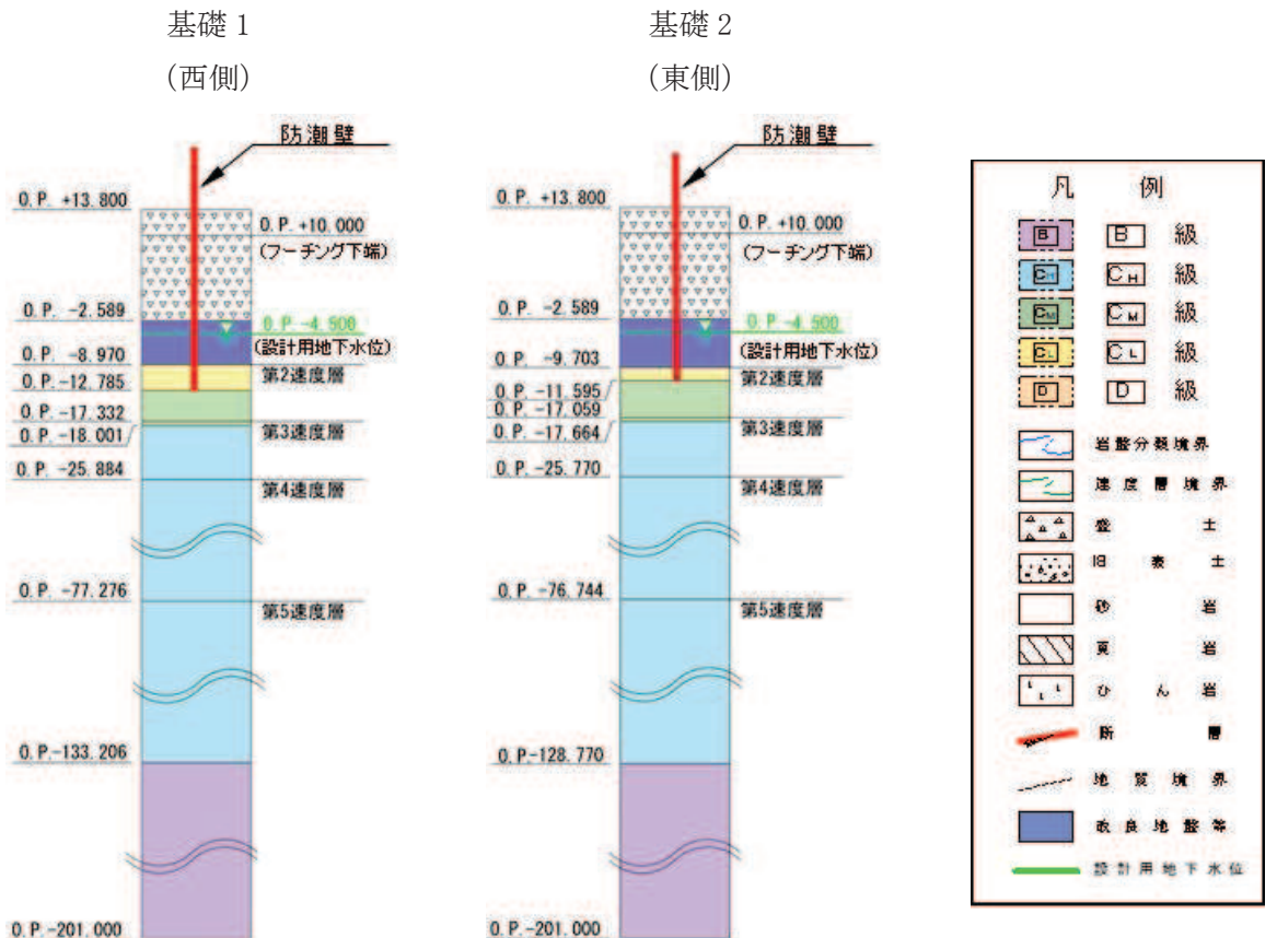
図 3.2-2(2) 評価対象断面の地層構成図 (鋼桁 2) (単位 : m)
