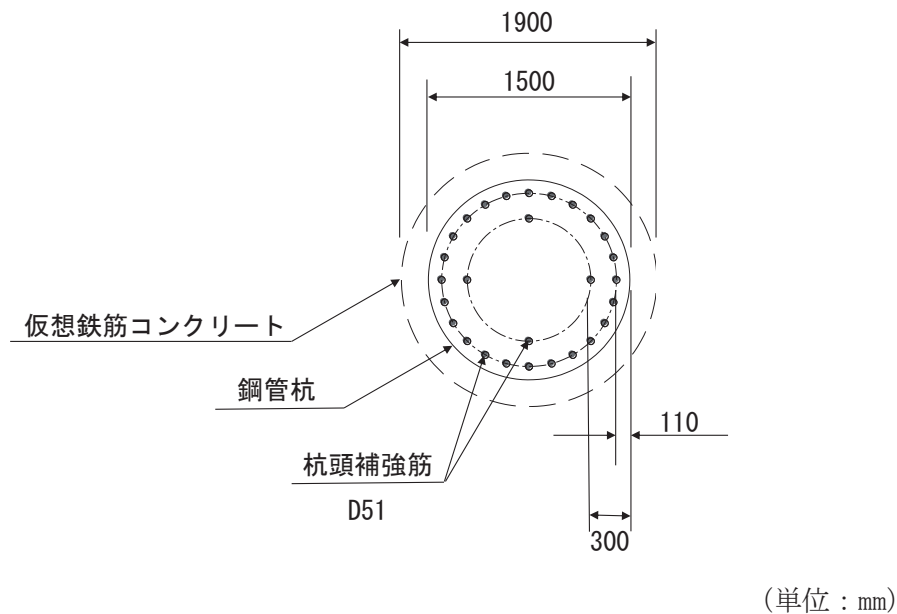
図 4.6-1 杭頭配筋概要図 (断面④の例)
