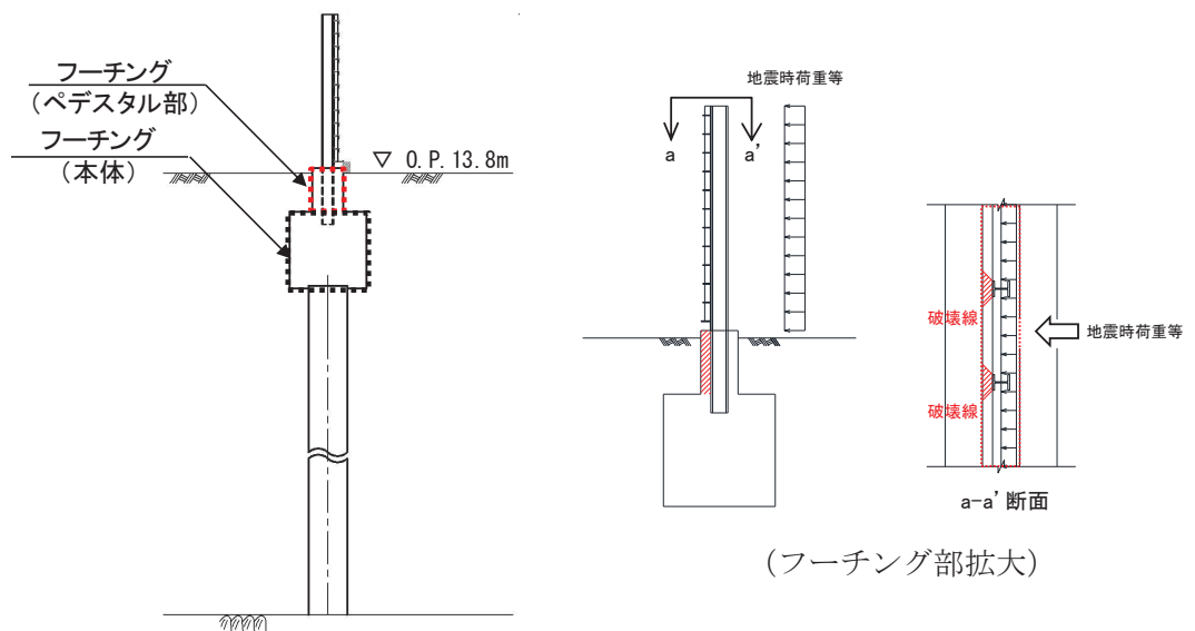
図 3.5-45 ペデスタル部に作用する荷重概念図
