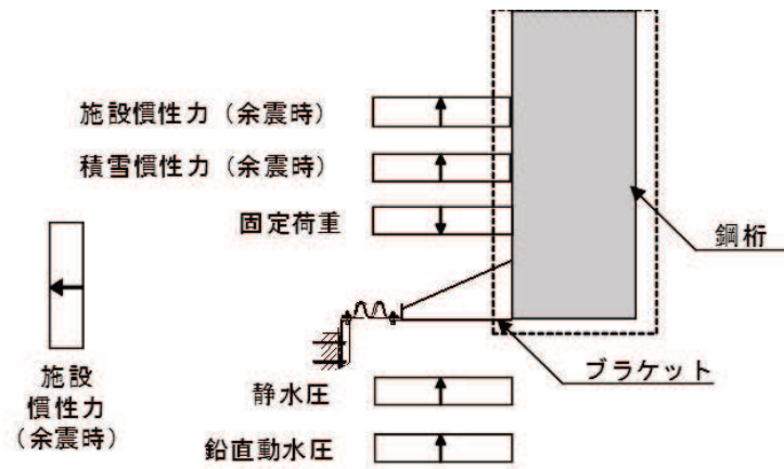
図 3.5-45 作用荷重図
