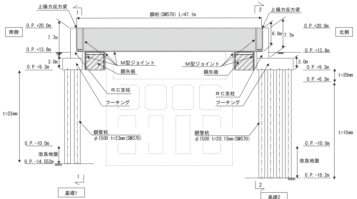
(正面図)
