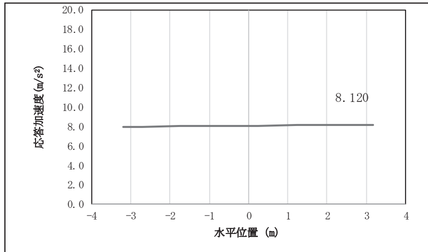
図 4.1-8(29) 扉体の鉛直応答震度分布 (鋼製扉 3, S s-D 3 (+ +))
