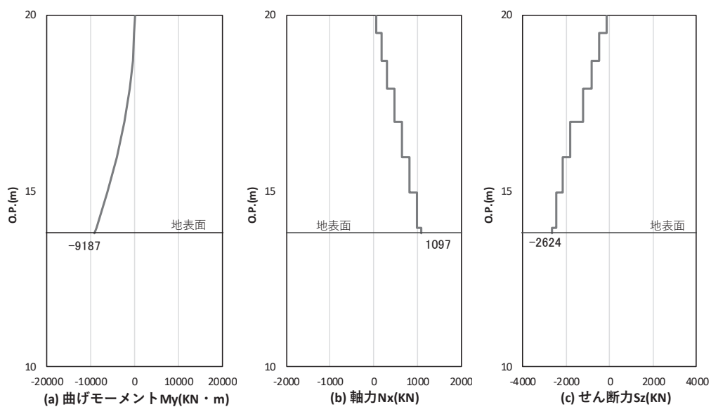
図 4.1-11(2) コンクリート及び鉄筋のせん断破壊に対する照査における発生時刻での断面力 (鋼製扉 3, S_s - N_1 (-+) , t = 7.93\text{s} ) 解析ケース③: 地盤物性のばらつき ( -1\sigma ) を考慮した解析ケース
