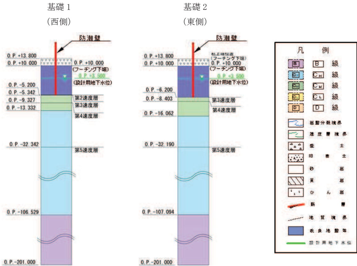
図 3.2-2(3) 評価対象断面の地層構成図 (鋼桁 3) (単位 : m)
