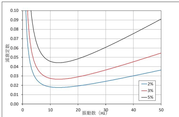
図 3.5-17 設定した Rayleigh 減衰 (断面⑥) _減衰 2%~5%
