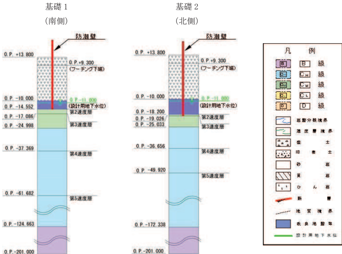
図 3.2-2(4) 評価対象断面の地層構成図 (鋼桁 4) (単位 : m)
