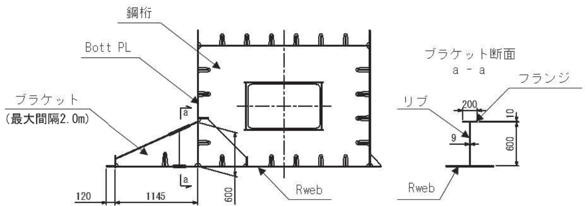
図 2.2-4(5) 鋼製遮水壁（鋼桁 1） 鋼桁構造図（断面図）
