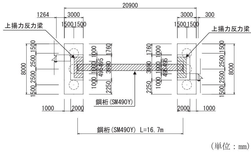
図 2.2-5 (2) 鋼製遮水壁 (鋼桁 2) 平面図
