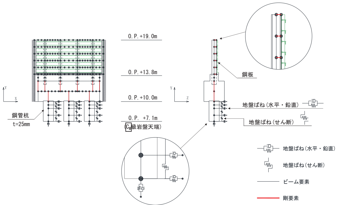
図 3.5-28 解析モデル (断面⑥)
