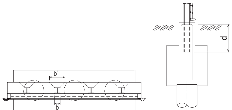
図 3.5-46 支圧に関する寸法
