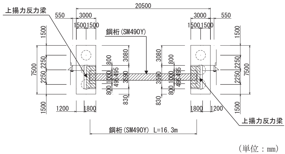
図 2.2-9(2) 鋼製遮水壁（鋼桁 6） 平面図
