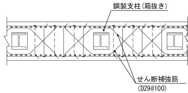
図 3.4-6 算定に用いる寸法位置
