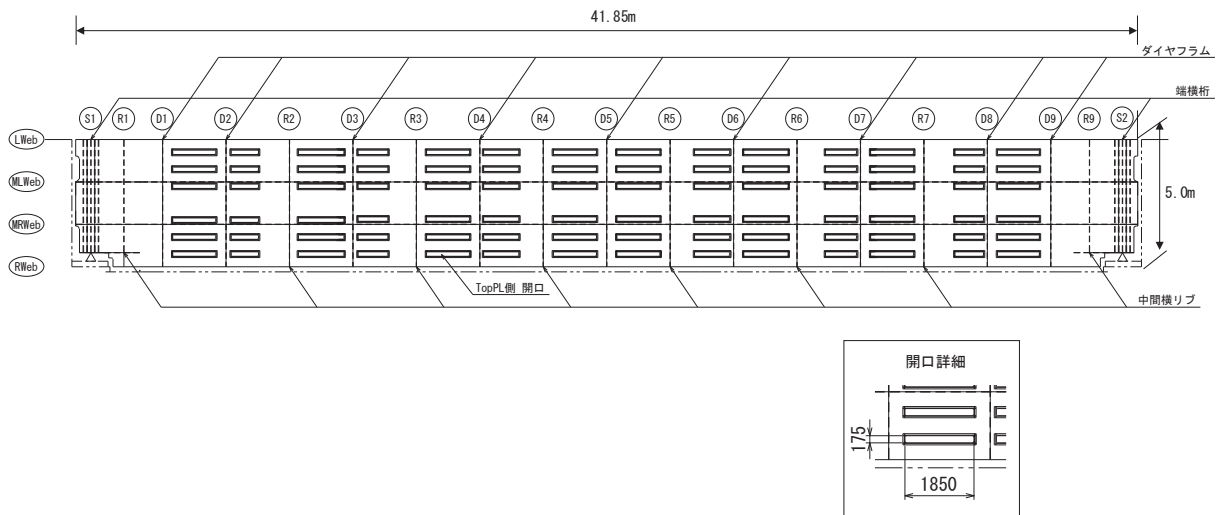
図 2.2-4(2) 鋼製遮水壁（鋼桁1） 平面図
