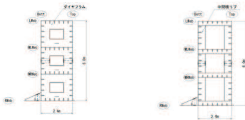
図 2.2-7(4) 鋼製遮水壁（鋼桁 4） 鋼桁構造図（底面図）
