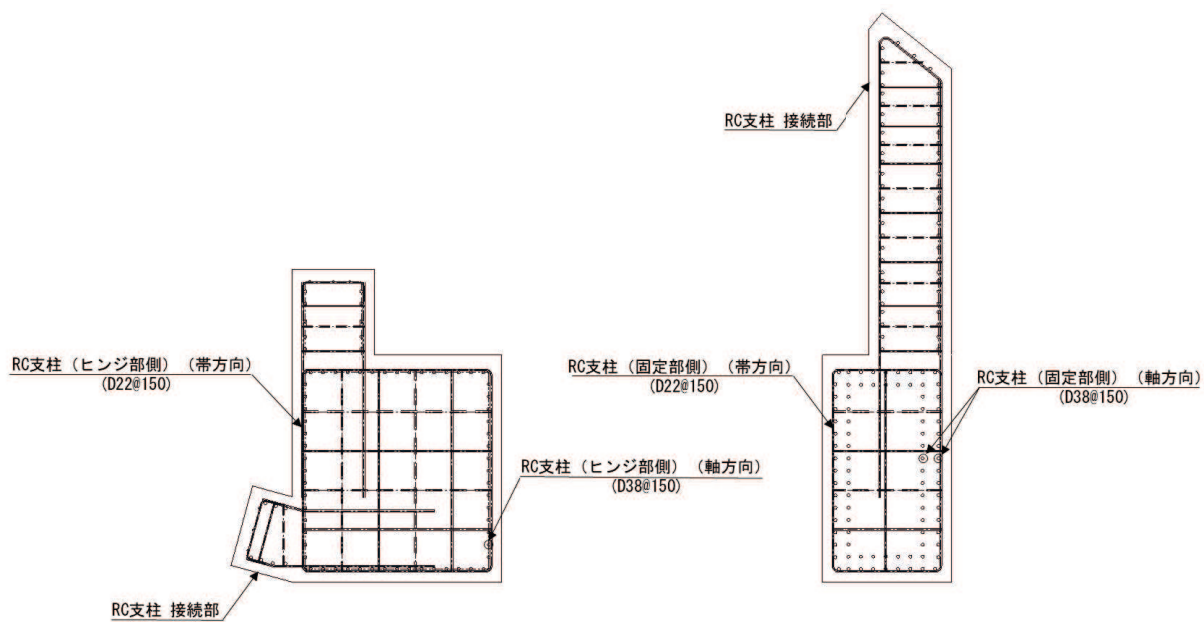
(3-3 断面)
