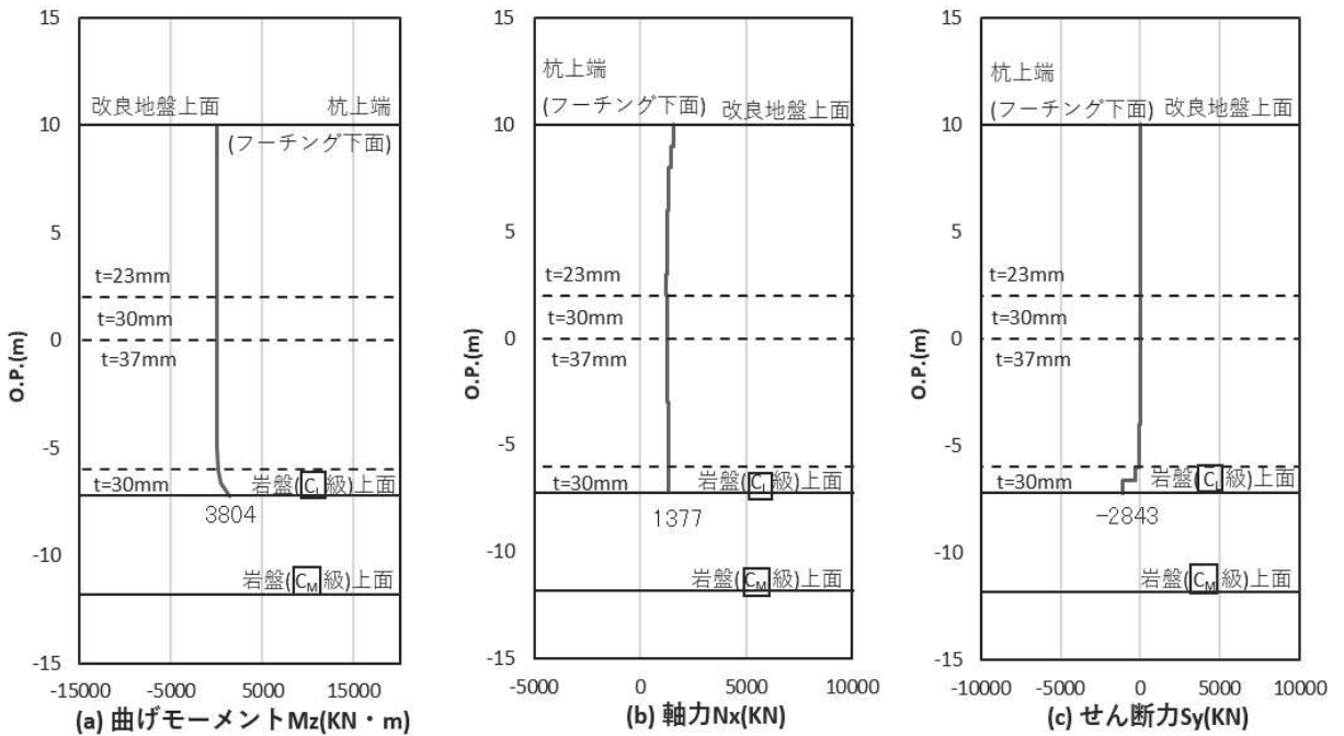
図 4.1-43(2) 鋼管杭の曲げ・軸力系の破壊に対する照査における照査時刻での断面力 (鋼桁 5 (地盤改良 (改良幅 2D 未満) 考慮) : 基礎 2, S s - N 1 ( + + ) , 桁軸直交方向加振時, t = 7.66s ) 解析ケース① : 基本ケース
