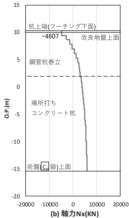
図 4.1-50(2) 基礎地盤の支持性能照査時刻での軸力（引き抜き） (鋼桁 1：基礎 2, S s - D 2 (++) , 桁軸方向加振時, t = 23.72s) 解析ケース③：地盤物性のばらつき (-1σ) を考慮した解析ケース
