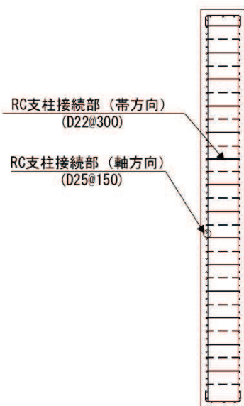
(2-2 断面)
