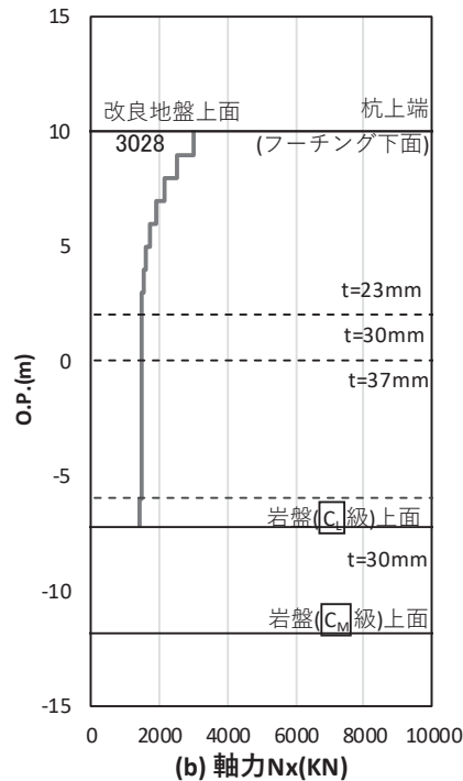
図 4.1-63(2) 基礎地盤の支持性能照査時刻での軸力（押し込み） （鋼桁 5（地盤改良（改良幅 2D 未満）考慮）：基礎 1， S s - D 2（++），桁軸直交方向加振時， t = 20.49s ） 解析ケース①：地盤物性のばらつき（ -1\sigma ）を考慮した解析ケース
