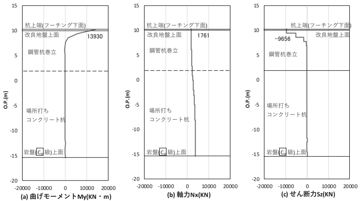
図 4.1-33(3) 場所打ちコンクリート杭の曲げ・軸力系の破壊に対する照査における 最大曲げモーメント発生時刻での断面力 (鋼桁 1 : 基礎 2, S s - D 2 ( - + ) , 桁軸方向加振時, t = 40.41s) 解析ケース③ : 地盤物性のばらつき ( - 1 \sigma ) を考慮した解析ケース
