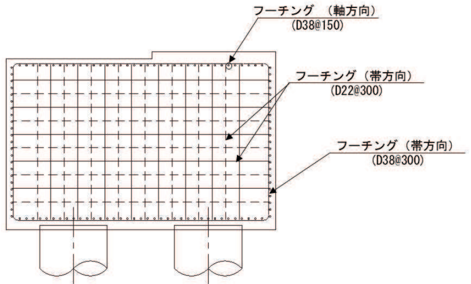
(1-1 断面)
