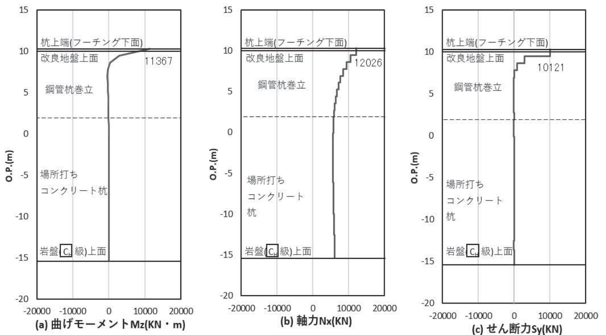
図 4.1-33(4) 場所打ちコンクリート杭の曲げ・軸力系の破壊に対する照査における 最大曲げモーメント発生時刻での断面力 (鋼桁 1 : 基礎 2, S s - D 1 ( + - ) , 桁軸直交方向加振時, t = 18.14s) 解析ケース③ : 地盤物性のばらつき ( - 1 \sigma ) を考慮した解析ケース
