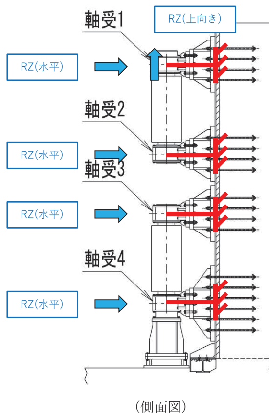
図 3.8-7 ヒンジ水平荷重支承部に伝達する荷重と評価用モデルのイメージ図
