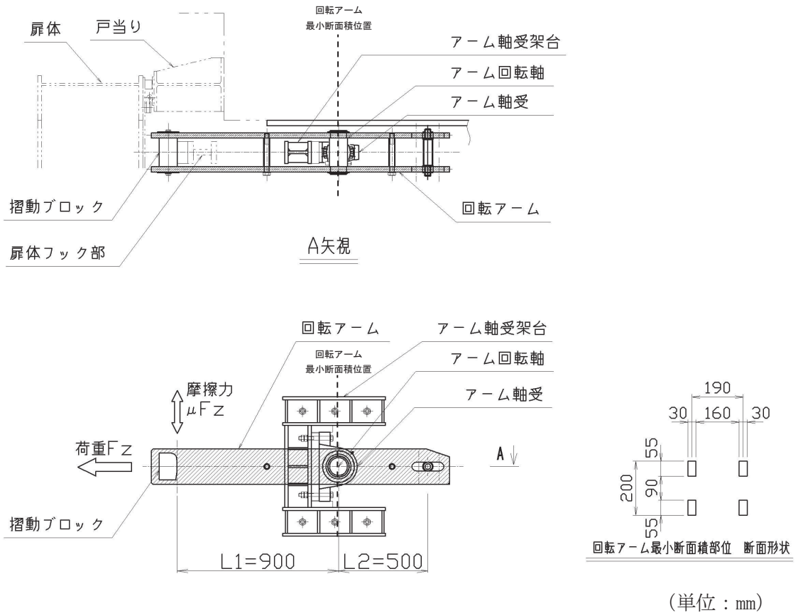
図 3.8-31 回転アームの概要図及び計算モデルの概念図
