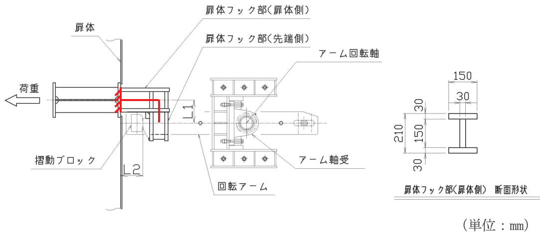
図 3.8-29 扉体フック部（扉体側）構造概要及び計算モデル概念図
