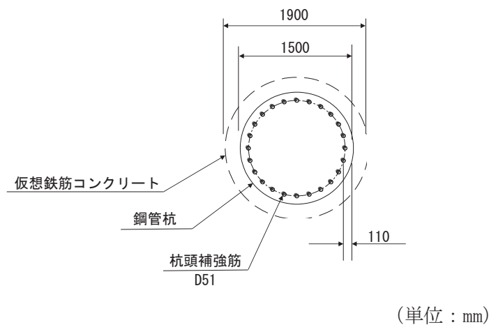
図3.8-50 仮想鉄筋コンクリート断面概念図
