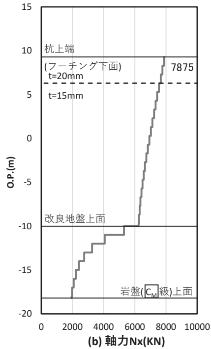
図 4.1-55(3) 基礎地盤の支持性能照査時刻での軸力（押し込み） (鋼桁 4 : 基礎 2, S s - N 1 ( - + ) , 桁軸方向加振時, t = 7.88s) 解析ケース① : 基本ケース
