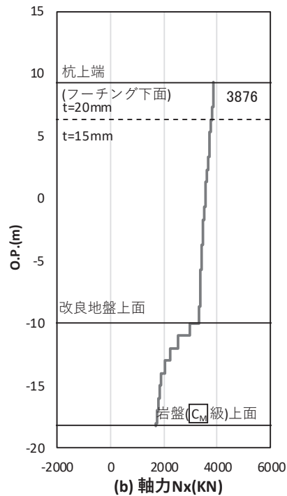
図 4.1-58(2) 基礎地盤の支持性能照査時刻での軸力（押し込み） (鋼桁 4 : 基礎 2, S s - N 1 ( - + ) , 桁軸直交方向加振時, t = 7.88s) 解析ケース① : 基本ケース
