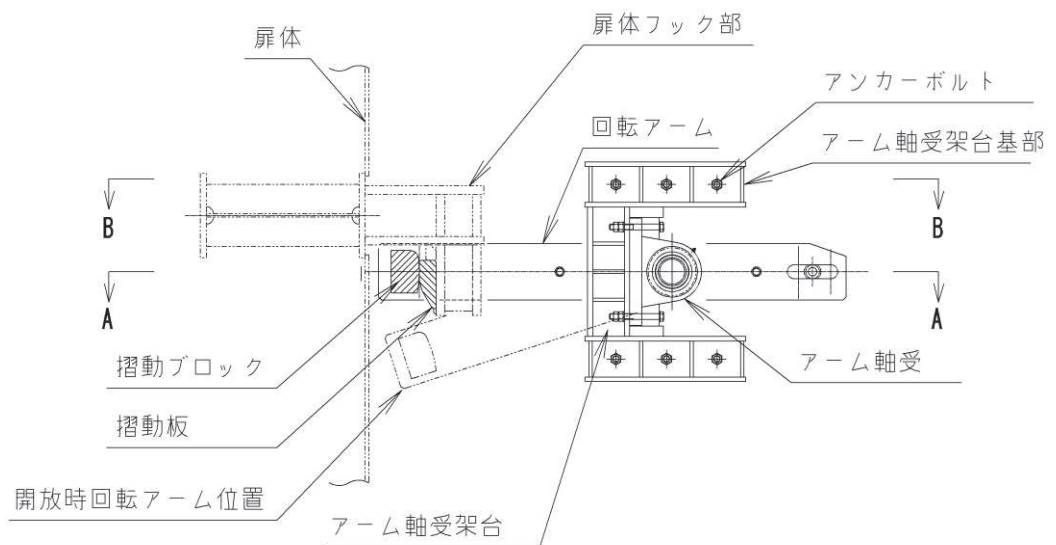
(側面図)
