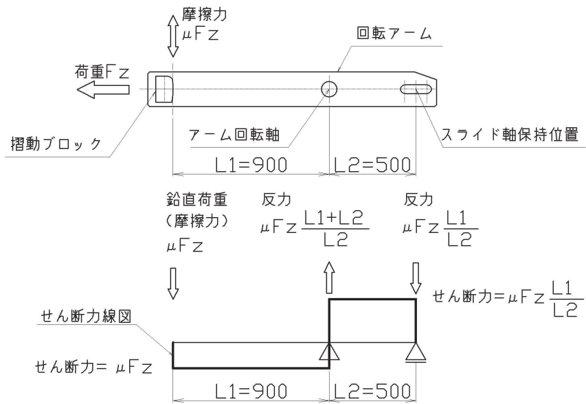
図 3.8-32 応力集中係数の計算モデル概要図
