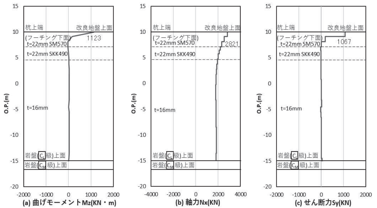
図 4.1-33(2) 鋼管杭の曲げ・軸力系の破壊に対する照査における照査時刻での断面力 (鋼桁 1 : 基礎 1, S s - D 1 (+), 桁軸直交方向加振時, t = 25.50s ) 解析ケース③ : 地盤物性のばらつき ( -1\sigma ) を考慮した解析ケース
