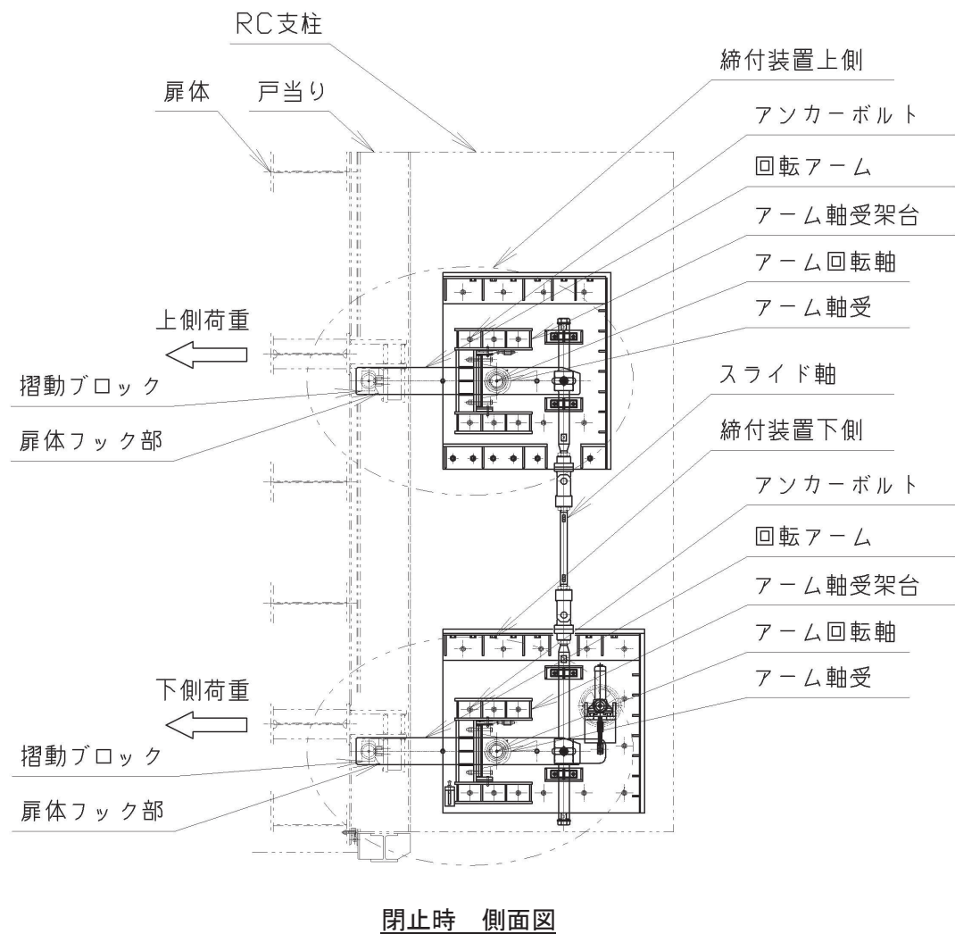
図 3.8-26 締付装置側面 概要図
