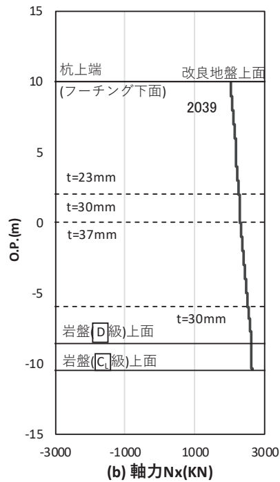
図 4.1-63(1) 基礎地盤の支持性能照査時刻での軸力（押し込み） （鋼桁 5（地盤改良（改良幅 2D 未満）考慮）：基礎 2， S s - D 2（-+），桁軸方向加振時， t = 23.56s ） 解析ケース③：地盤物性のばらつき（ -1\sigma ）を考慮した解析ケース
