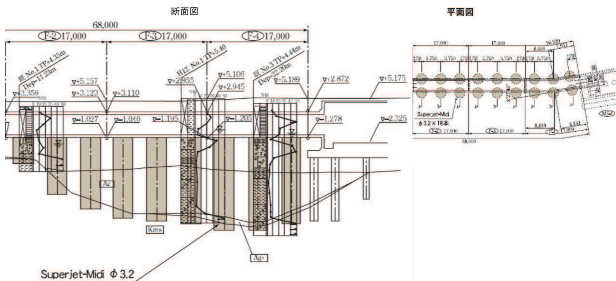
図 6.4-23 施工概要図
