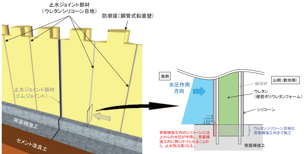
(ウレタンシリコン目地の下部詳細)
