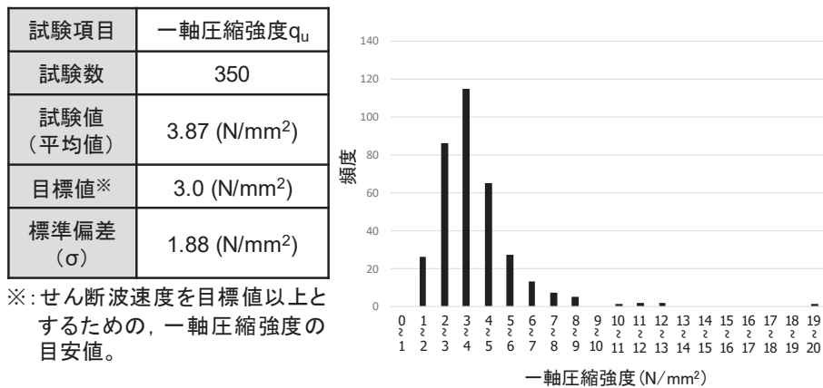
図 6.4-8 既設改良地盤における一軸圧縮強度試験結果 (参考値)
