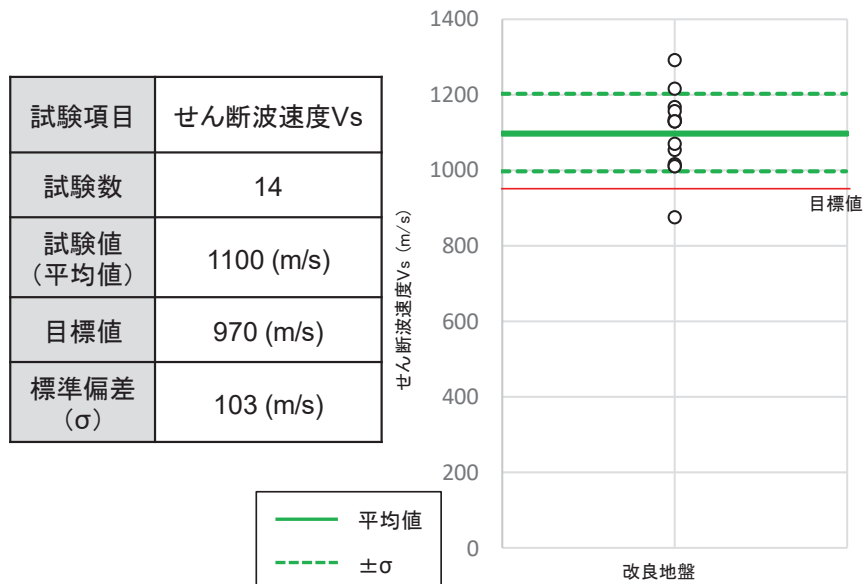
図 6.4-7 既設地盤改良における品質確認結果 (PS 検層)
