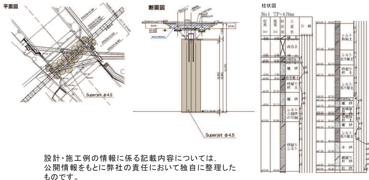
図 6.4-20 施工概要図
