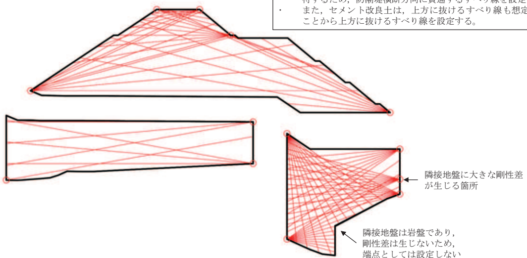
図 12-4 想定すべり線のイメージ（防潮堤（盛土堤防））
