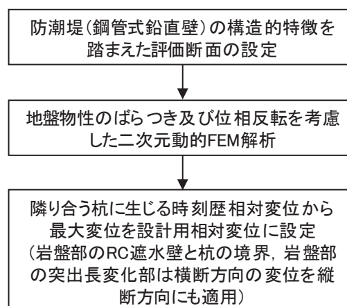
図 6.1.6-19 地震時の縦断方向の相対変位算出フロー
