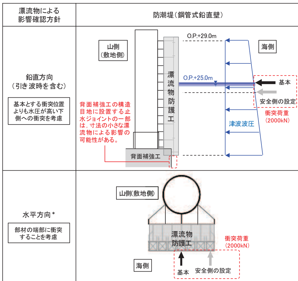
図 2.3-1 漂流物による影響確認方針
