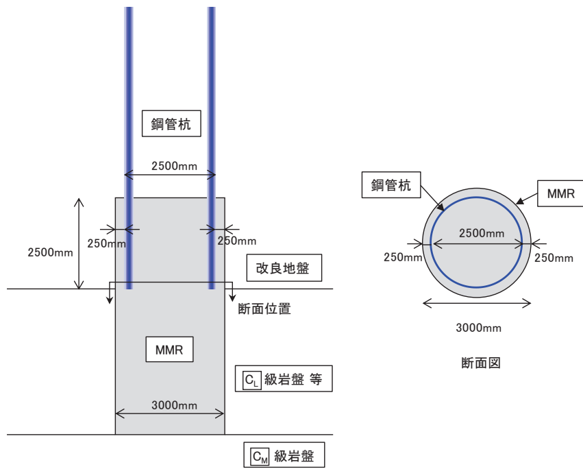
図 13.3-3 鋼管杭と MMR の接合詳細
