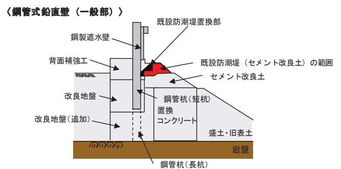
図 7.2-1 既設防潮堤の概要
