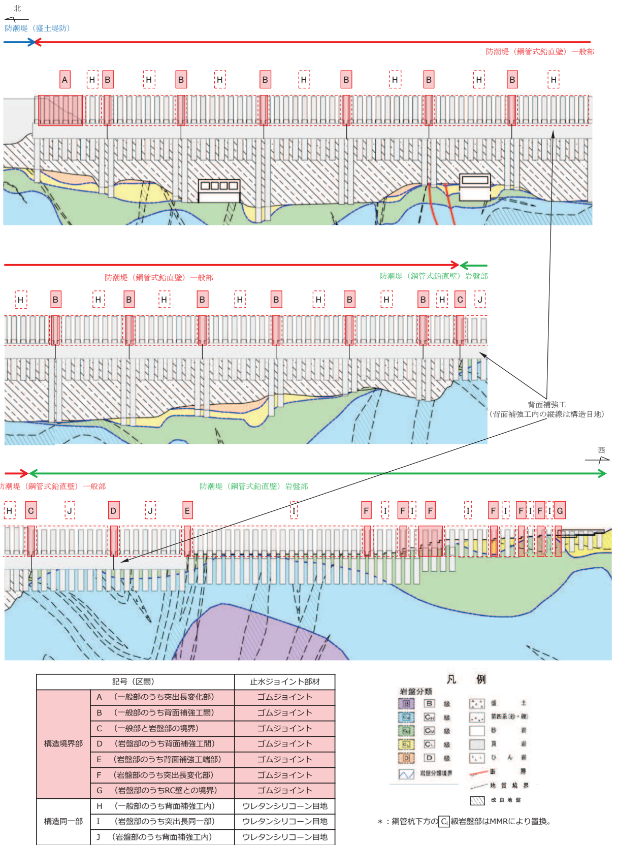
図 6.1.5-2 止水ジョイント部材の設置箇所 (防潮堤縦断面図)
