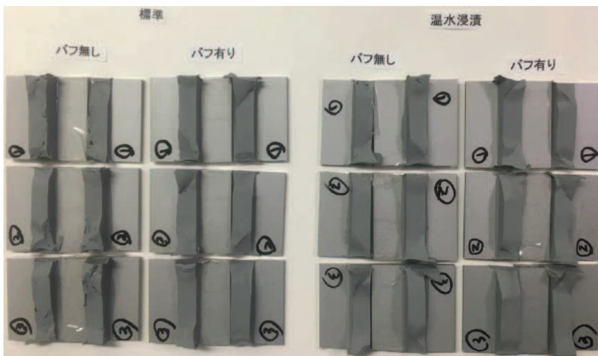
図 6.1.5-27(4) 接着性（付着性）試験結果（40 \mu mメタリック色-1） （いずれの試験結果もCFすなわち、シリコン材で切れているため、左右どちらにも灰色のシリコン材が残っていることが確認される）
