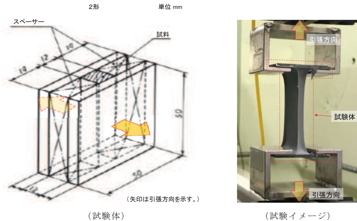
図 6.1.5-26 試験概要
