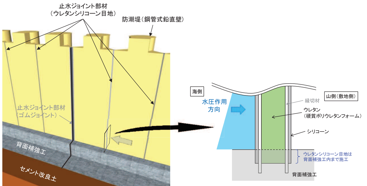
(ウレタンシリコーン目地の下部詳細)
