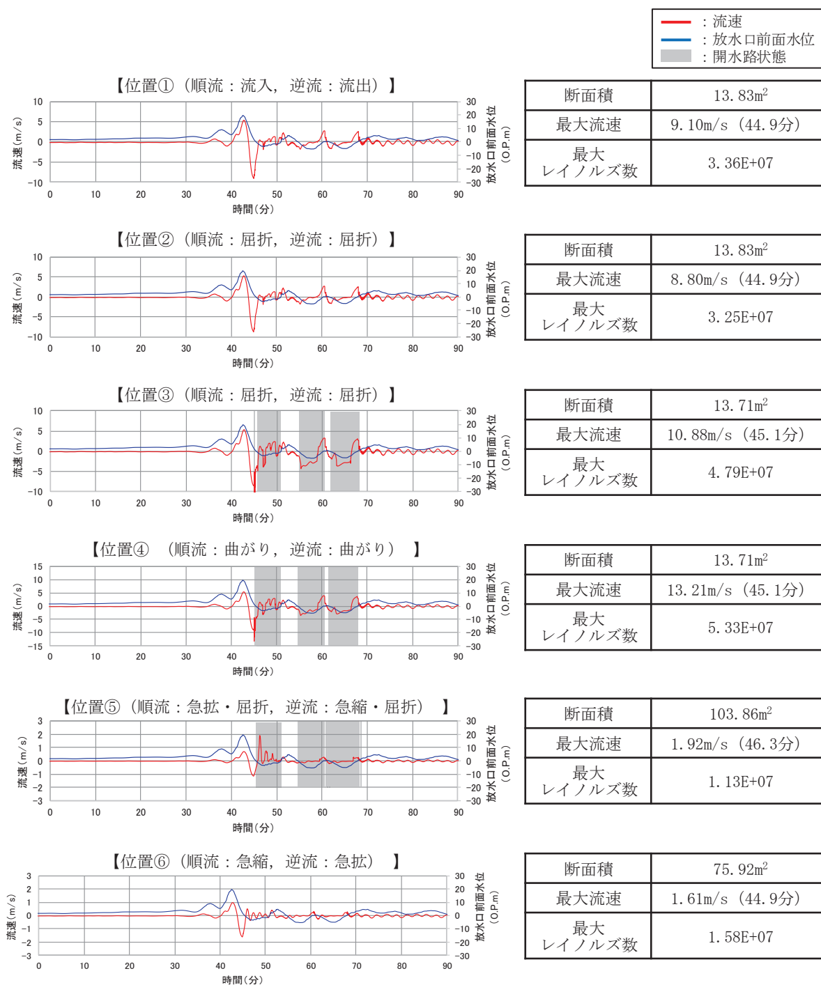
図 1.4-19 (8) 流速の経時変化 (第3号機放水路 (1))
