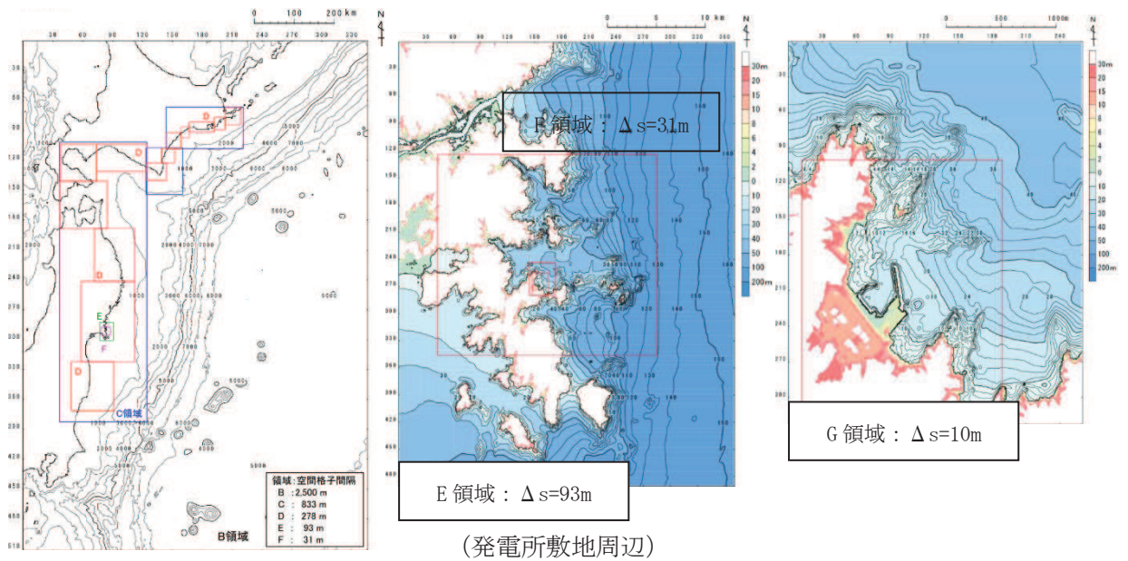
図 1.2-1 数値シミュレーションにおける解析モデル
