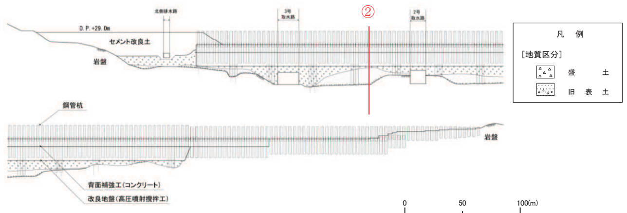
図4(1) 地質断面図(①-①'断面)
