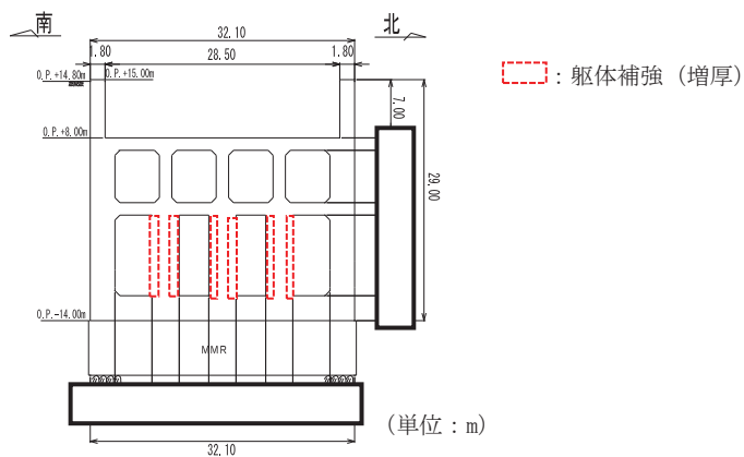
図 2-3(3) 第 3 号機海水ポンプ室断面図 (B-B)
