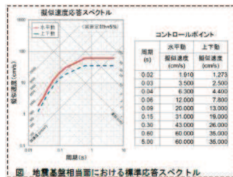
図 9 地震基盤相当面における標準応答スペクトル
