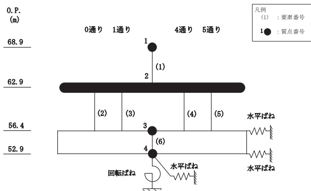
図2-14 せん断スケルトンカーブ上の最大応答値 (S s - F 3, EW 方向)
