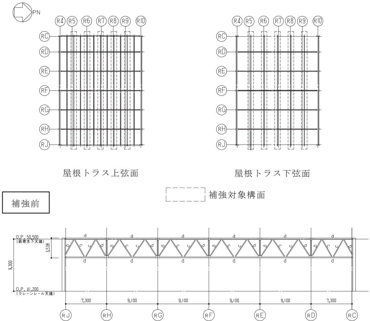
図 2-2 サブトラス各構面軸組図（補強前）
