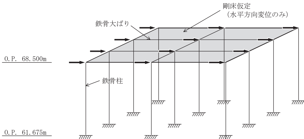
図 2-3 フレームの静的漸増解析の概要
