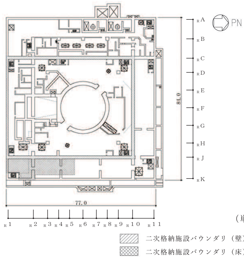
図 3-4 原子炉建屋原子炉棟（二次格納施設）の範囲の平面図 (B1F, O.P. 6.0m)
