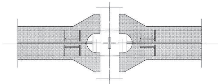
A-A section
