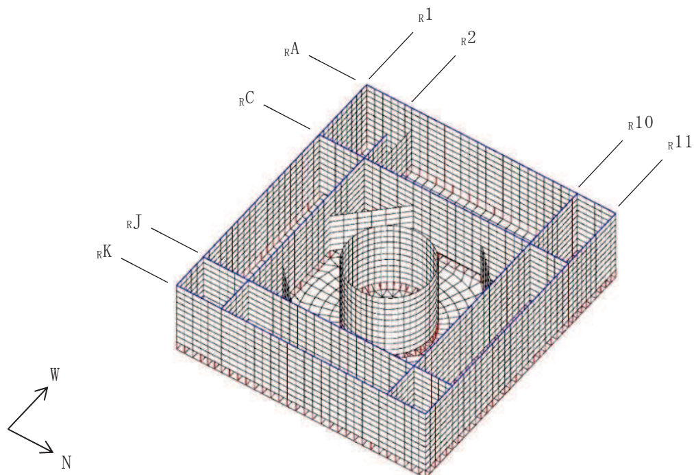
図 4-1 耐震壁配置状況
