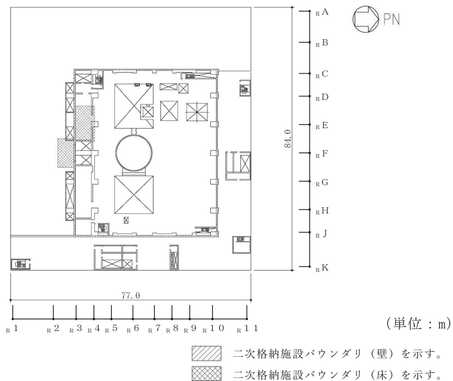
図 3-7 原子炉建屋原子炉棟（二次格納施設）の範囲の平面図 (3F, O.P. 33.2m)
