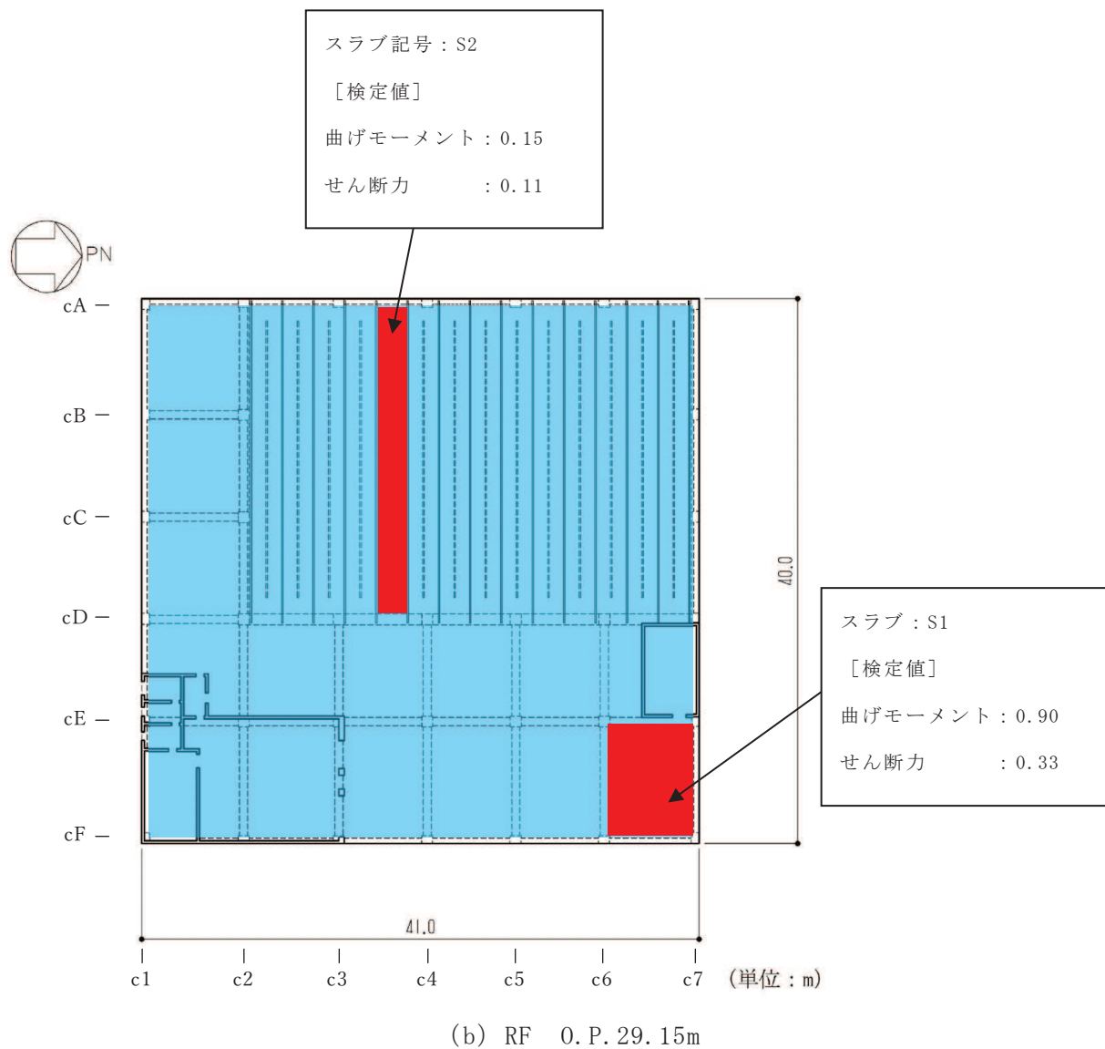
図 3-4(2) 断面の評価位置及び評価結果 (2/2)
