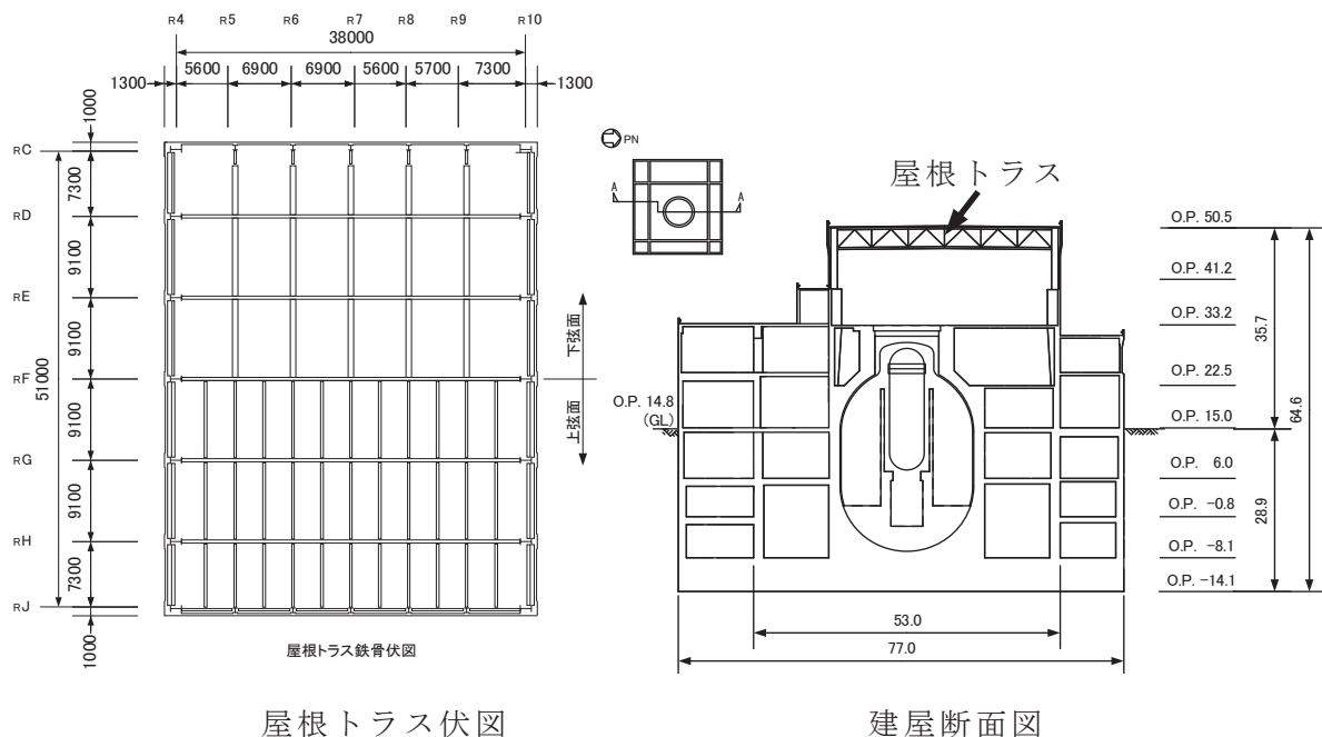
図2-1 原子炉建屋屋根トラスの概要
