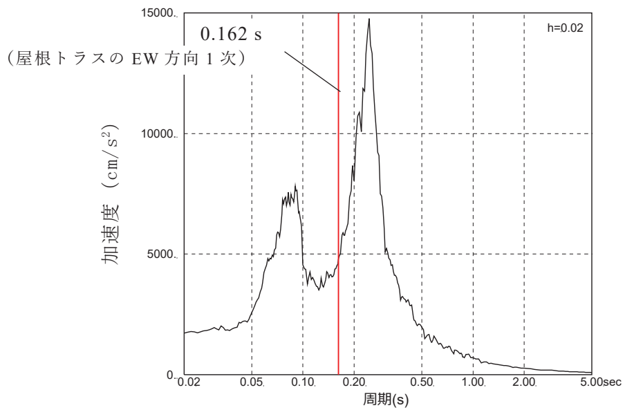
図 2-4 固有周期と入力地震動の加速度応答スペクトルの関係 (EW 方向)
