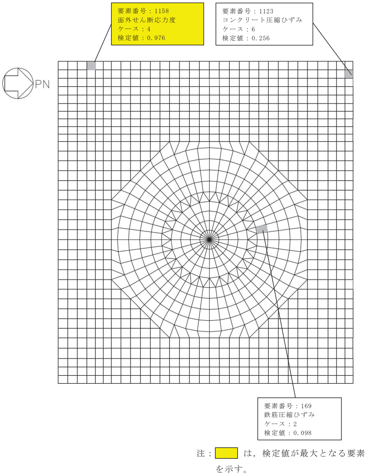
図 2-2 断面力ごとの検定値が最大となる要素及び断面の評価結果
