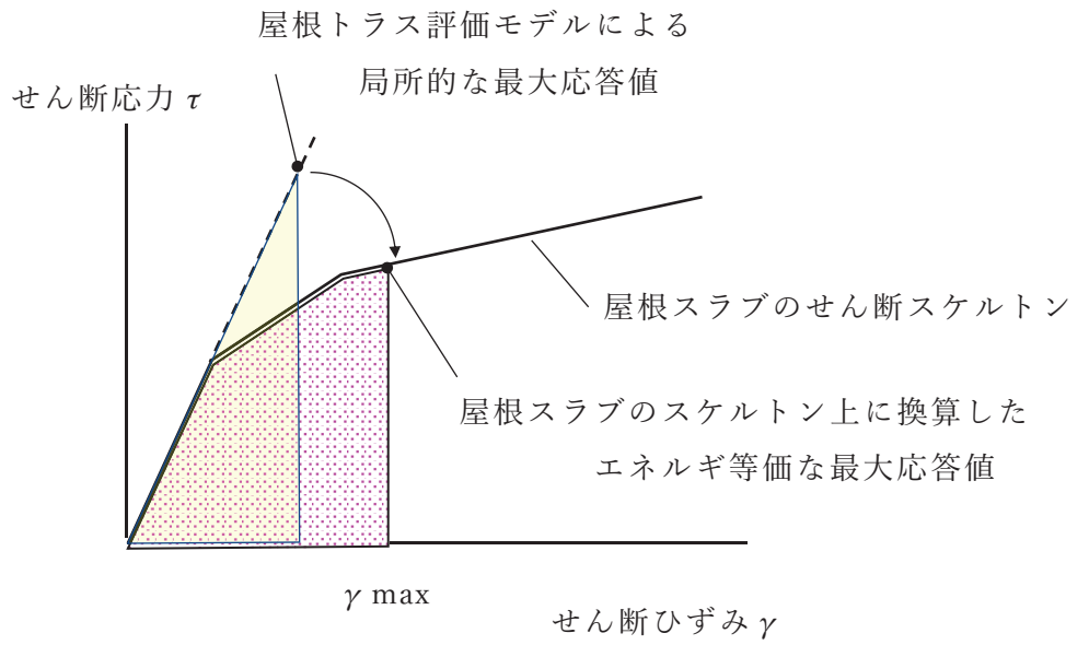
図 4-5 エネルギー一定則に基づく屋根スラブのせん断ひずみの評価方法
