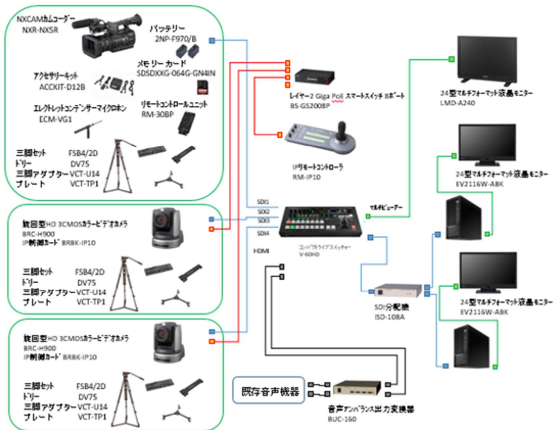
(13F A 会議室機材構成図)
