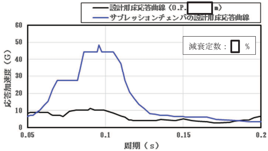
別図 2-13 今回工認の耐震評価に適用した設計用床応答曲線 (O.P. [redacted] m) とサプレッションチェンバの設計用床応答曲線との比較結果
