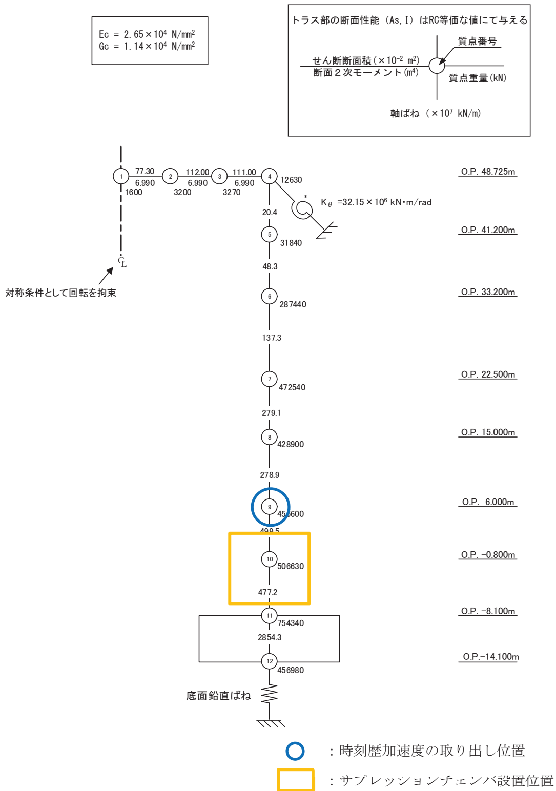
図7 原子炉建屋の地震応答解析モデルにおける時刻歴加速度の取り出し位置 (RHR-010, UD方向)
