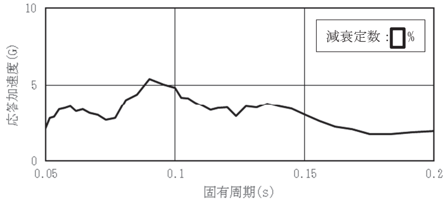
図 11 床応答スペクトル (1/3) (RHR-010, 基準地震動 S s-D 2, 原子炉建屋: 0.P. [ ] m, NS 方向)
