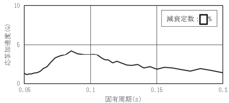
図 11 床応答スペクトル (3/3) (RHR-010, 基準地震動 S s-D 2, 原子炉建屋: 0.P. [ ] m, UD 方向)
