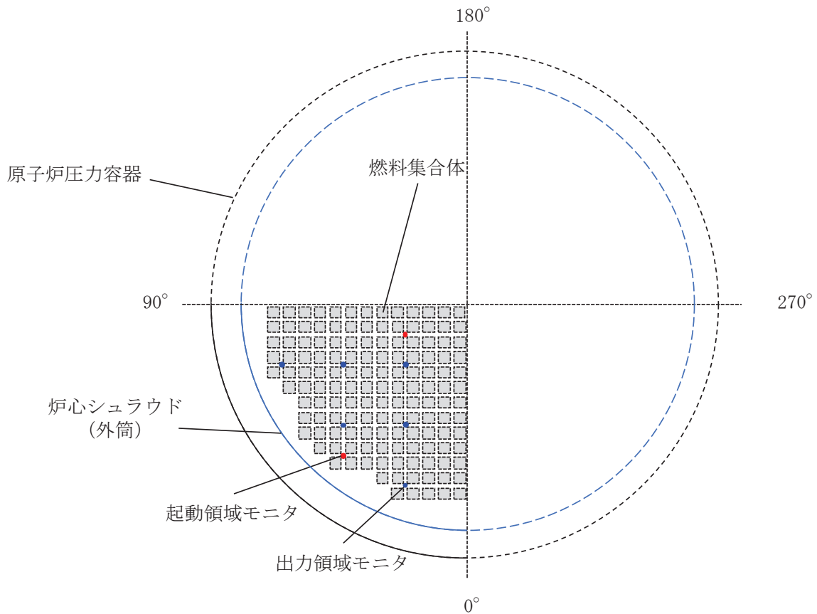
別図 1 炉内計測装置，燃料集合体及び炉心シュラウドの配置イメージ図
