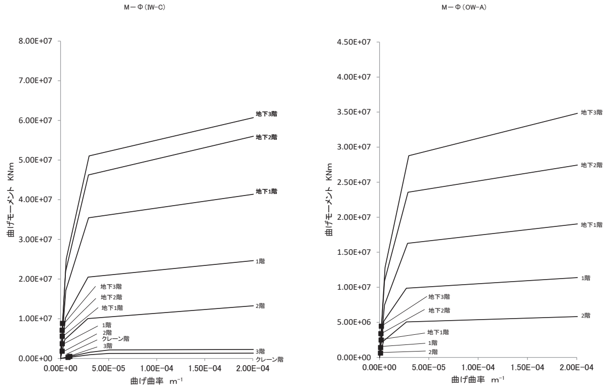
図 2-51 原子炉建屋 曲げスkeleton カーブ 上の最大応答値(NS 方向) 4.7 地震 (2/2)
