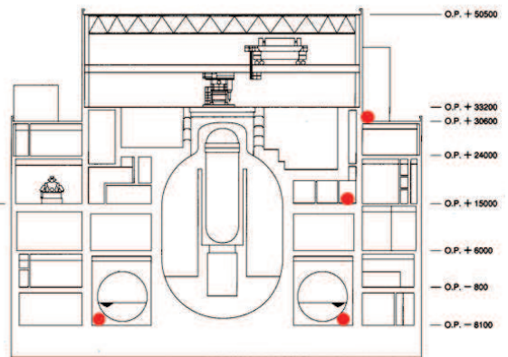
B-B 断面
