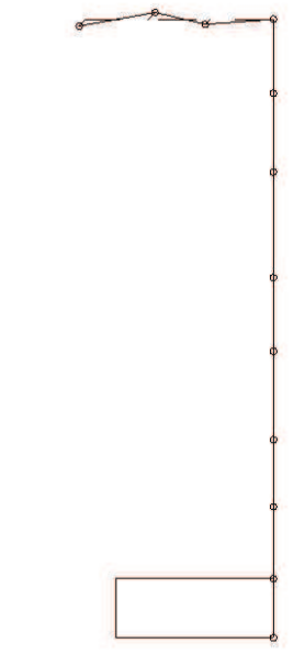
図 3-25 第 3 号機原子炉建屋 固有振動モード (鉛直方向)
