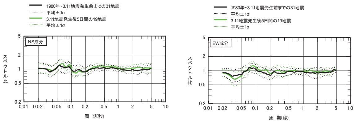
図 2.5-3 スペクトル比 (女川1号機原子炉建屋直下/自由地盤)
