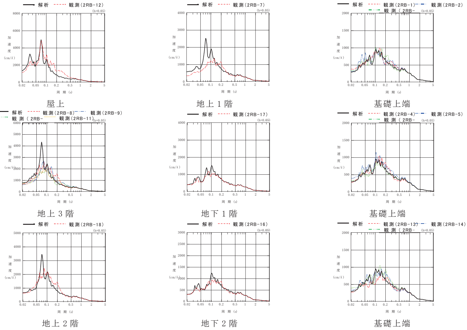
図 2-17 原子炉建屋 加速度応答スペクトルの比較 (3.11 地震 鉛直方向)
