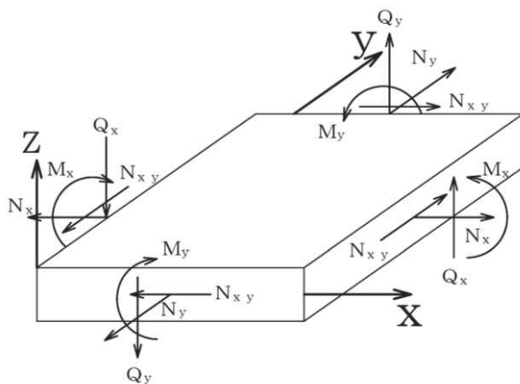
図 6-8 シェル要素における断面力の方向
