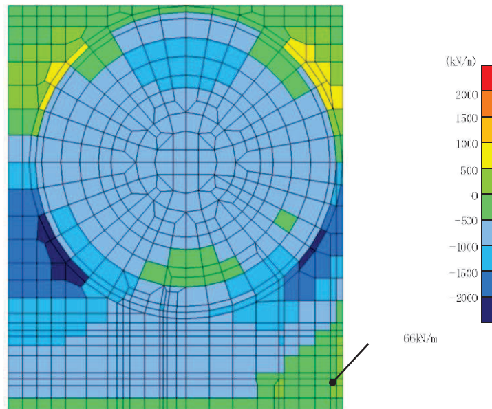
図 6-16(4) 曲げ・軸力系の破壊に対する照査値最大時の断面力分布図 (軸力 ( \text{kN/m} ) : N_y ) (解析ケース②, S_s - D 2 (++) , t=6.86\text{s} , 南北)
