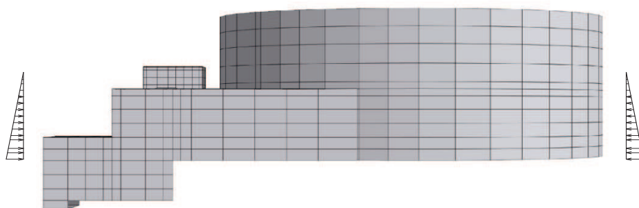
図4-16(1) 静止土圧の荷重概念図（しゃへい壁，バルブ室及び連絡ダクト）
