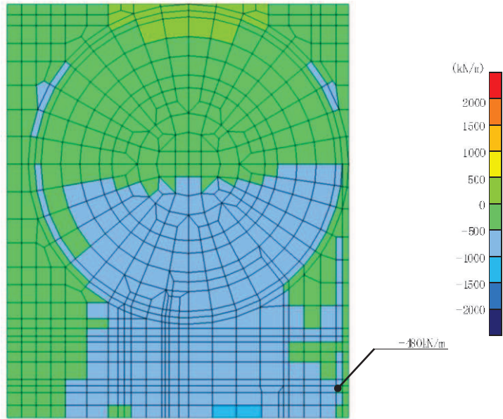
図 6-16(3) 曲げ・軸力系の破壊に対する照査値最大時の断面力分布図 (軸力 ( \text{kN/m} ) : N_x ) (解析ケース②, S_s - D 2 (++) , t=6.86\text{s} , 南北)
